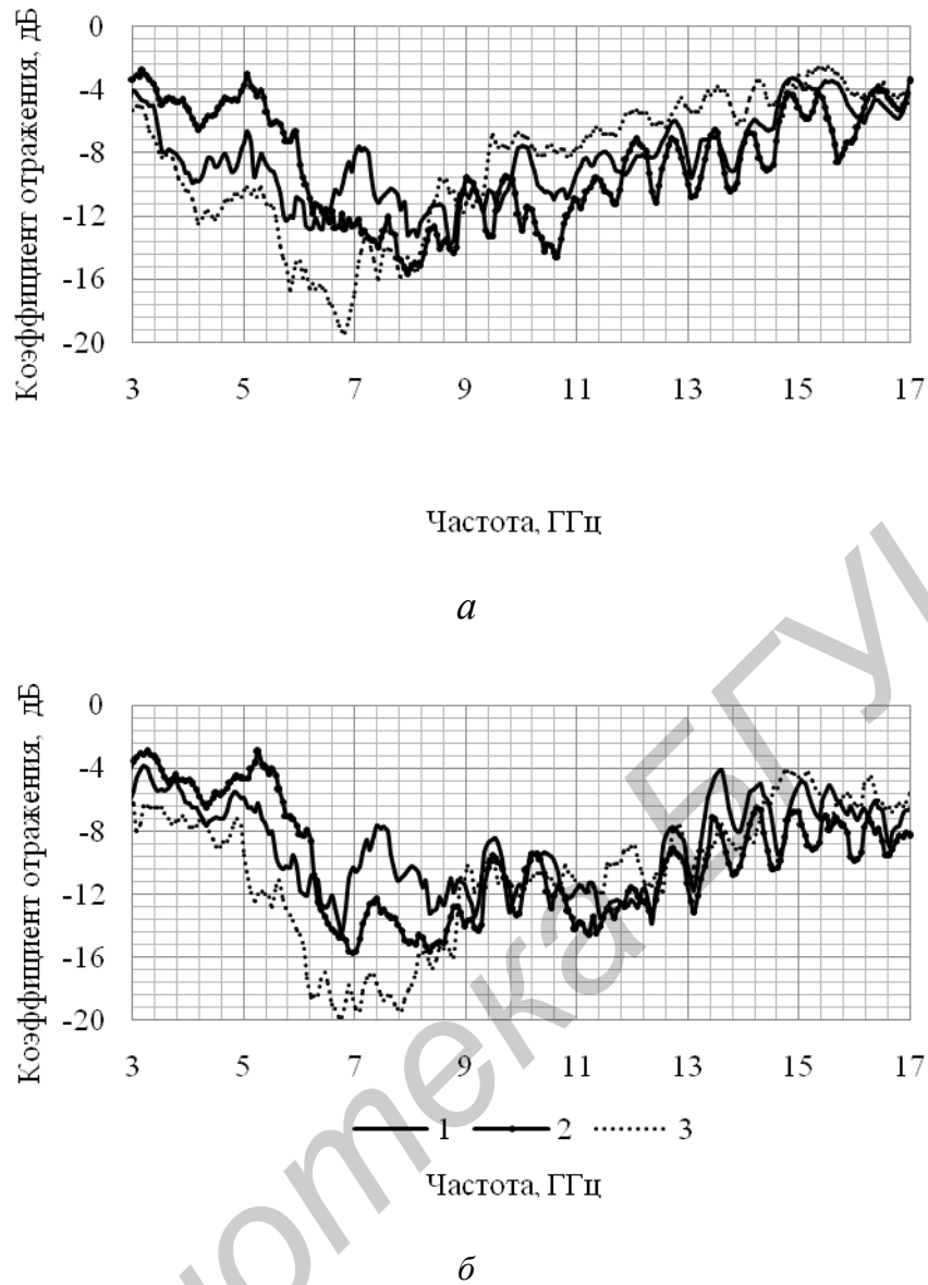
Рис. 3. Частотные зависимости коэффициента отражения ( a ) и коэффициента отражения с металлом ( b ) конструкции экрана ЭМИ в диапазоне частот 3–17 ГГц, выполненной на основе керамзита, содержащего водные растворы хлорида натрия:
