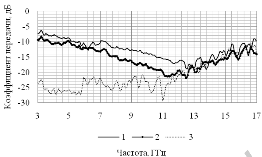
Рис. 4. Частотные зависимости коэффициента передачи конструкции экрана ЭМИ, в диапазоне частот 3–17 ГГц, выполненной на основе керамзита, содержащего водные растворы хлорида натрия: 1 – 3 см. на рис. 1
