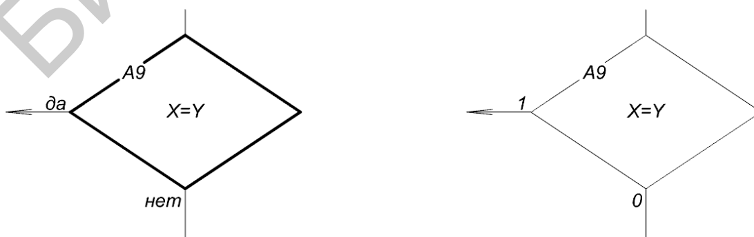
Рис. 2.12. Стили изображения символов схемы программы
