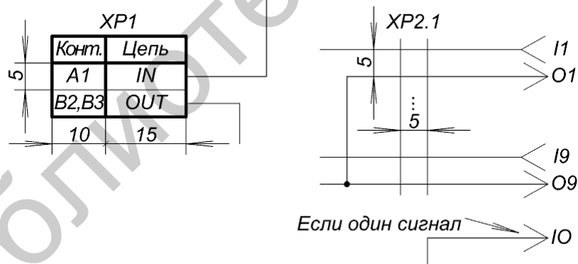
Рис. 2.10. Стили изображения УГО разъемов
