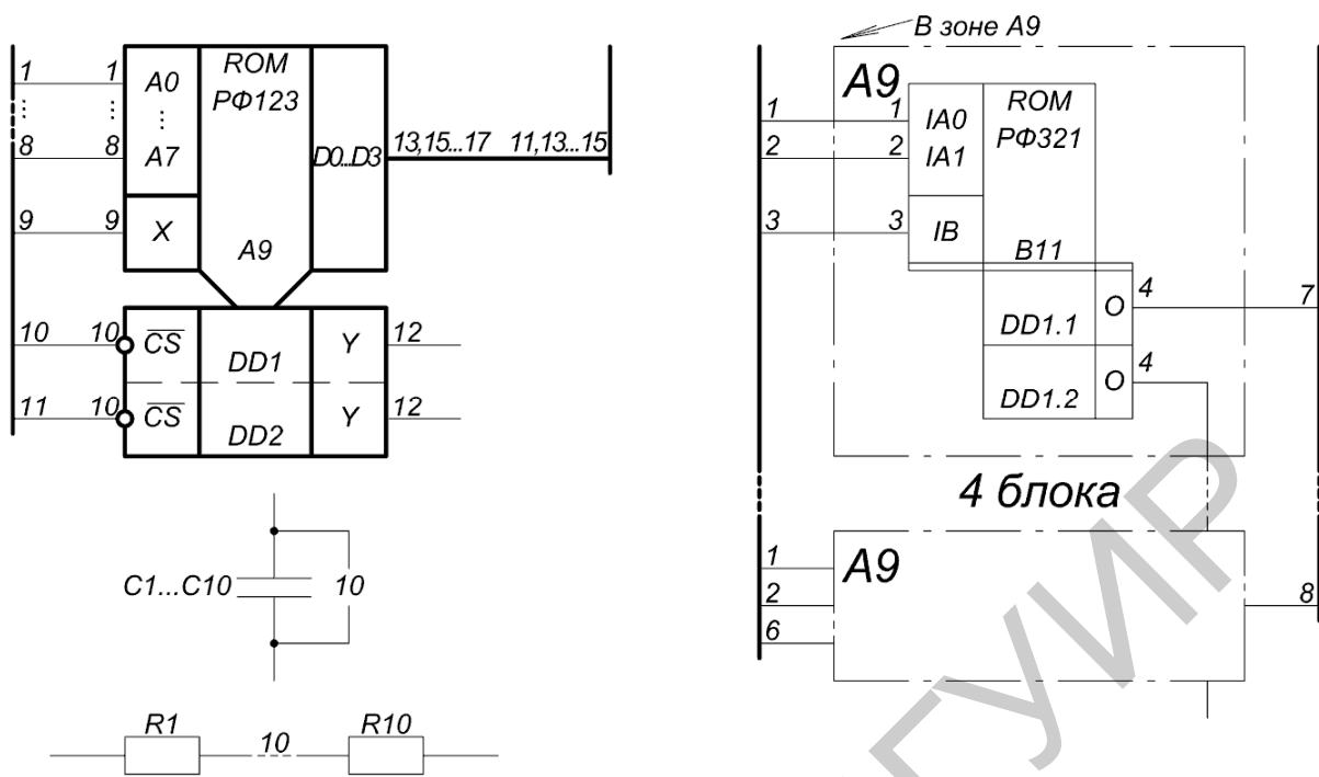
Рис. 2.9. Основные варианты сокращений
