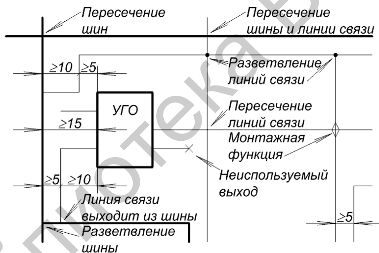
Рис. 2.7. Правила взаимного расположения УГО, линий контактов, линий связи и шин
