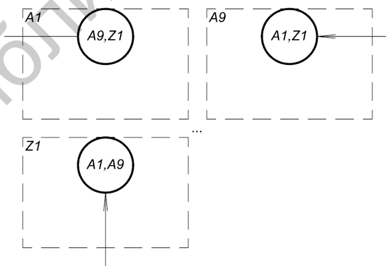
Рис. 2.13. Обозначение разрыва линии логической связи
