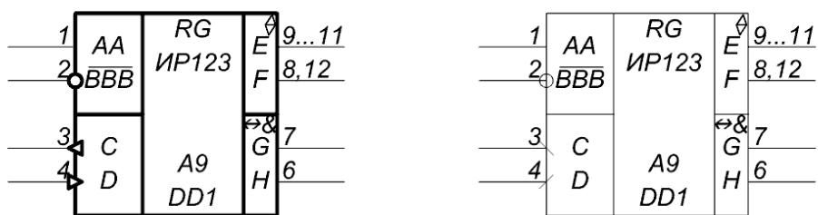
Рис. 2.6. Стили изображения УГО микросхем
