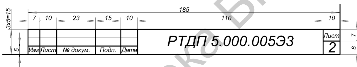
Рис. 2.5. Основная надпись по форме 2а
