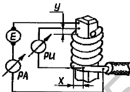
Рис. 3.5. Схема измерения переходного сопротивления
