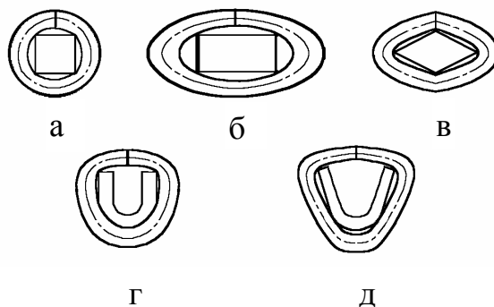
Рис. 3.2. Формы поперечного сечения выводов: квадратная (а), прямоугольная (б), ромбовидная (в), U-образная (г), V-образная (д)
