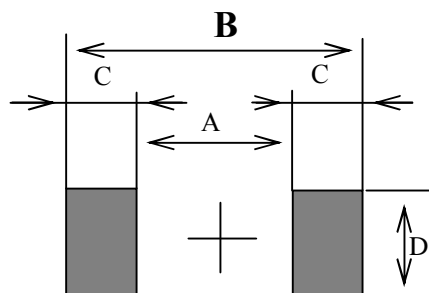
Рис. 4.1. Знакоместо чиповых резисторов и конденсаторов
