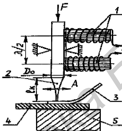
Рис. 2.5. Схема ультразвуковой сварки
