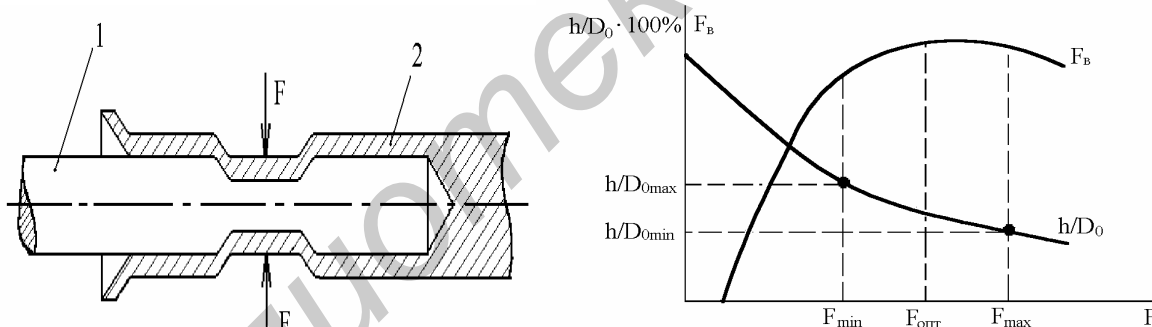
Рис. 3.6. Соединение обжатием (а) и диаграмма деформаций (б)
