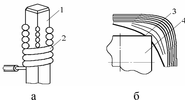
Рис. 3.1. Соединение накруткой (а) и врезание вывода в провод (б): 1–вывод, 2–провод, 3–область соединения, 4–кромка штыря
