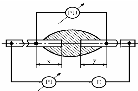
Рис.1.6. Схема измерения разности потенциалов на паяном соединении
