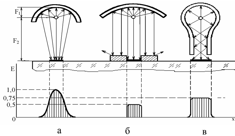
Рис. 1.4. Способы фокусировки ИК излучения
