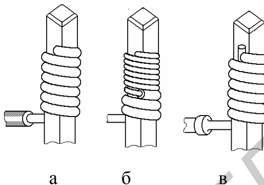
Рис. 3.3. Виды соединений накруткой
