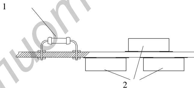
Рис. 4.2. Варианты установки на плату: 1 – элементов, монтируемых в отверстия; 2 – SMD
