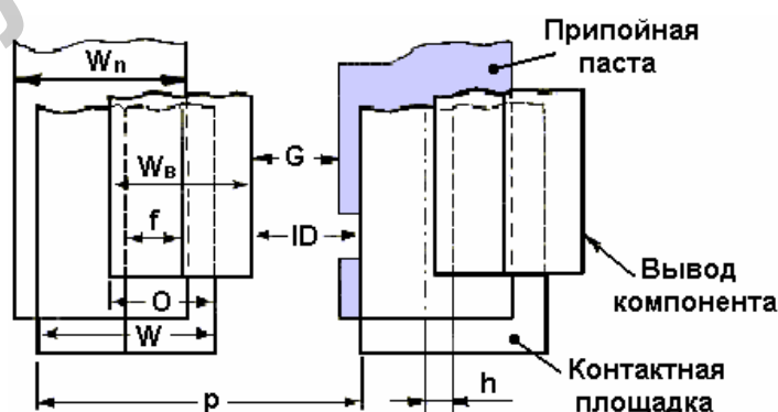
Рис. 4.4. Схема к расчёту точности позиционирования компонентов P – шаг выводов; W – ширина контактной площадки; W_B – ширина вывода; ID – гарантированный зазор исходя из требований изоляционной прочности;
