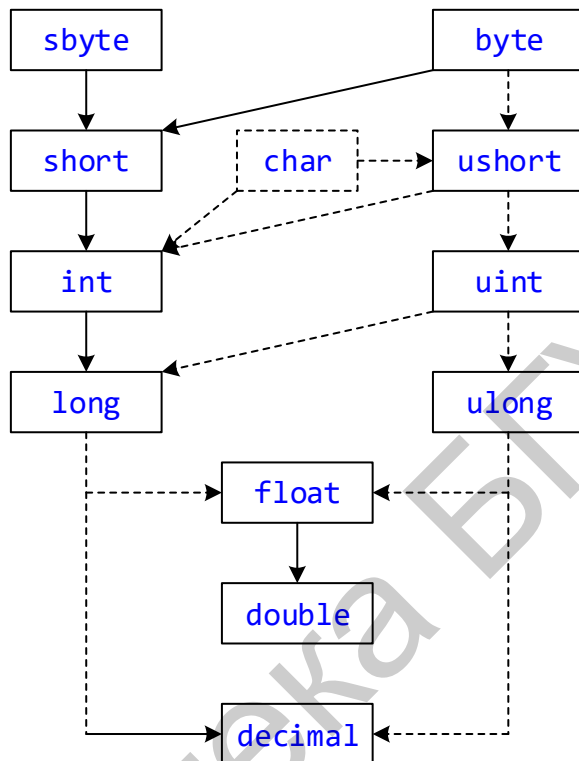
Рис. 2. Схема неявного преобразования числовых типов
