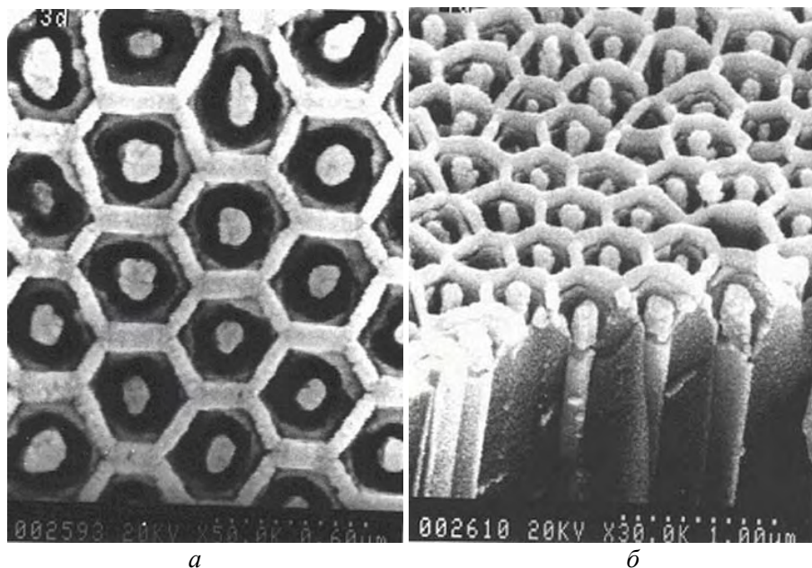
Рис. 5. Высокоупорядоченные матрицы пор в анодном диоксиде алюминия, заполненные никелем: a — вид сверху; б — поперечное сечение
