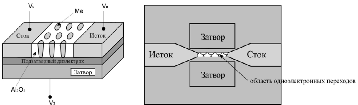
Рис. 7. Конструкции одноэлектронных транзисторов на основе самоорганизованных наноразмерных матриц пористого оксида алюминия, заполненных металлом
