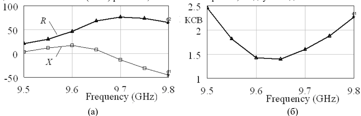
Рис.2. Активная ( R ) и реактивная ( X ) части входного сопротивления (а) и КСВ (б) по входу 1 с горизонтальной поляризацией в диапазоне частот
