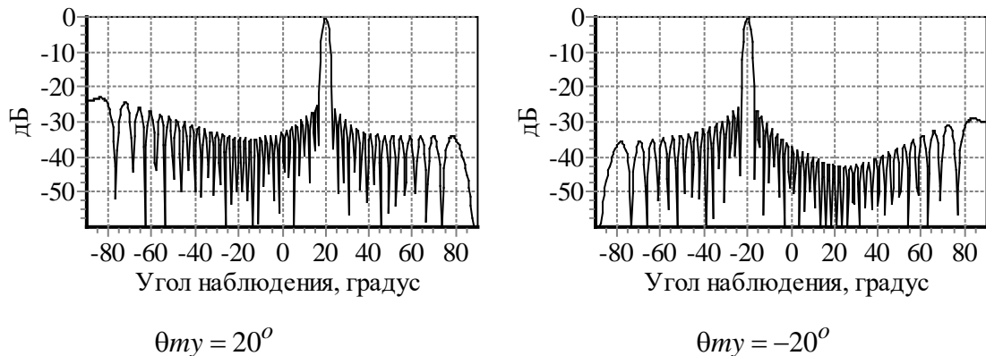
Рис.6. ДН в вертикальной плоскости для случая N_u=36 , шаг размещения излучателей D_u=21 мм, частота 9650 МГц
