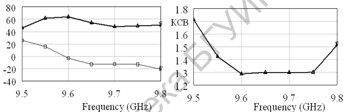
Рис.3. Активная ( R ) и реактивная ( X ) части входного сопротивления (а) и КСВ (б) по входу 2 с вертикальной поляризацией в диапазоне частот
