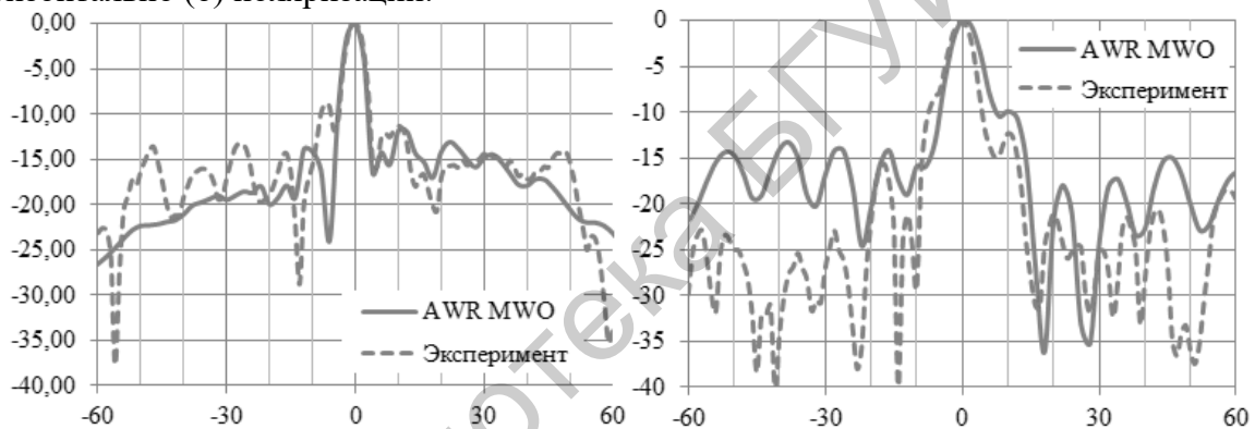
Рис.7. ДН на частоте 9,65 ГГц по вертикальной (а) и горизонтально (б) поляризации.
