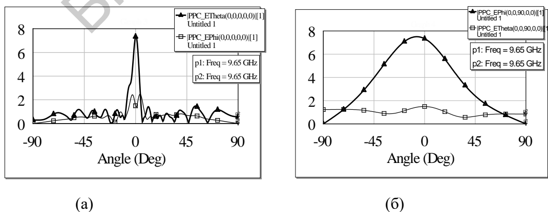
Рис.4. Диаграммы направленности при возбуждении входа 1 по горизонтальной поляризации (а) – ДН в горизонтальной плоскости; (б) – ДН в вертикальной плоскости
