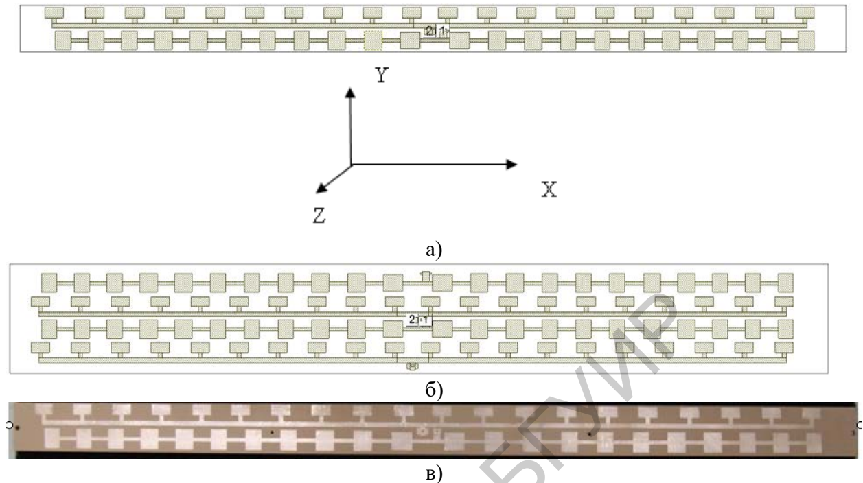
Рис.1. Схема построения и фотография макета решетки
