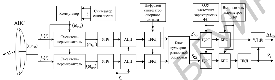
Рис. 3. Вариант структуры широкополосного моноимпульсного радиолокатора сопровождения по одной угловой координате
