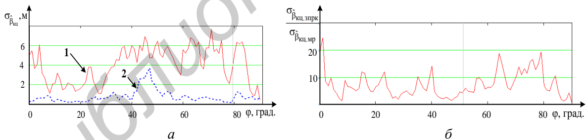
Рис. 5. Зависимость \sigma_{\hat{\beta}_{кц}} кажущегося центра цели (а) и отношения \sigma_{\hat{\beta}_{кц,зпрк}} / \sigma_{\hat{\beta}_{кц,мр}} (б) от ракурса наблюдения, измеренных: 1 – станцией сопровождения целей ЗРПК; 2 – широкополосным моноимпульсным радиолокатором сопровождения
