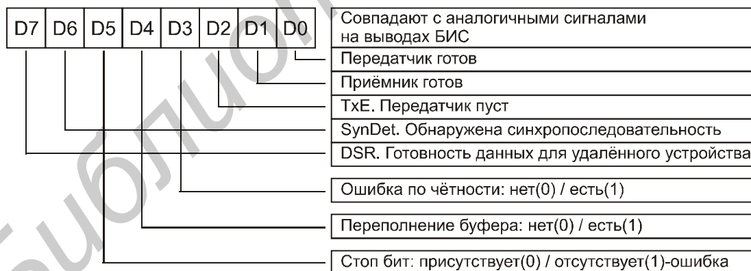
Рис. 41. Формат слова состояния KP580BB51
