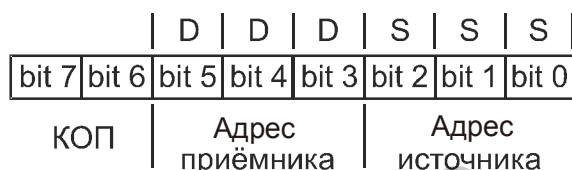
Рис. 13. Формат первого байта команды KP580BM80A
