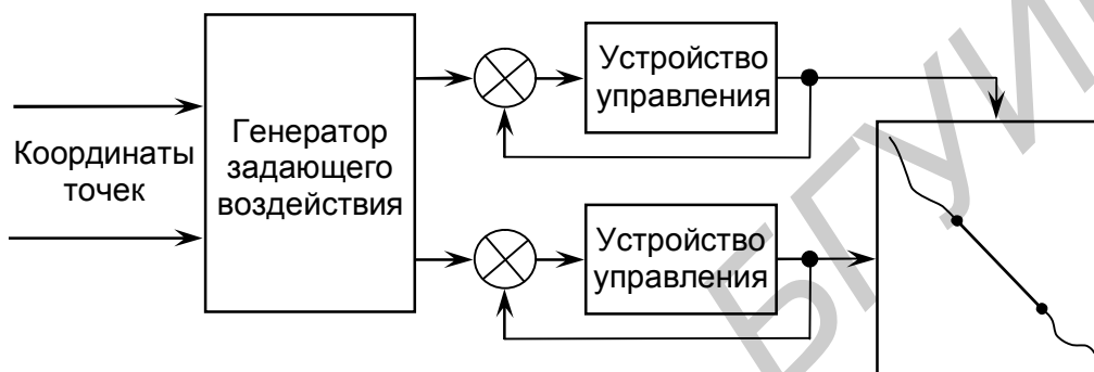
Рис. 50. Контурное управление
