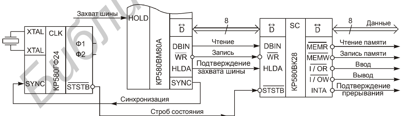
Рис. 18. Системный контроллер и шинный формирователь КР580ВК28
