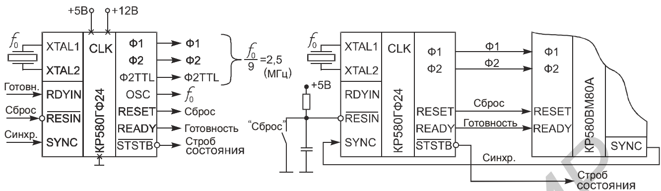
Рис. 17. Генератор тактовых импульсов КР580ГФ24
