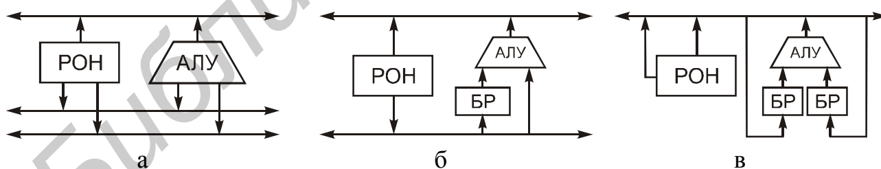
Рис. 4. Топология:
