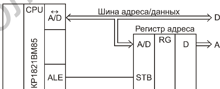
Рис. 25. Мультиплексирование шин
