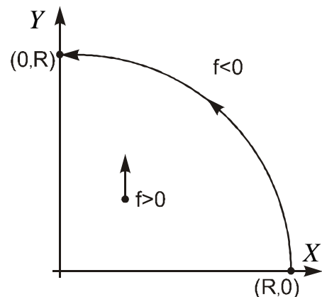
Рис. 53. Представление дуги методом оценочной функции
