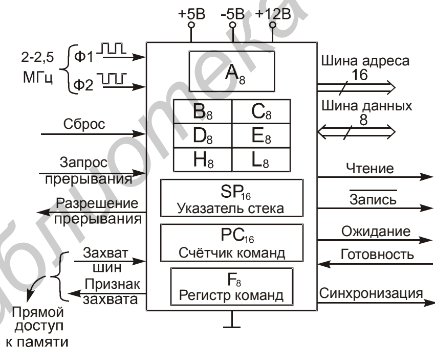
Рис. 11. Структурная схема КР580ВМ80А
