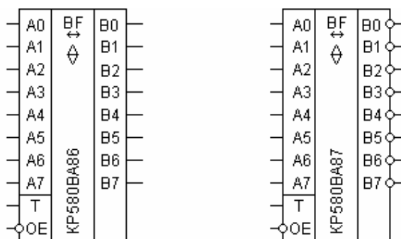
Рис. 20. Шинные формирователи
