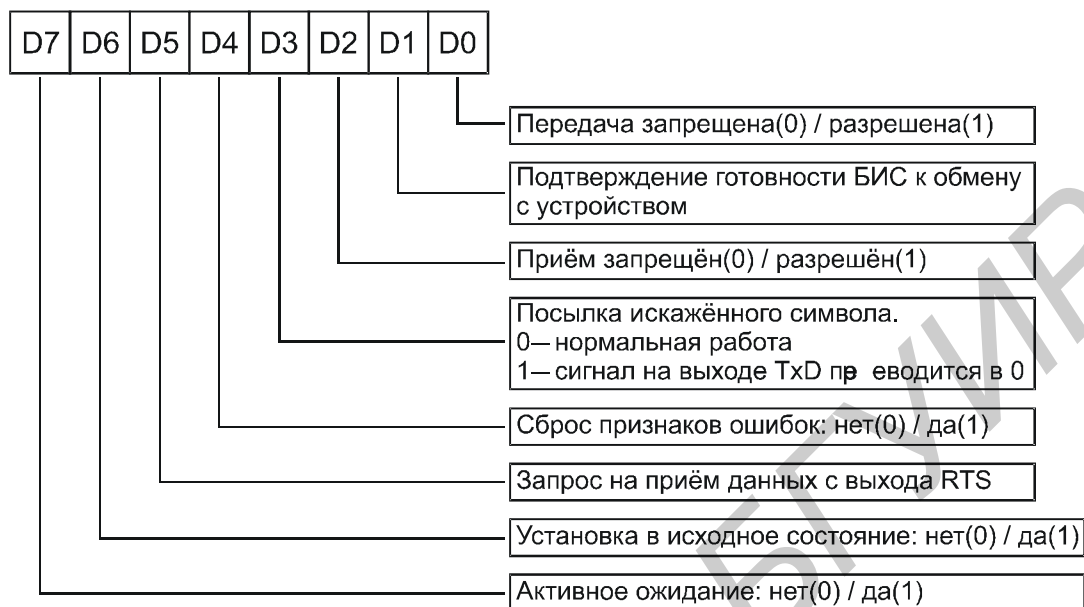
Рис. 40. Формат слова команды KP580BB51
