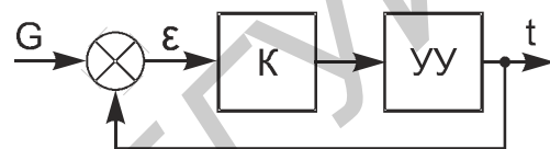
Рис. 47. П-регулятор
