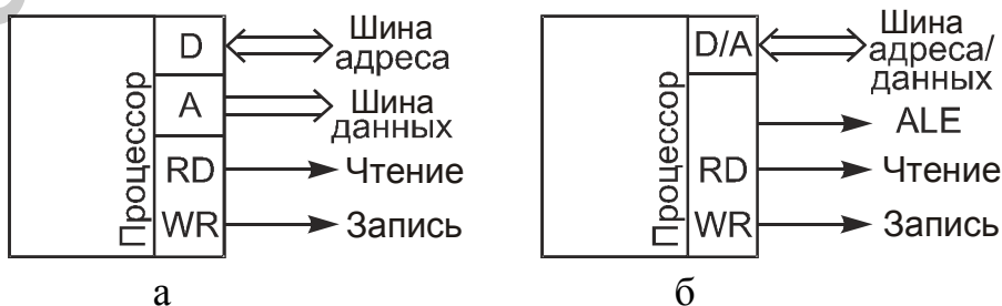
Рис. 5. Микропроцессор:
