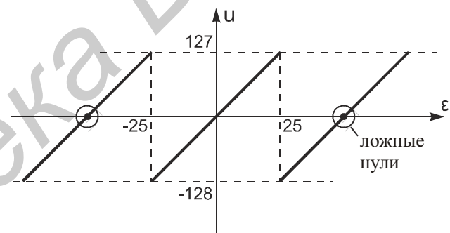
Рис. 48. Ложные нули
