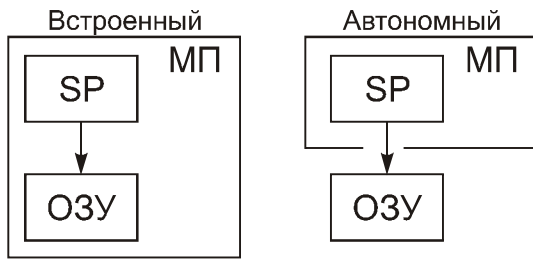
Рис. 28. Типы стека
