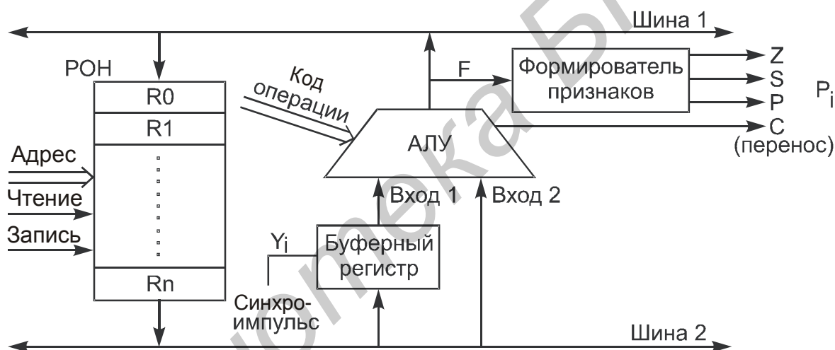
Рис. 7. Упрощенная схема микропроцессора
