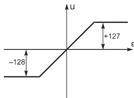
Рис. 49. Подавление ложных нулей
