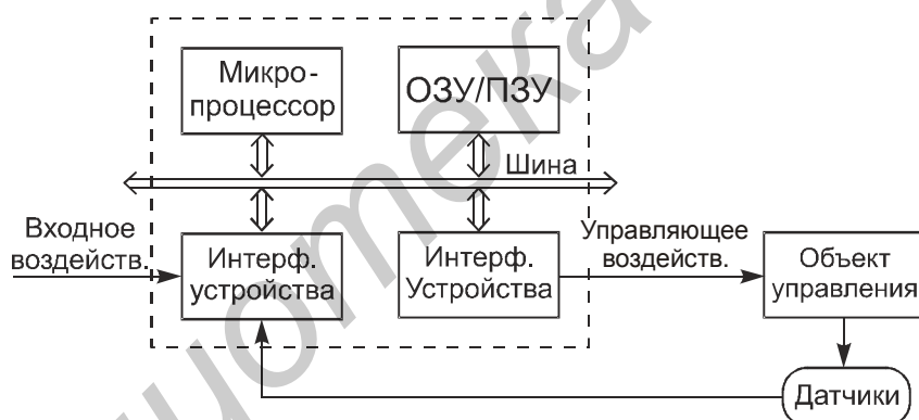
Рис. 1. Система управления на базе микроЭВМ
