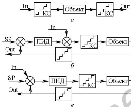
Рис. 1 – Структуры моделирования: а – при отсутствии обратной связи (S1); б – с обратной связью, при подаче ТС после регулятора (S2); в – с обратной связью, при подаче ТС по каналу задания (S3); In – точка приложения ТС; Out – выходной сигнал для анализа
