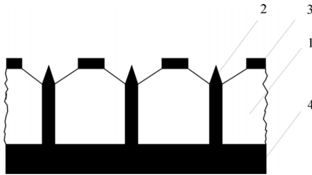
Рис. 6. Поперечное сечение матричных автоэмиссионных катодов с управляющим электродом: 1 – диэлектрическая матрица анодного оксида алюминия; 2 – металлические эмиттеры; 3 – управляющий электрод; 4 – металлическая подложка
