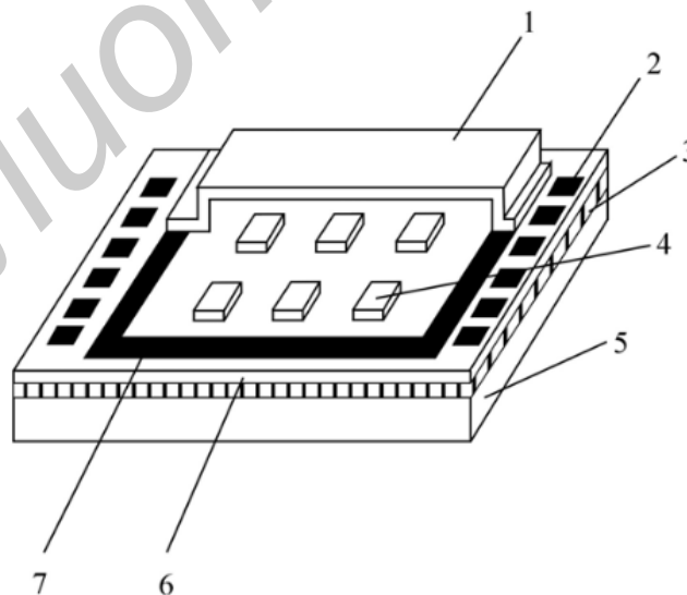
Рис. 2. Алюминиевый корпус гибридных интегральных схем:
