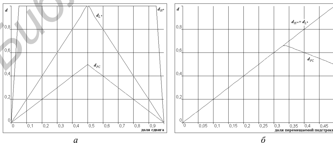
Рис. 3. Зависимости d_{H^*} , d_{L^*} и d_{PC} для случаев циклического сдвига k символов (а); перестановки подстрок длиной k символов (б)
