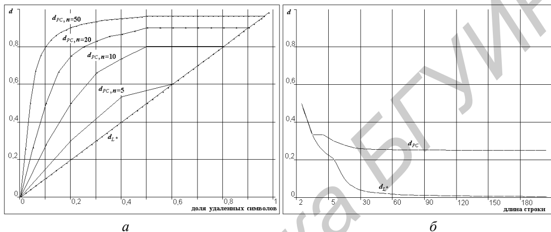
Рис. 2. Зависимости d_{L^*} и d_{PC} для случаев k пропущенных символов (а); пропуска (добавления) символа в позиции k (б)
