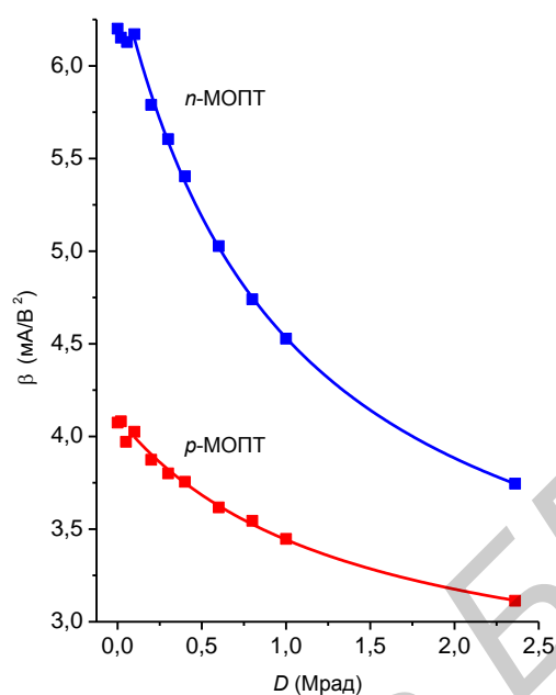
Рис. 4. Дозовая зависимость удельной крутизны p -МОП и n -МОП транзисторов ИМС 1554ЛН1 при облучении \gamma -квантами Co^{60}
