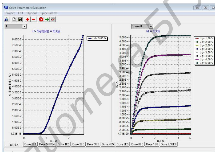
Рис. 1. Окно программы с исходными ВАХ n -МОПТ ИМС 1554ЛН1
