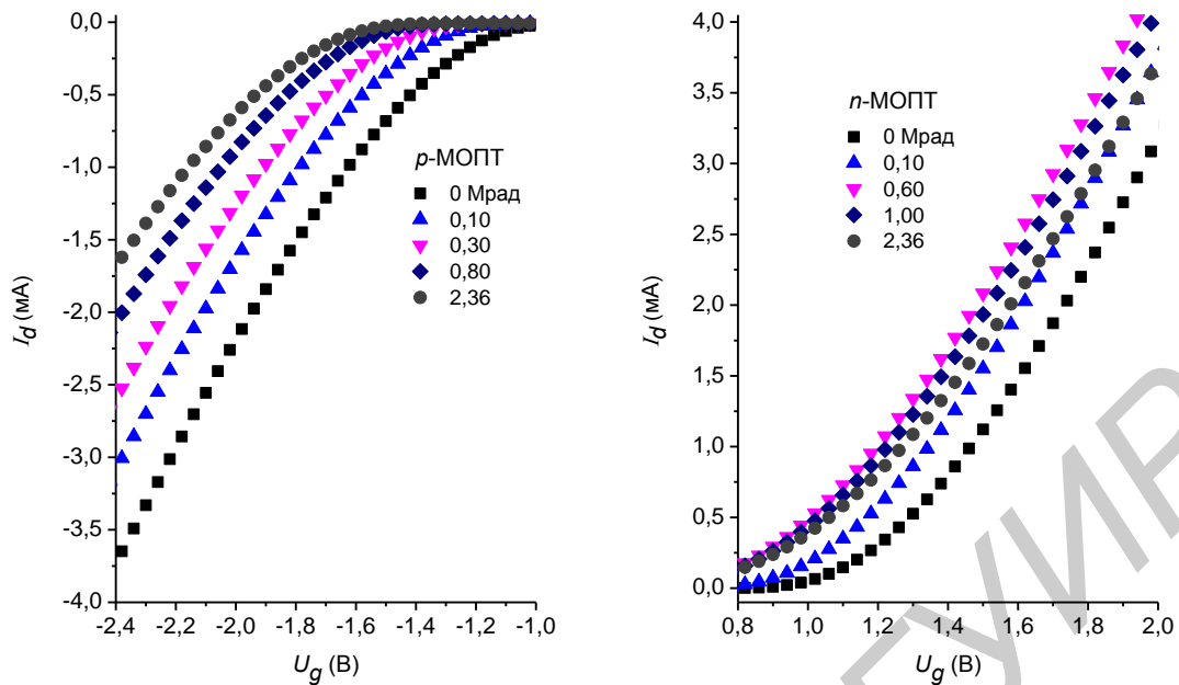
Рис. 2. Изменения стокзатворной характеристики p -МОП и n -МОП транзисторов ИМС 1554ЛН1 при облучении \gamma -квантами Co^{60} .
