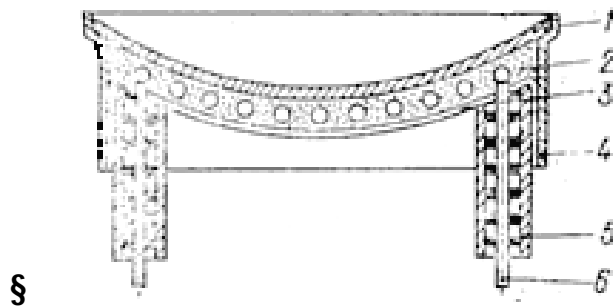
Рис. 1.1 Конструкция КПУ МГП с монокристаллическим подогревателем (1 – ядро катода; 2 – изолирующий материал; 3 – экран (Ni); 4 – держатель (Ni); 5 – трубка вывода подогревателя (Ni); 6 – подогреватель (W))
