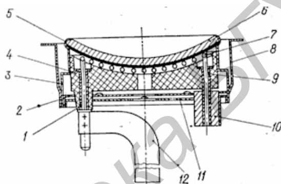
Рис. 1.2 Конструкция КПУ МГП (1,9 – пистоны (Ta); 2,3,8,11 – экраны (Ta); 4 – изолятор ( Al_2O_3 ); покрытие Al_2O_3 + W и Al_2O_3 ; 6 – катод; 7 – подогреватель (W); 10 – втулка (Mo); пластина (Ta)).
