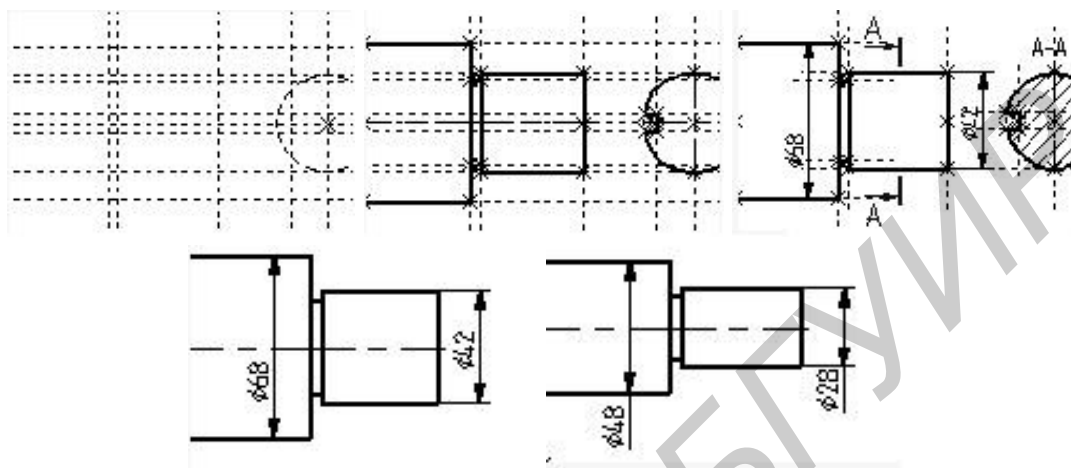
Рис. 6.1 Иллюстрация последовательности построения чертежа
