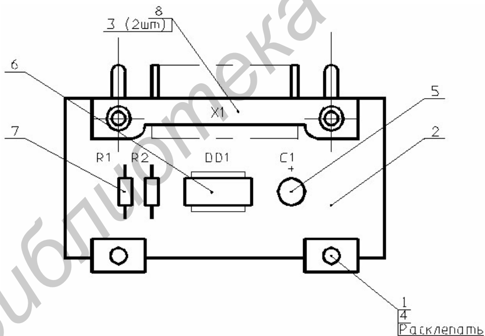
Рис. 5.3. Фрагмент сборочного чертежа платы таймера
