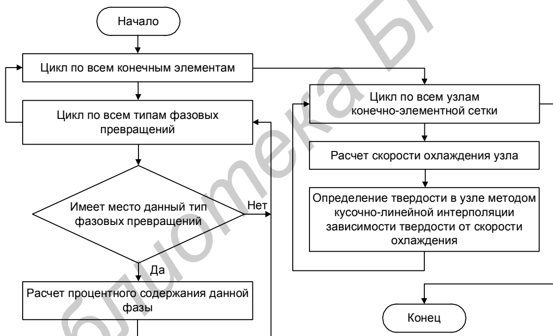
Рис. 4.3 Логическая схема расчета фазового состава и твердости
