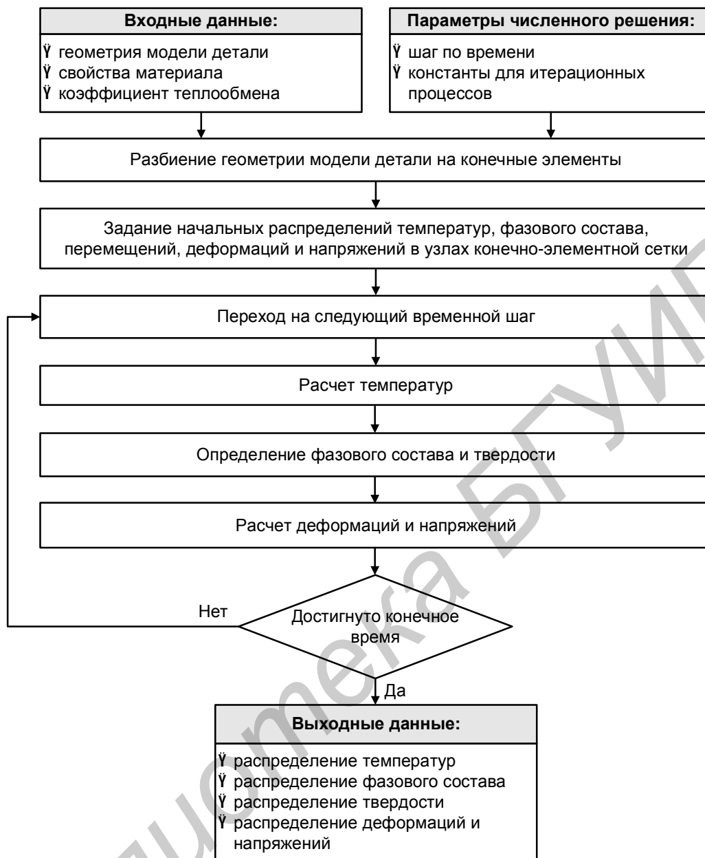
Рис. 4.1 Алгоритм комплексной модели теплофизических процессов при термообработке
