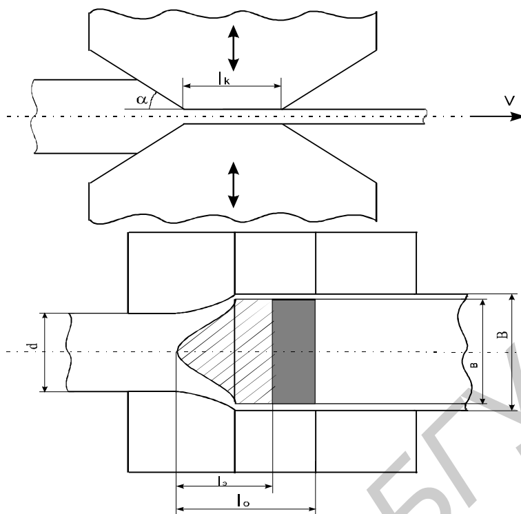
Рис. 2.4 Схема очага деформации
