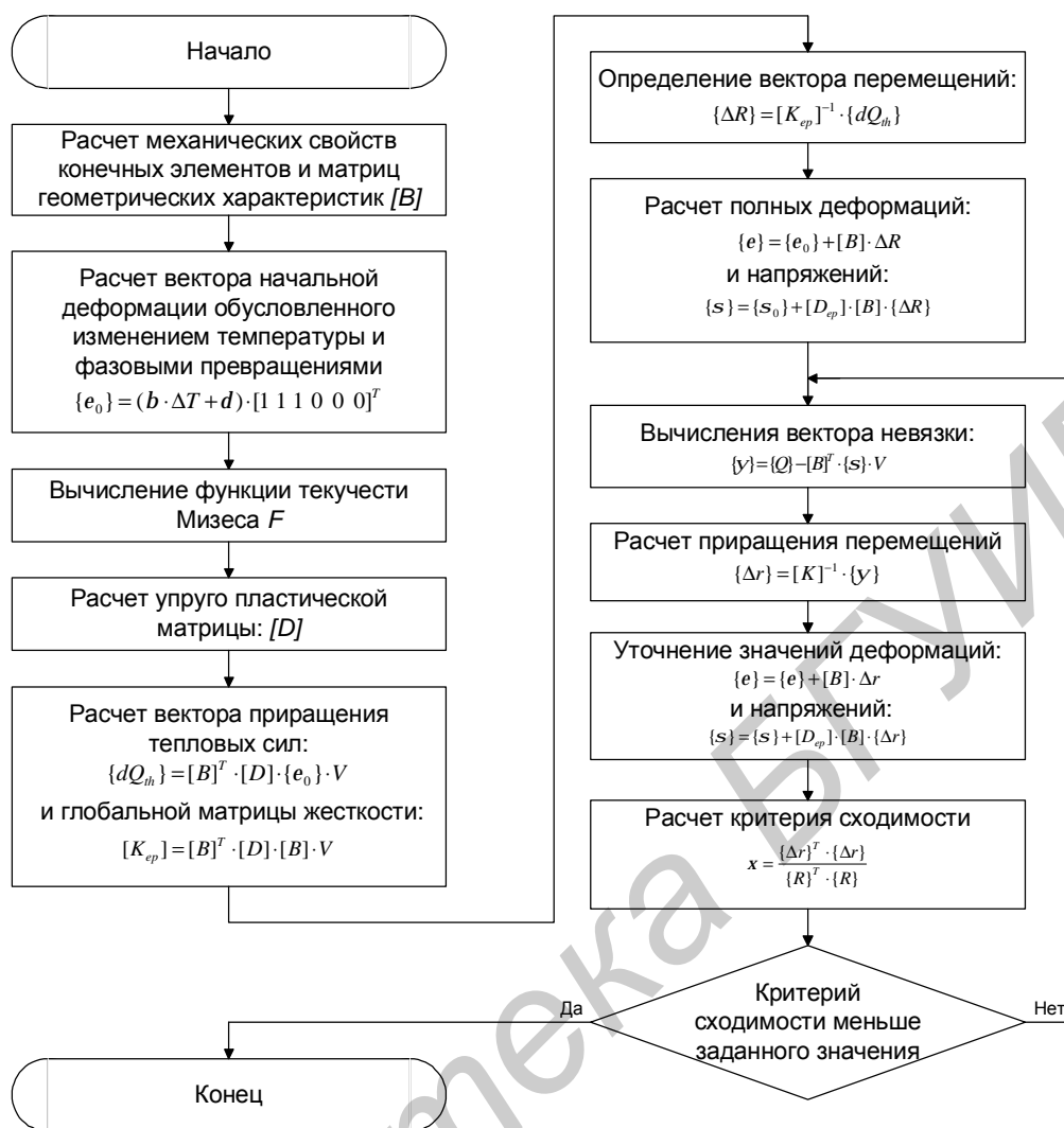
Рис. 4.4 Логическая схема расчета перемещений, деформаций и напряжений
