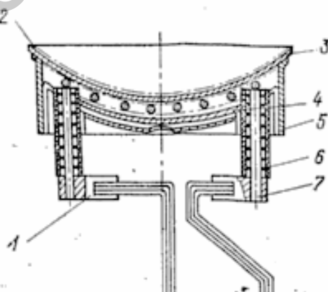
Рис. 1.3 Конструкция КПУ МГП с малым временем разогрева (1 – держатель вывода подогревателя (Mo); 2 – эмиссионное покрытие; 3 – ядро катода; 4 – экран (Ni); 5 – держатель (Ni); 6 – керамический изолятор; подогреватель (W)).
