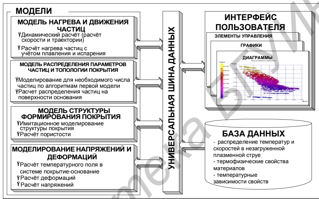
Рис. 1.5 Структурная схема программного комплекса Plasma
