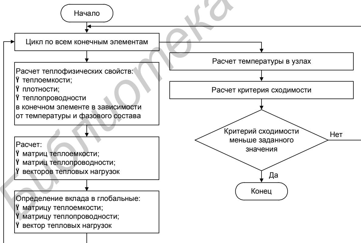
Рис. 4.2 Логическая схема расчета температур
