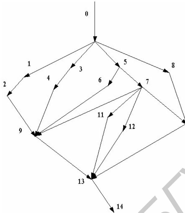
Рис. 5.4. Граф ТП сборки платы таймера
