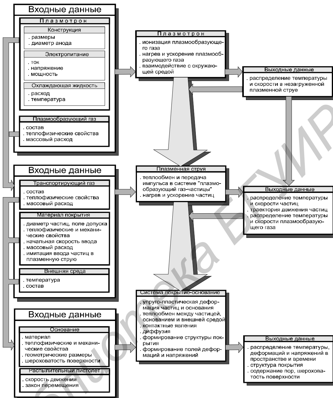
Рис. 1.4 Схема комплексного моделирования процесса плазменного напыления покрытий
