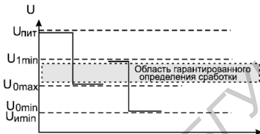
Рис. 3.7. Уровни напряжений
