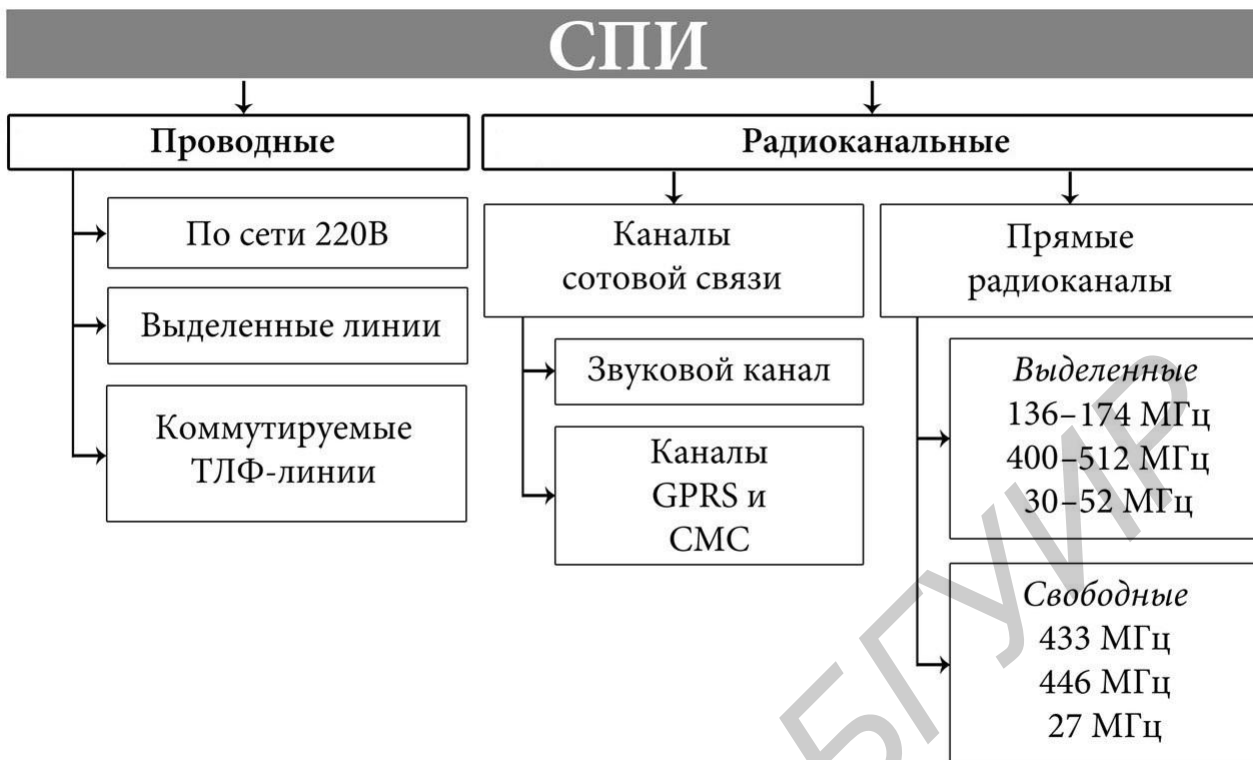
Рис. 1.1. Виды каналов передачи информации систем передачи извещений
