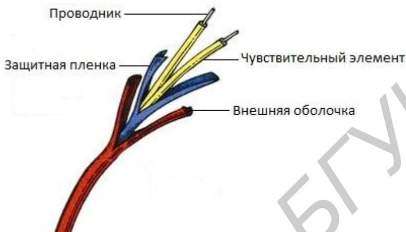
Рис. 2.6. Термокабель
