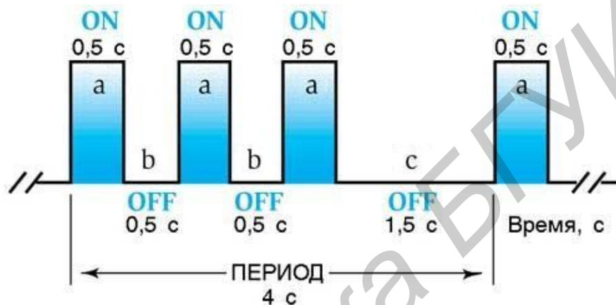
Рис. 5.8. Временная диаграмма стандартного сигнала оповещения СПС:
