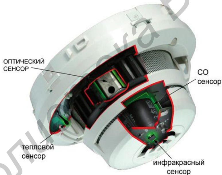
Рис. 2.14. Комбинированный пожарный извещатель
