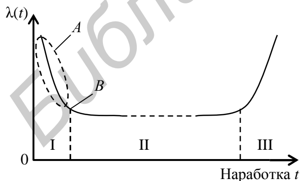
Рис. 2.14. Типичная \lambda -характеристика РЭУ технологическим прогоном РЭУ.
