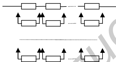
Рис. 2.8. Раздельное (поэлементное) резервирование
