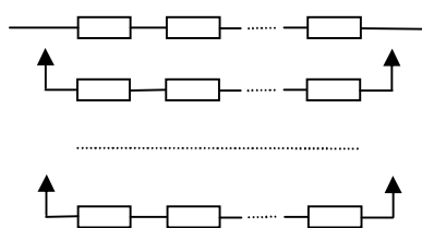
Рис. 2.7. Общее резервирование
