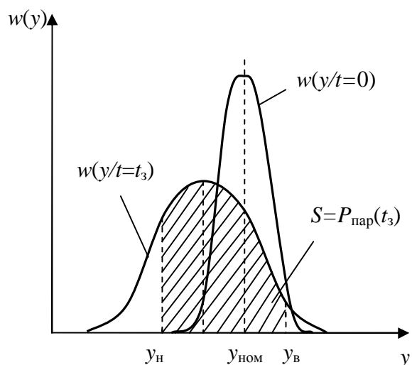
Рис. 2.6. Влияние процесса эксплуатации на распределение выходного параметра РЭУ: y_{н} , y_{в} – нижняя и верхняя допустимые границы
