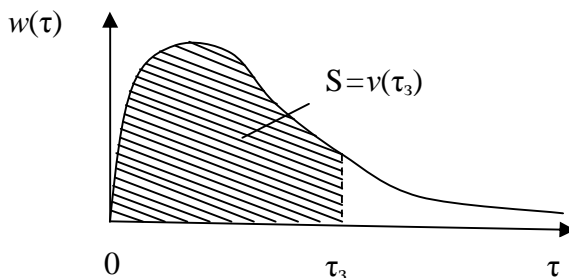
Рис. 2.5. К вопросу об определении величины v(\tau_3)
