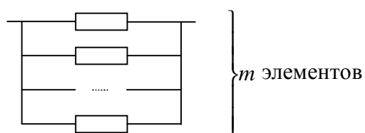
Рис. 2.9. Параллельный способ соединения элементов резервируемого узла
