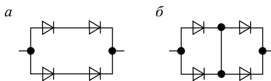
Рис. 2.11. Примеры смешанного соединения элементов резервируемого узла: a – последовательно-параллельная схема; б – параллельно-последовательная схема
