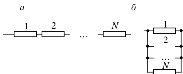
Рис. 2.1. Схемы (модели) соединения элементов в устройстве с точки зрения надёжности: a – последовательное соединение; б – параллельное соединение ( N – количество элементов в устройстве)
