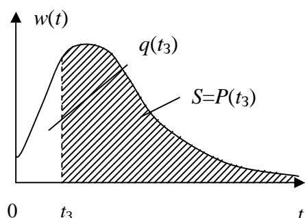
Рис. 2.3. К определению вероятности безотказной работы и вероятности отказа
