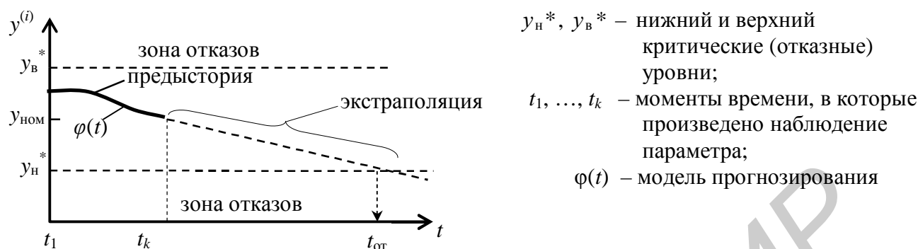
Рис. 2.15. Прогнозирование методом экстраполяции параметра
