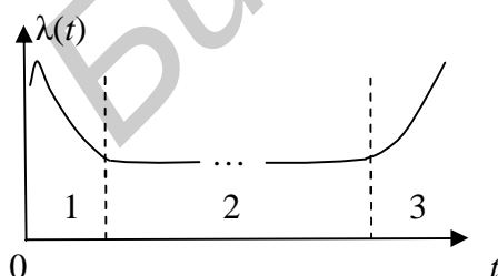
Рис. 2.4. Типичный вид \lambda -характеристики РЭУ
