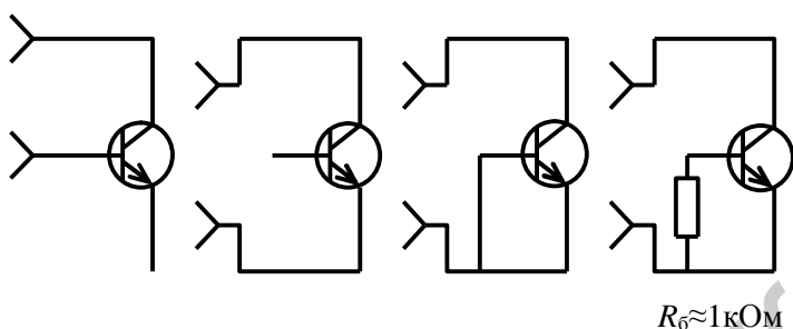
Рис. 2.13. Типовые схемы подачи обратных напряжений
