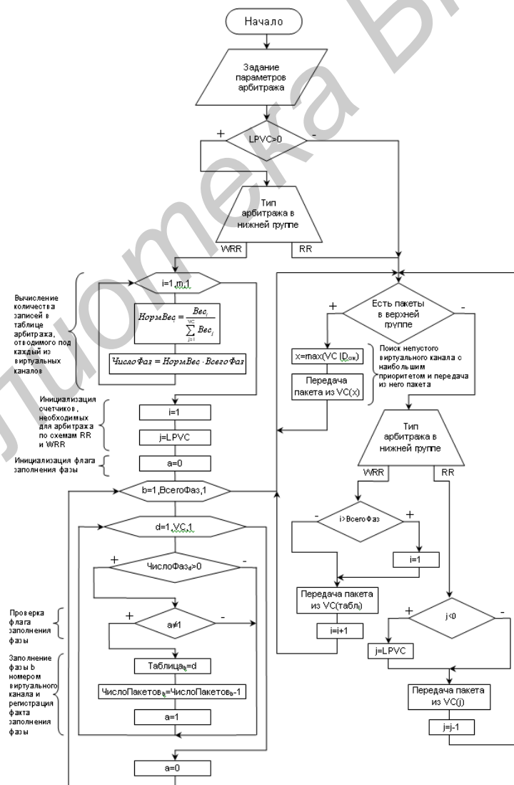
Рис. 1 – Блок-схема алгоритма арбитража виртуальных каналов
