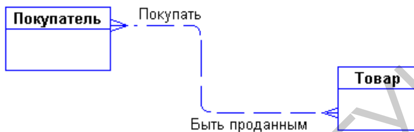
Рисунок 3.22 – Пример модальности связей
