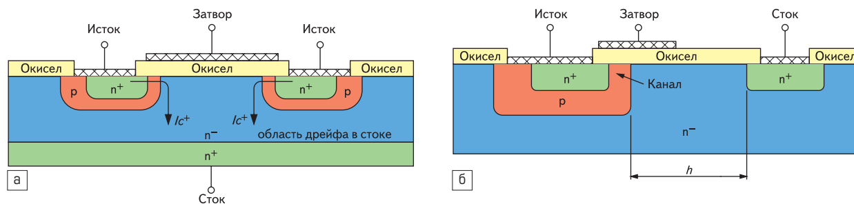
Рис. 1. а) Структура MOSFET с коротким каналом, полученным методом двойной диффузии; б) Структура вертикального ДМОП-транзистора
