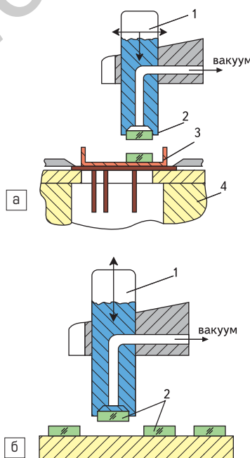
Рис. 6. Контактнореактивная пайка кристаллов: а) захват кристалла; б) присоединение кристалла к корпусу
