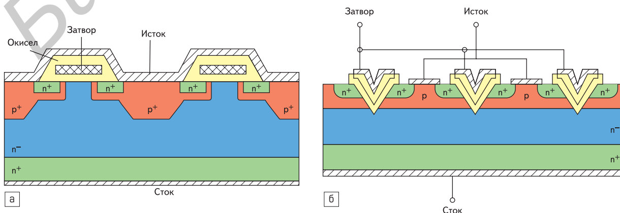
Рис. 3. Конструкция мощных MOSFET с вертикальным p-каналом: а) с поликремниевым затвором; б) p-канального с двойной диффузией
