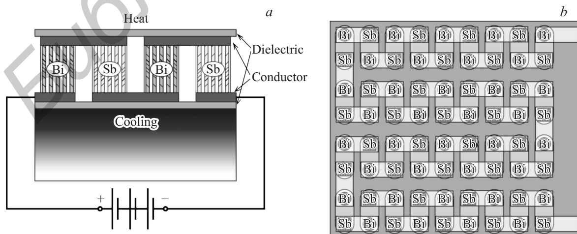
Рис. 1. Схематическое изображение термоэлектрической ячейки на основе массивов нанопроводов Bi и Sb (a) и термоэлектрической батареи из последовательно соединенных термоэлектрической ячеек (b).
