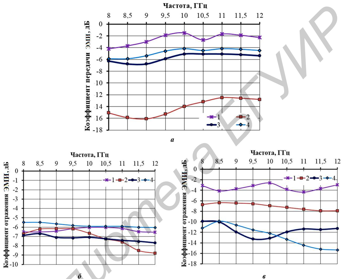
Рисунок 3. – Частотные зависимости коэффициента передачи (а), коэффициента отражения, измеренного в режиме согласованной нагрузки (б), и короткого замыкания (в) исследованных образцов красок
