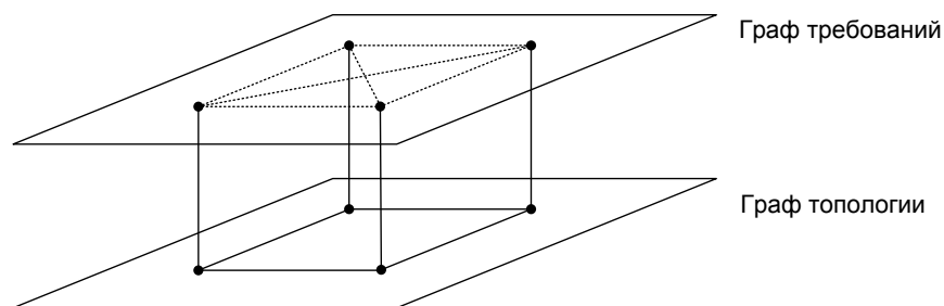
Постановка задачи
