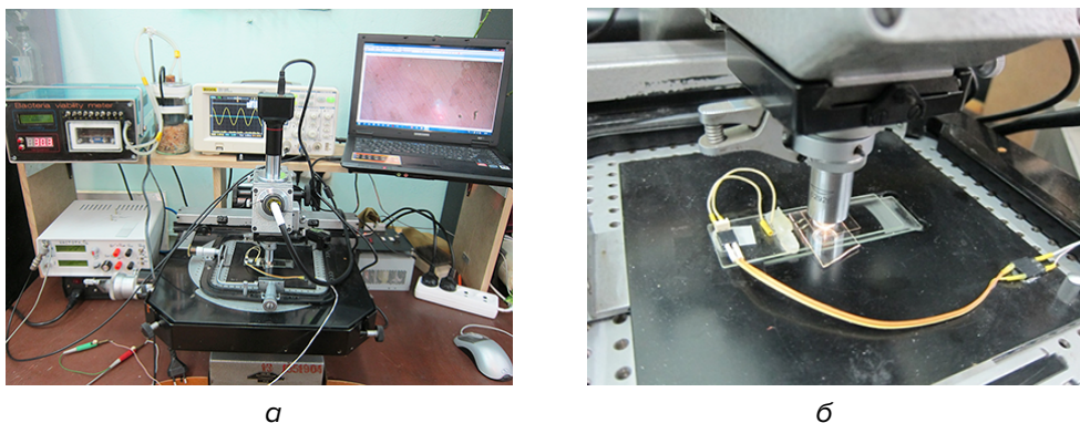
Рис. 2. Фотографии общего вида: а – экспериментальной установки; б – одноразовой измерительной ячейки
