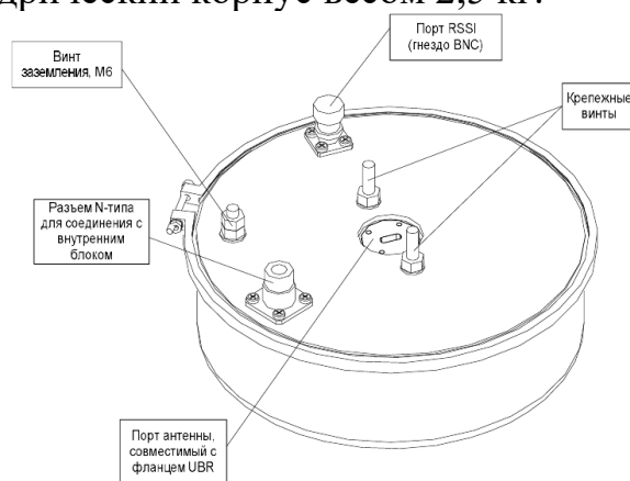
Рис. 86. Радиоблок CFM-LM
