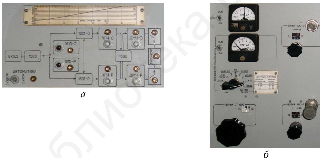
Рис. 48. Передняя панель шкафа стойки 1600:
