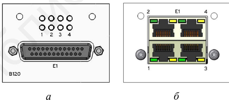
Рис. 93. Модуль 4 \times E1 :
