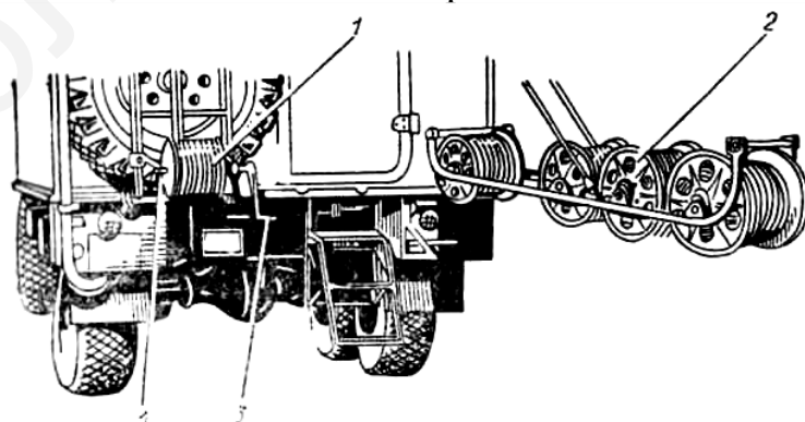
Рис. 80. Разматывание и наматывание фидеров и силового кабеля:
