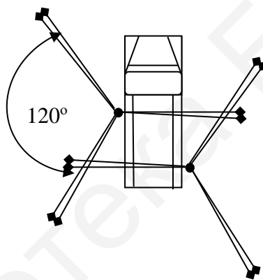
Рис. 77. Расположение оттяжек при разворачивании двух мачт
