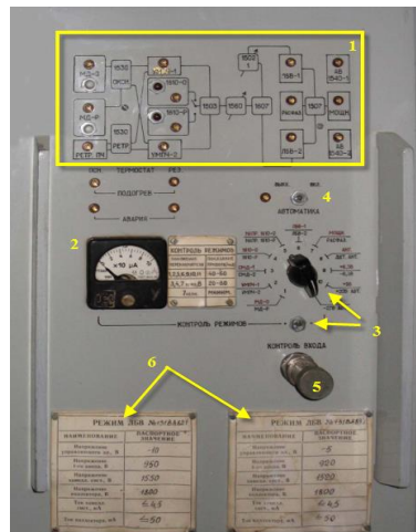
Рис. 45. Верхняя часть передней панели стойки 1500: 1 – упрощенная трактовая мнемосхема; 2 – контроль режимов; 3 – переключатель и тумблер прибора; 4 – тумблер включения автоматики; 5 – ВЧ разъем для измерения уровня видеосигналов на входе приборов МД-О и МД-Р
