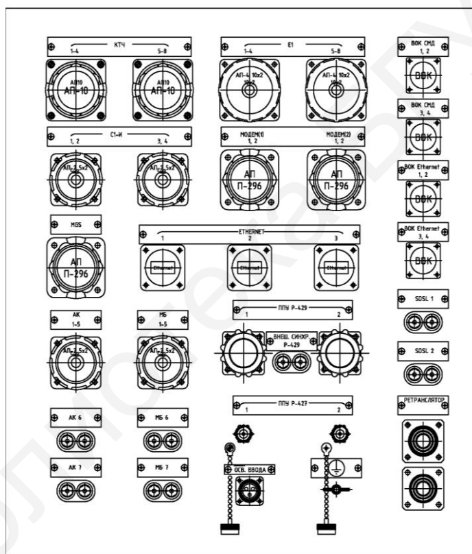
Рис. 71. Кабельный ввод 2
