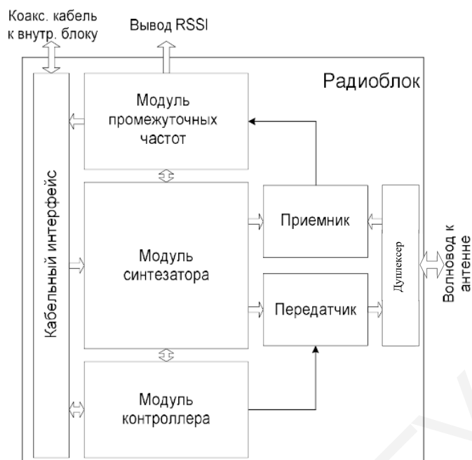
Рис. 88. Функциональная схема радиоблока
