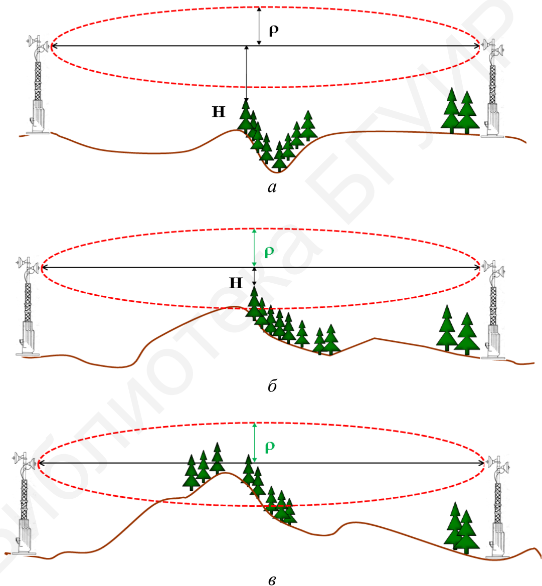
Рис. 8. Варианты радиорелейных интервалов: а – открытый; б – полуоткрытый; в – закрытый
