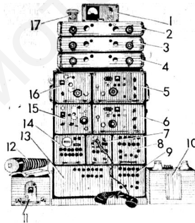
Рис. 33. Стойка приемопередатчика:
