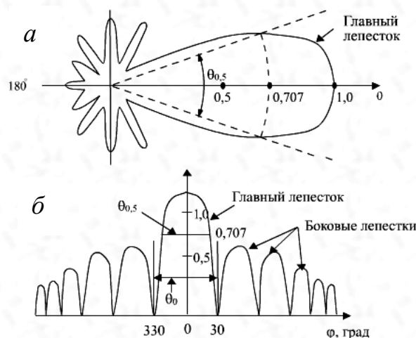
Рис. 9. Диаграмма направленности: а – в полярной системе координат; б – в прямоугольной системе координат
