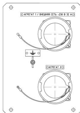
Рис. 70. Ввод питания
