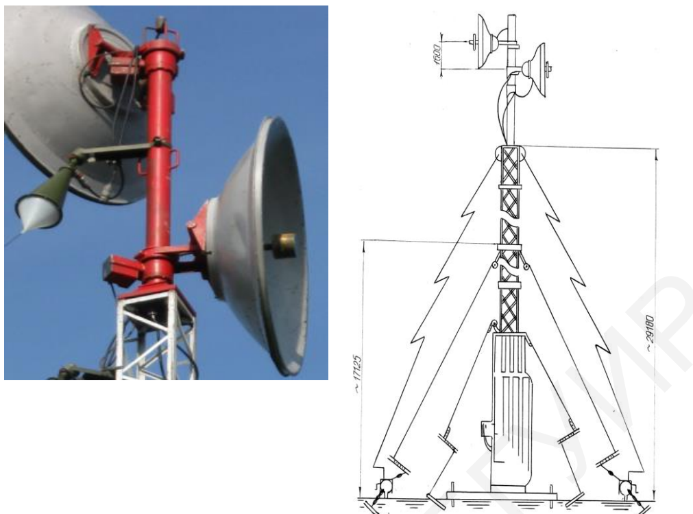
Рис. 43. Общий вид основного антенно-мачтового устройства
