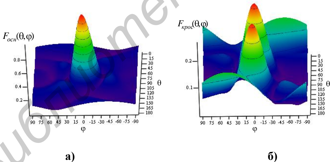
Рисунок 2 – Нормированные ДН конформной антенной решетки по \theta -ой (основной) составляющей поля (а) и по \varphi -ой (крсовой) составляющей поля (б)
