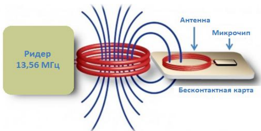
Рисунок 1 – Принцип работы NFC модуля в фитнес-браслетах [3]
