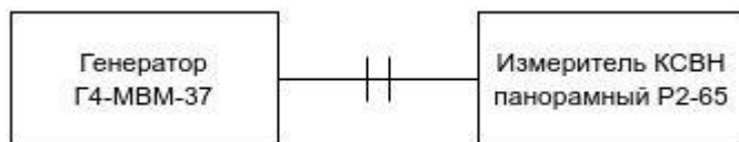
Рисунок 3 – Схема соединения приборов при измерении КСВН выхода генератора.
