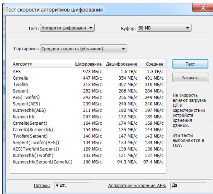
Рисунок 2 – Тест скорости алгоритмов шифрования VeraCrypt
