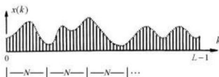
Рисунок 1– Секционирование входной последовательности при вычислении СПМ по методу Бартлетта
