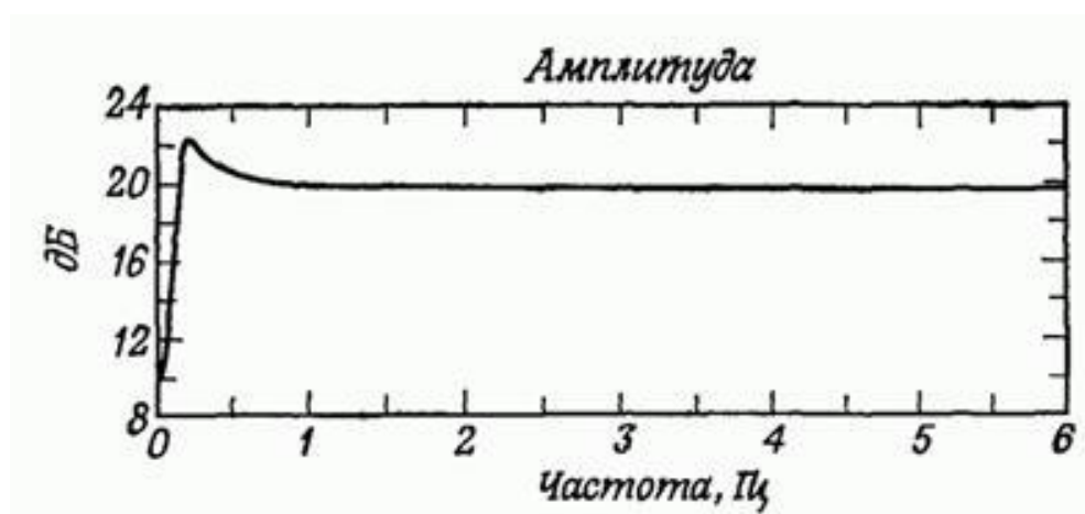
Рисунок 1 – Амплитудная характеристика цифрового фильтра, рассчитанного методом согласованного z-преобразования полюсов и нулей аналогового фильтра
