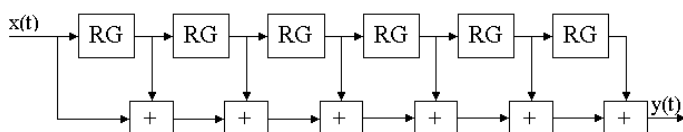
Рисунок 1. Структурная схема однородного фильтра седьмого порядка
