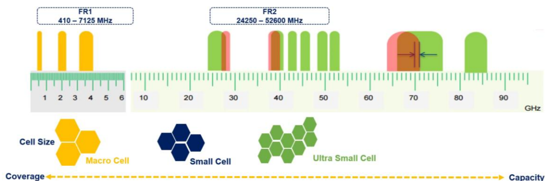
Рисунок 1 – Частотные диапазоны 5G NR
