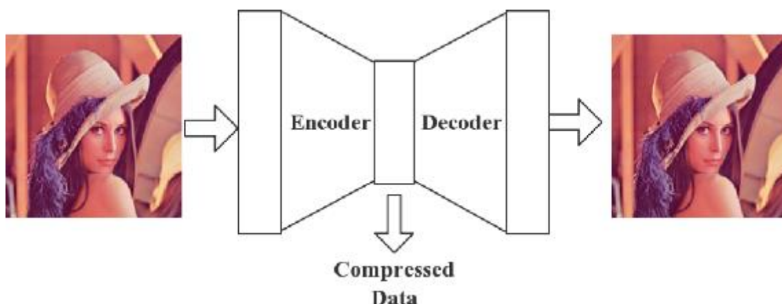
Рисунок 1 – Упрощенная архитектура автоэнкодера
