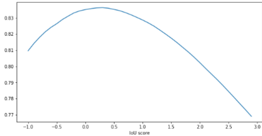
Рисунок 99 – График зависимости IoU от порога PAN
