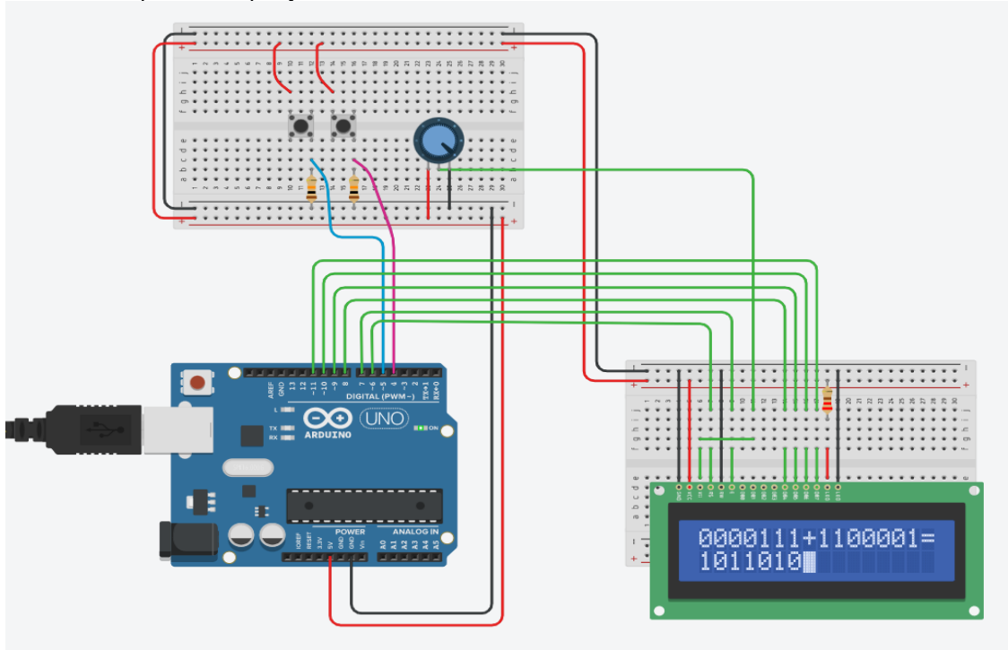
Рисунок 3 - Вид схемы двоичного сумматора на Arduino
