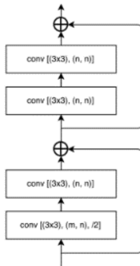
Рисунок 81 – Архитектура encoder блока
