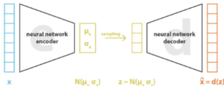
Рисунок 9 – Архитектура variational autoencoder
