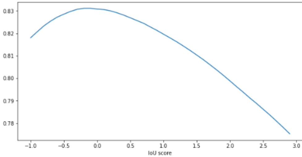
Рисунок 85 – График зависимости IoU от порога LinkNet
