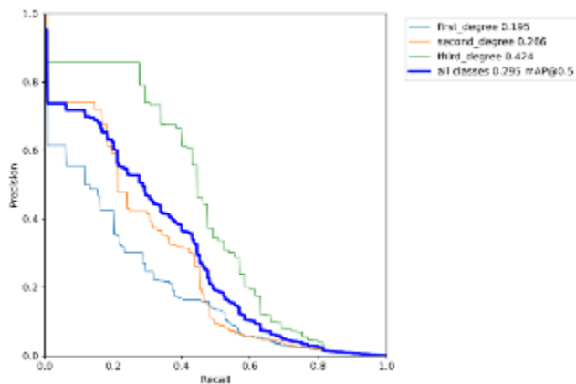
Рисунок 116 – Зависимость Precision от Recall модели YOLOv5s(640x640)
