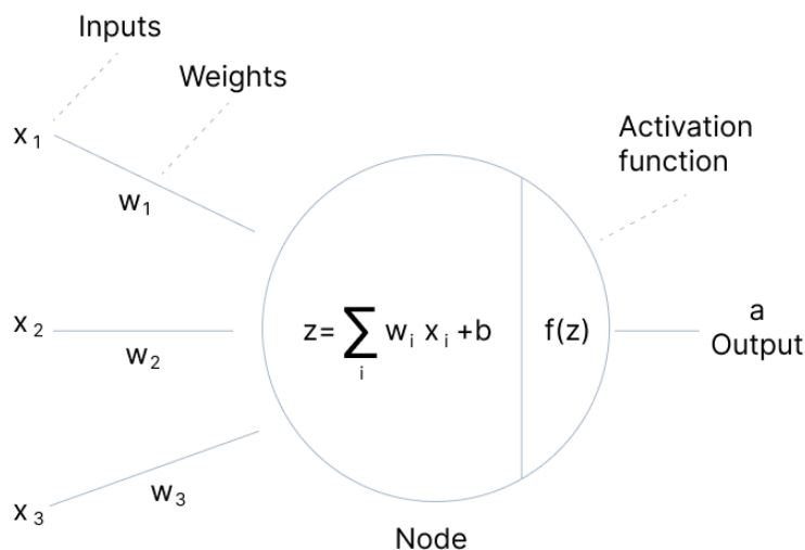
Рисунок 1 - Схема работы функции активации
