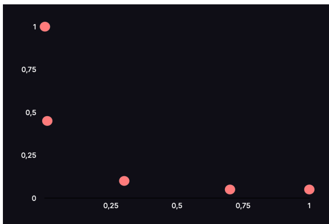
Рисунок 18 – Значения логарифмических потерь при прогнозах с разной вероятностью Если мы построим график логарифмических потерь для перечня спам-писем со всеми возможными видами вероятностей, график будет выглядеть как на рисунке 19.
