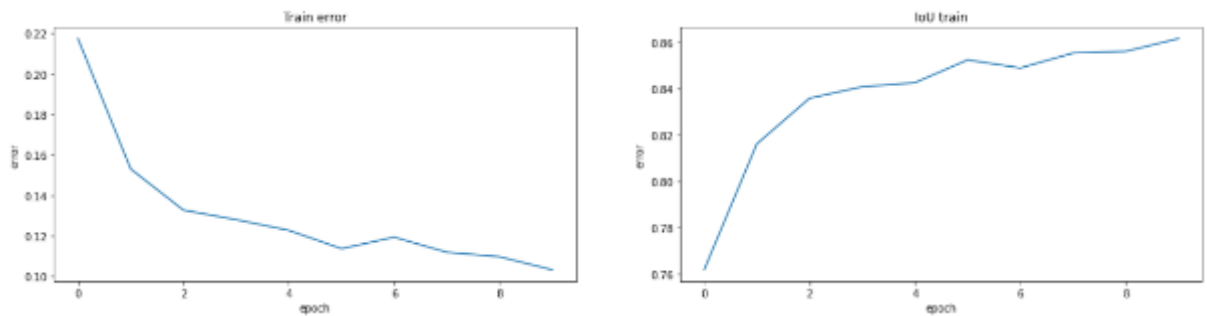
Рисунок 89 – Ошибка PSPNet на тренировочных данных и IoU
