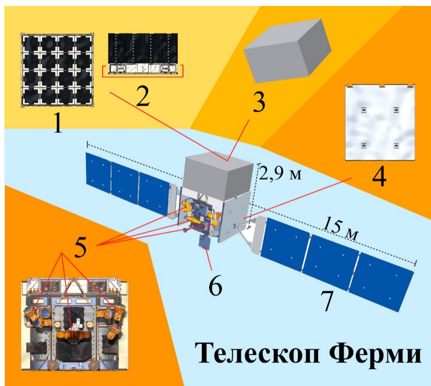
Рисунок 2 – Схематичное изображение приборов телескопа Ферми
