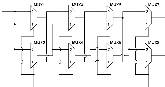
Рисунок 1 – Схема физически неклонлируемой функции типа арбитр на базе цепочки из мультиплексоров.
