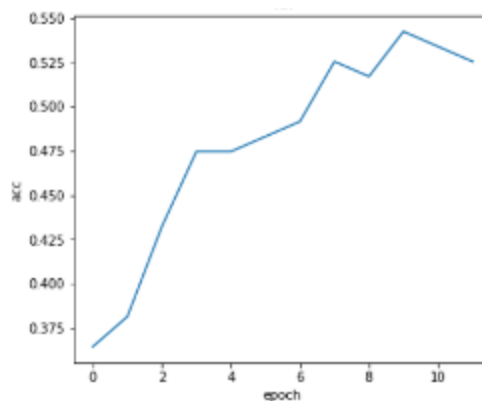
Рисунок 50 – Точность EfficientNet_V2_L с заморозкой промежуточных слоев
