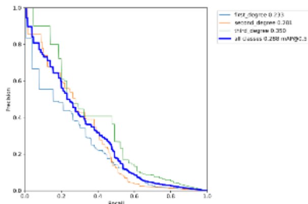
Рисунок 128 – Зависимость Precision от Recall модели Yolov5x(640x640)
