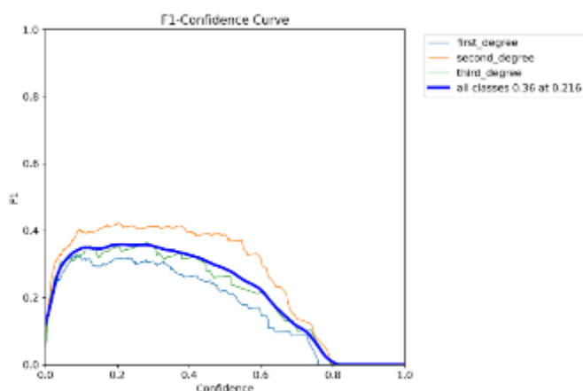
Рисунок 133 – Зависимость F1 score от уверенности модели Yolov5m(640x640)
