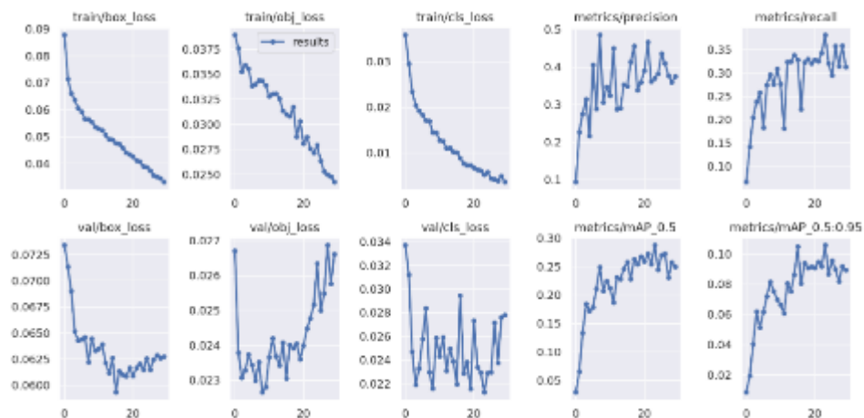
Рисунок 126 – Ошибки и точности модели Yolov5x(640x640)
