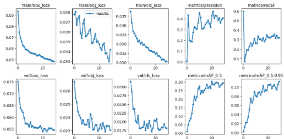
Рисунок 114 – Ошибки и точности модели YOLOv5s(640x640)
