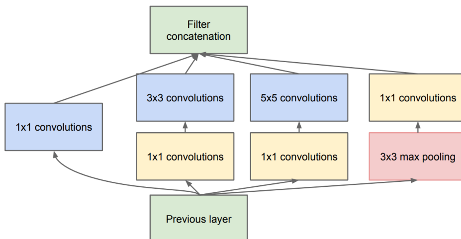
Рисунок 3 – Блок Inception с уменьшением размерности
