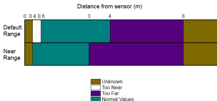
Рисунок 2 – Схема диапазонов Kinect
