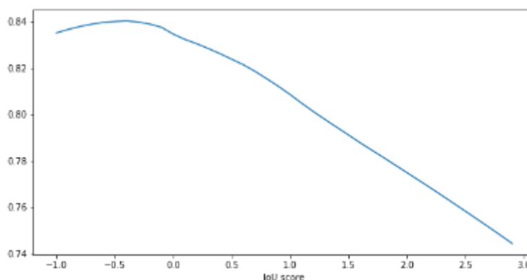
Рисунок 72 – График зависимости IoU от порога UNET(resnet18)
