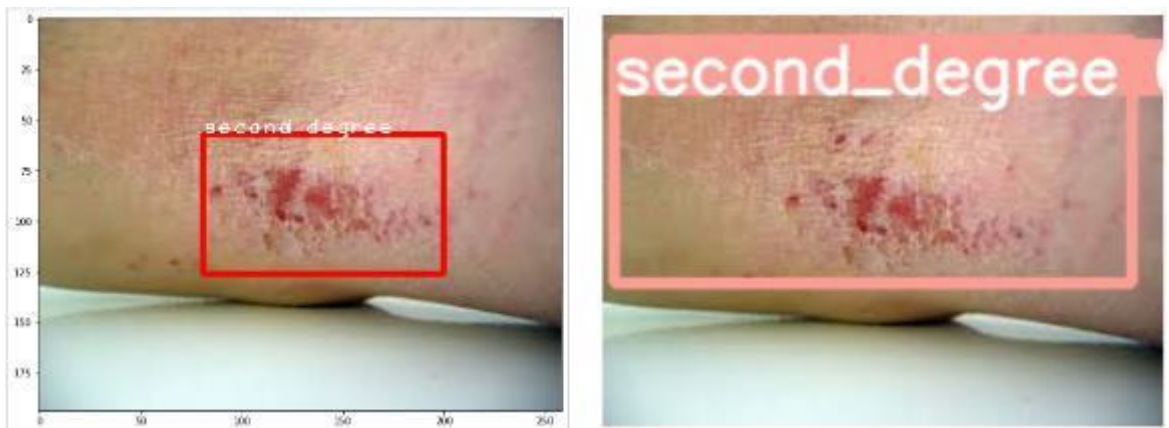
Рисунок 130 – Результаты Yolov5x(640x640)
