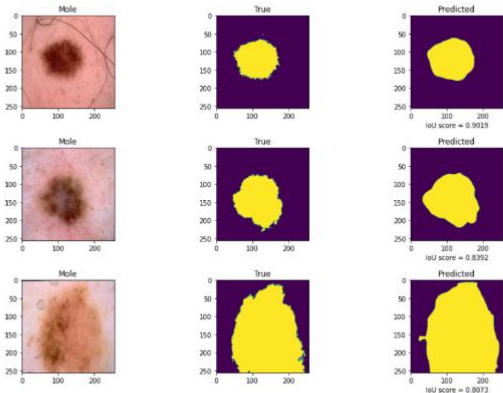
Рисунок 93 – Результаты PSPNet
