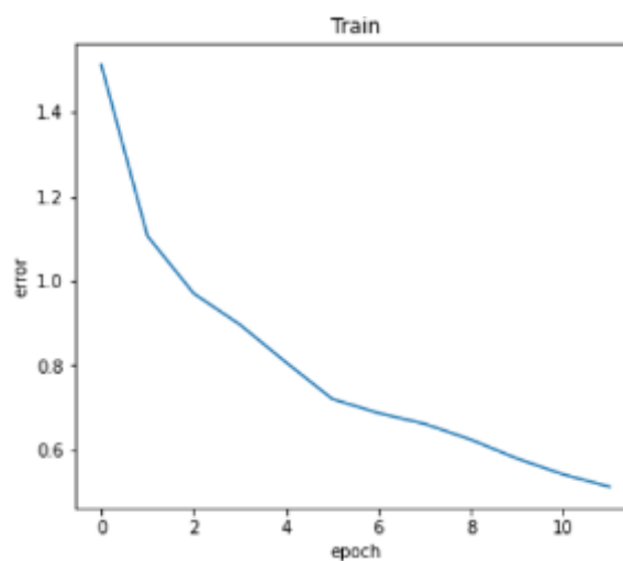
Рисунок 44 – Ошибка EfficientNet_V2_L
