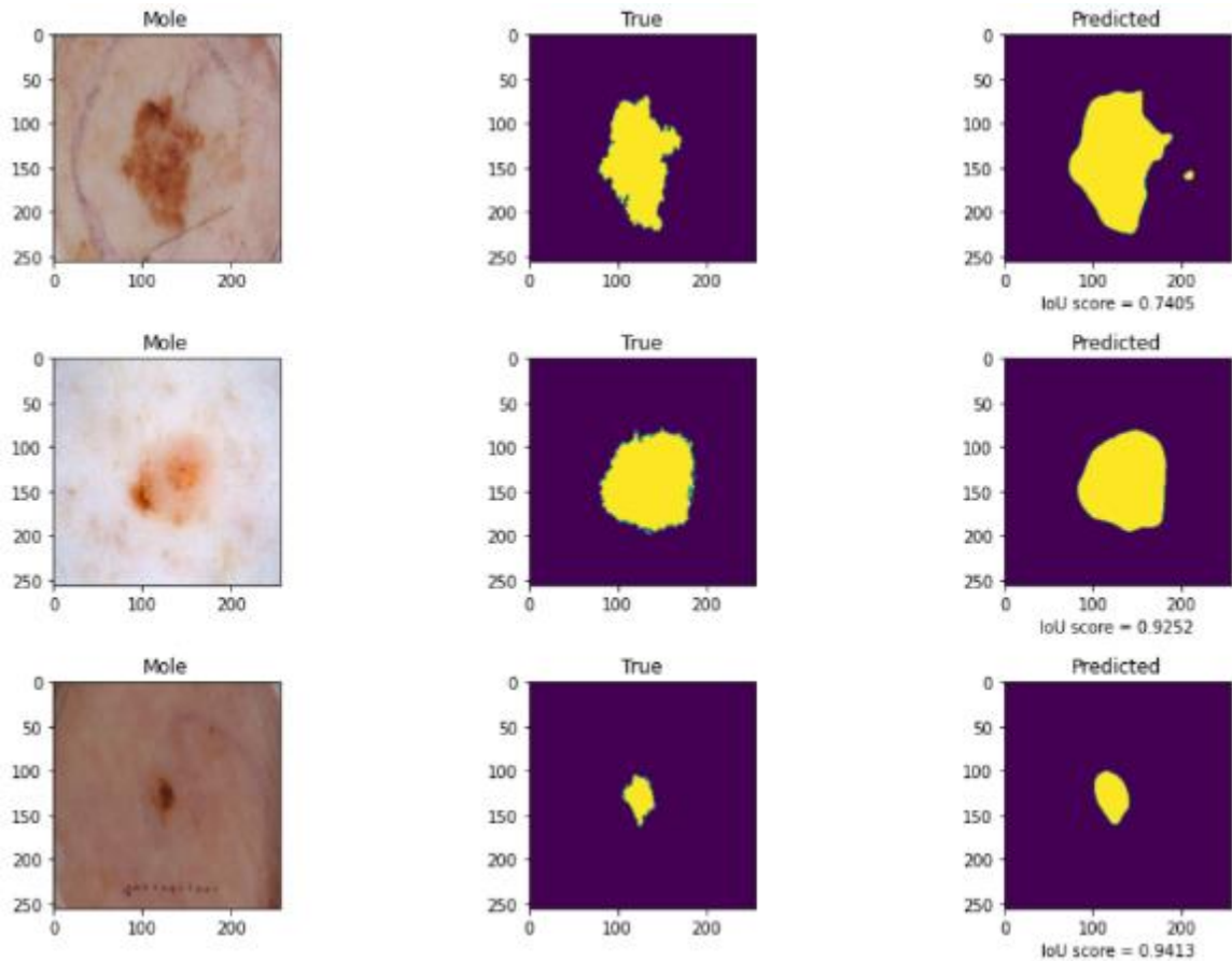
Рисунок 74 – Результаты UNET(resnet18)
