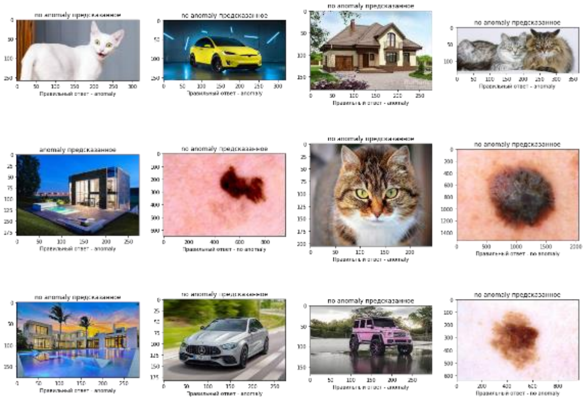
Рисунок 7 – Результаты autoencoder
