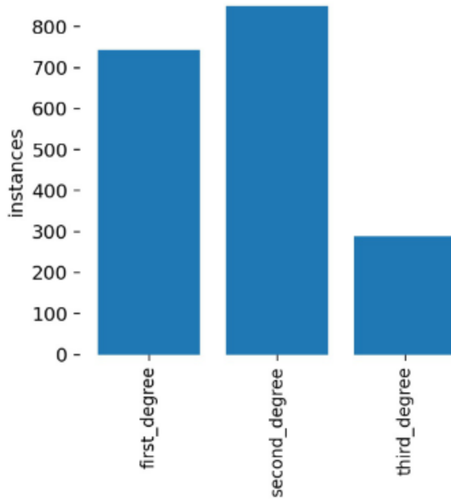
Рисунок 112 – Распределение данных
