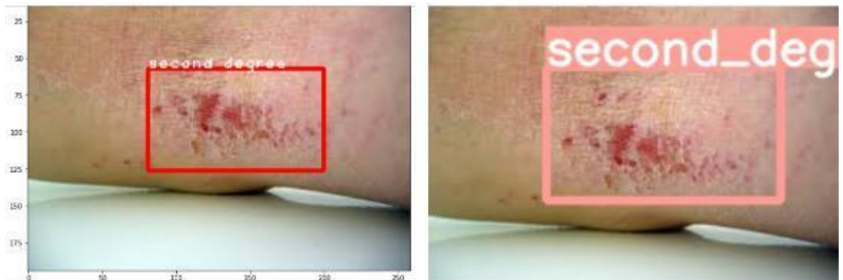
Рисунок 124 – Результаты Yolov5x(256x256)
