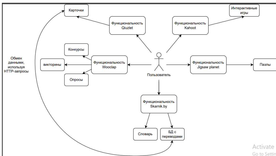
Рисунок 9 – Структура приложения
