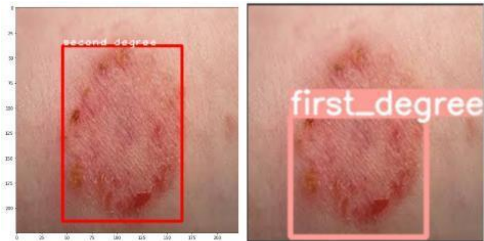
Рисунок 118 – Результаты Yolov5s(640x640)
