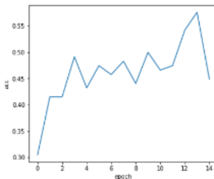
Рисунок 33 – Точность WIDE_RESNET50_2
