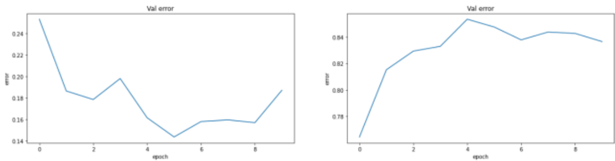
Рисунок 76 – Результаты UNET(resnet101)
