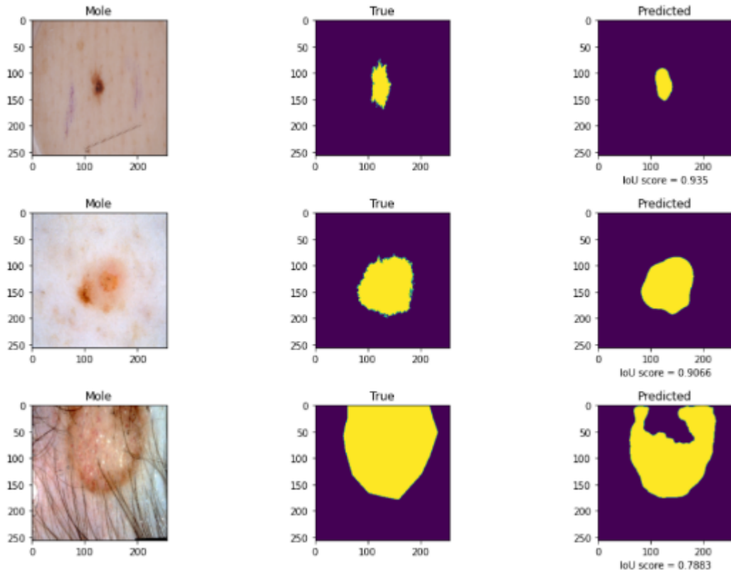
Рисунок 79 – Результаты UNET(resnet101)
