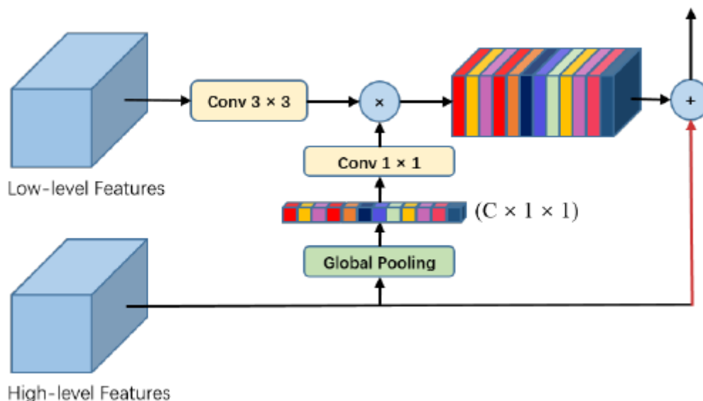
Рисунок 96 – Архитектура GAU
