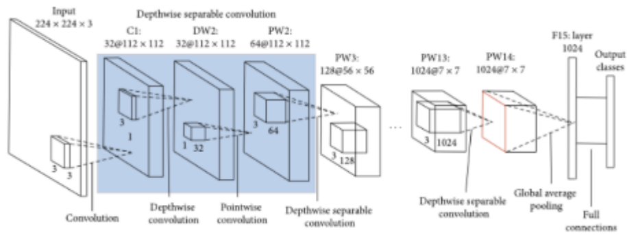
Рисунок 54 – Архитектура MOBILENET
