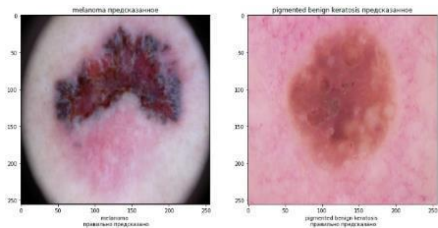
Рисунок 57 – Результаты MOBILENET
