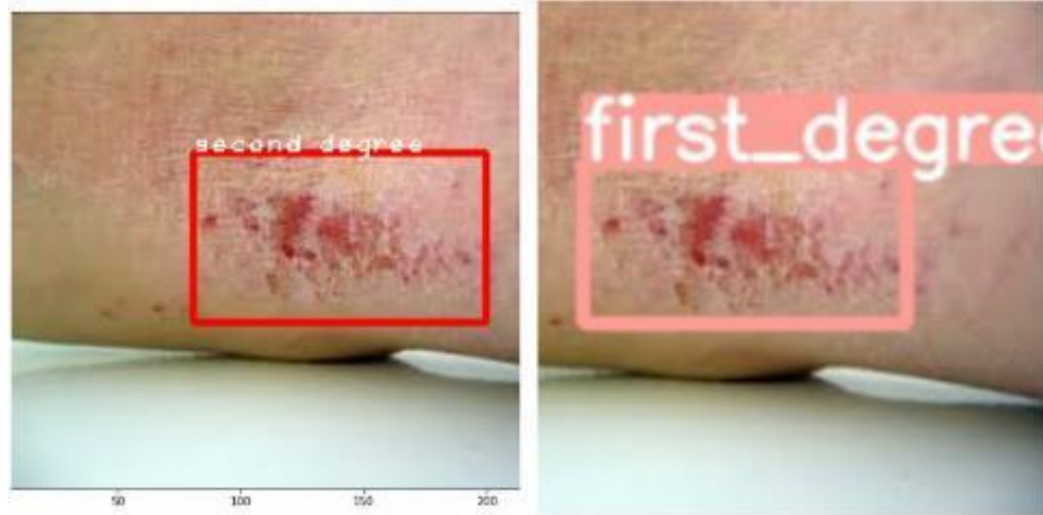
Рисунок 117 – Результаты Yolov5s(640x640)
