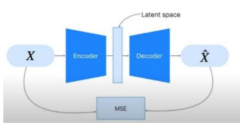
Рисунок 2 – Архитектура автоэнкодера
