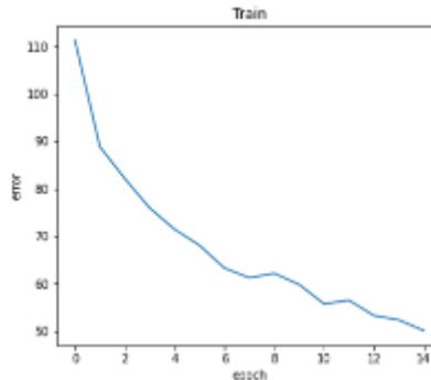
Рисунок 32 – Ошибка WIDE_RESNET50_2
