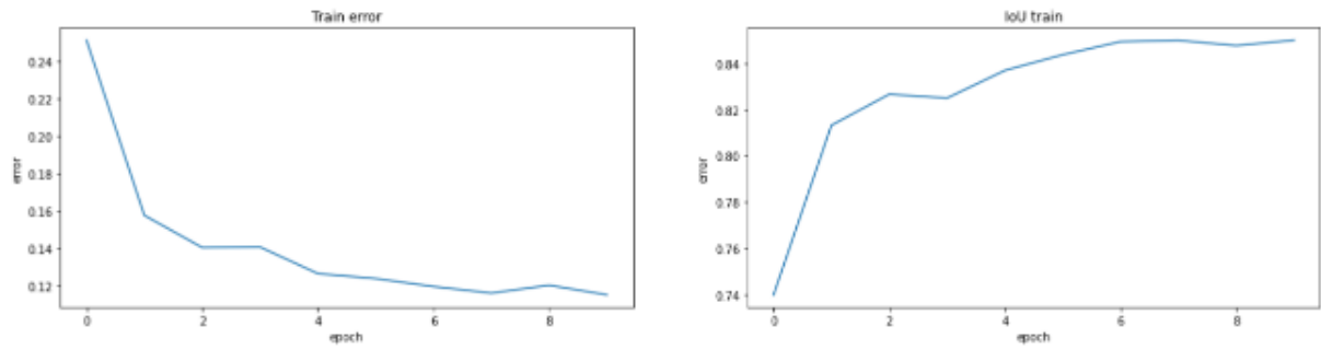
Рисунок 75 – Результаты UNET(resnet101)
