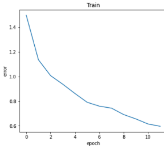
Рисунок 54 – Ошибка MOBILENET
