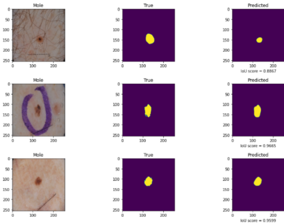
Рисунок 101 – Результаты PAN
