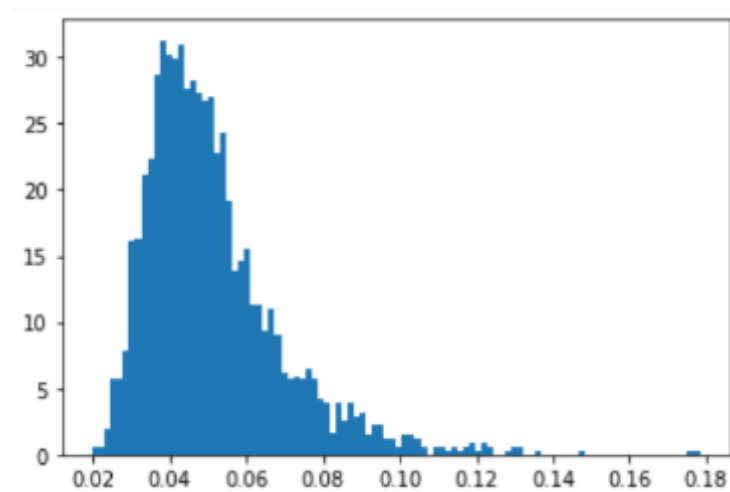
Рисунок 12 – Гистограмма разностей
