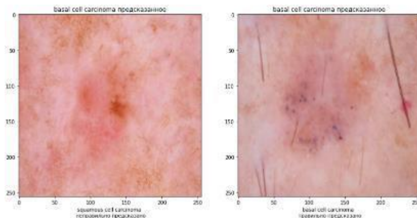
Рисунок 47 – Результаты EfficientNet_V2_L
