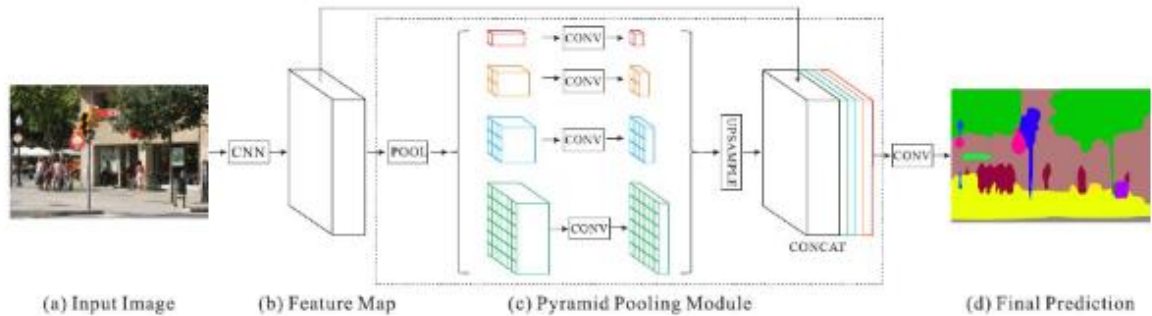
Рисунок 88 – Архитектура PSPNet
