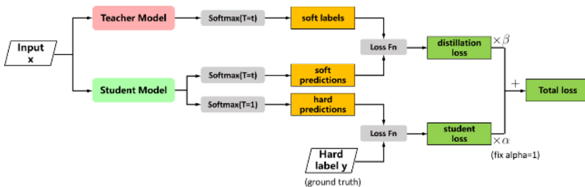
Рисунок 59 – Архитектура дистилляции
