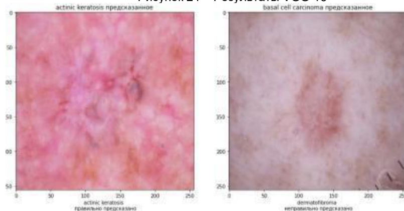
Рисунок 25 – Результаты VGG-16
