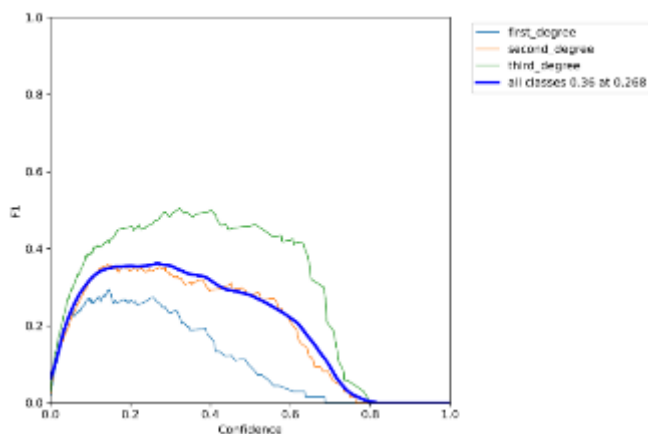
Рисунок 115 – Зависимость F1 score от уверенности модели YOLOv5s(640x640)
