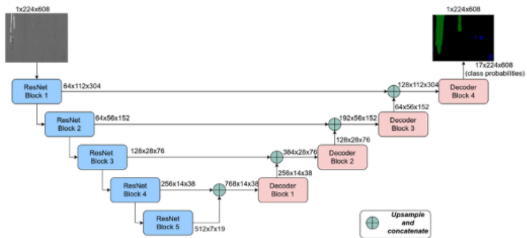
Рисунок 69 – Архитектура модели UNET
