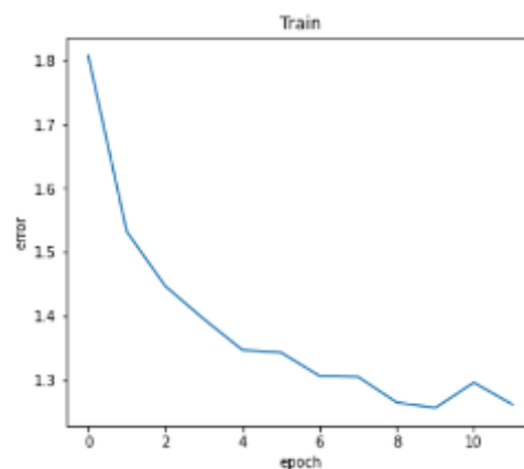
Рисунок 49 – Ошибка EfficientNet_V2_L с заморозкой промежуточных слоев
