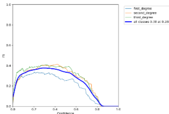
Рисунок 121 – Зависимость F1 score от уверенности модели Yolov5x(256x256)
