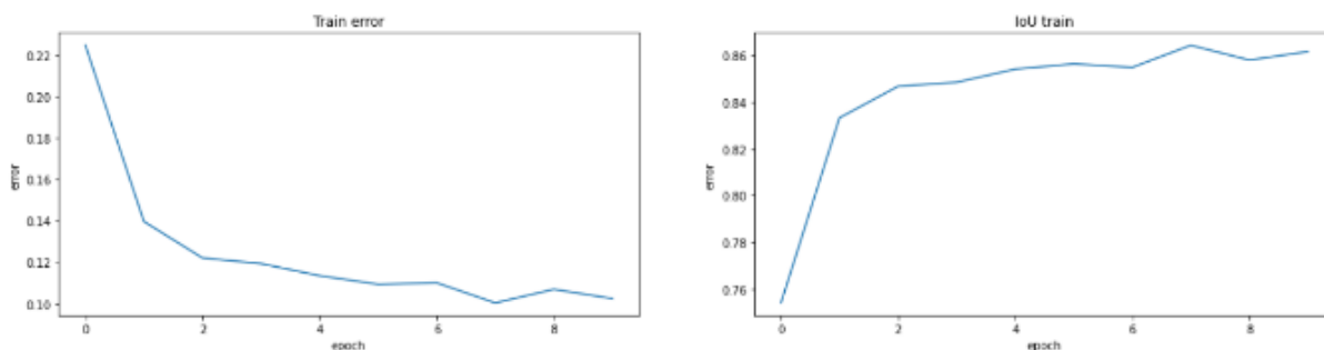
Рисунок 70 – Ошибка UNET(resnet18) на тренировочных данных и IoU
