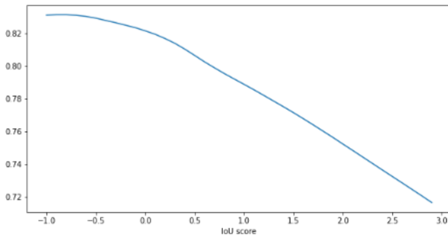
Рисунок 77 – График зависимости IoU от порога UNET(resnet101)
