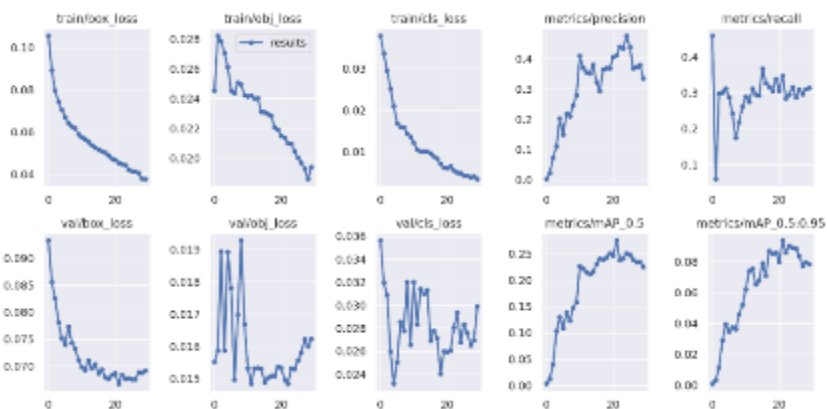
Рисунок 120 – Ошибки и точности модели Yolov5x(256x256)
