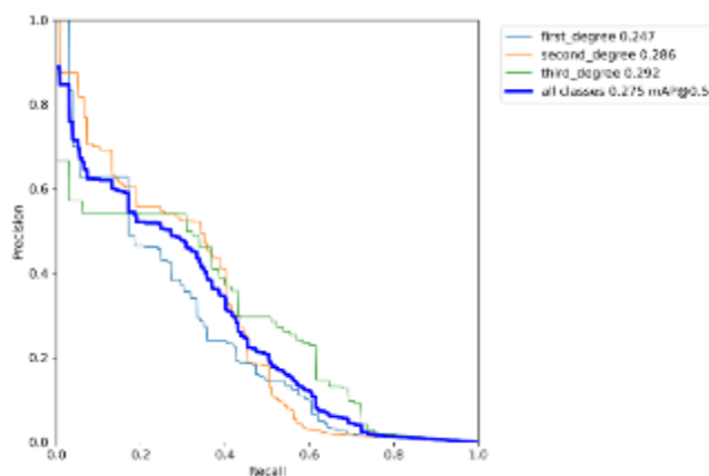
Рисунок 122 – Зависимость Precision от Recall модели Yolov5x(256x256)
