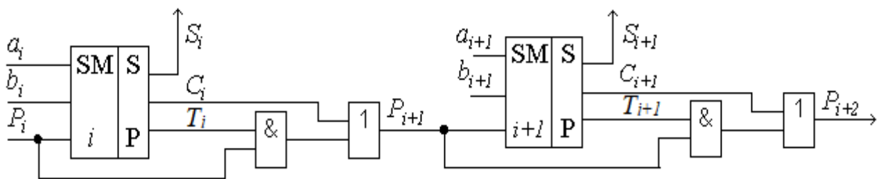
Рисунок 2 - Структурная схема параллельного сумматора со сквозным переносом
