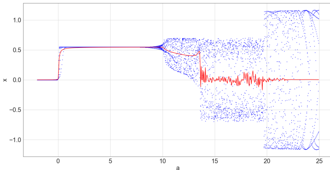
Рисунок 2 - Бифуркационная диаграмма при управлении по \alpha -параметру
