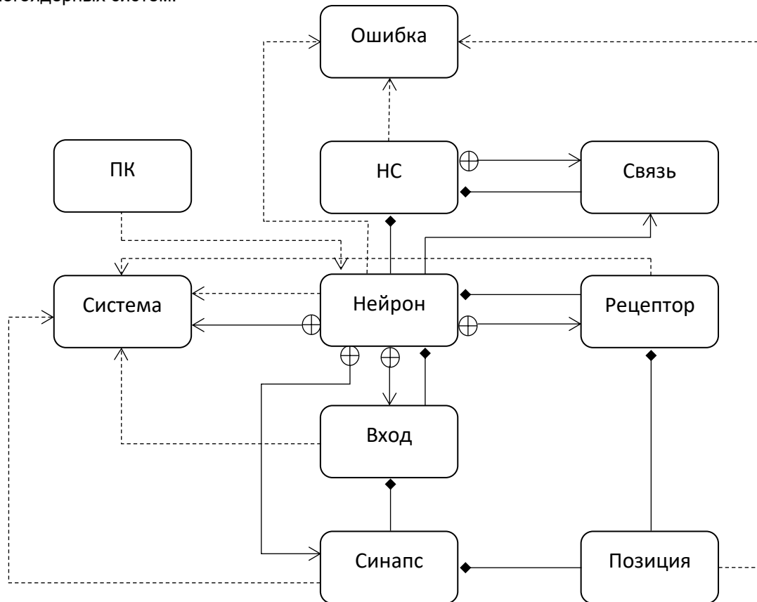
Рисунок 3 – Схема работы библиотеки прецизионной ИНС
