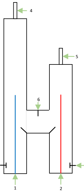
Рис. 1 – схема устройства «Электролизёр»
