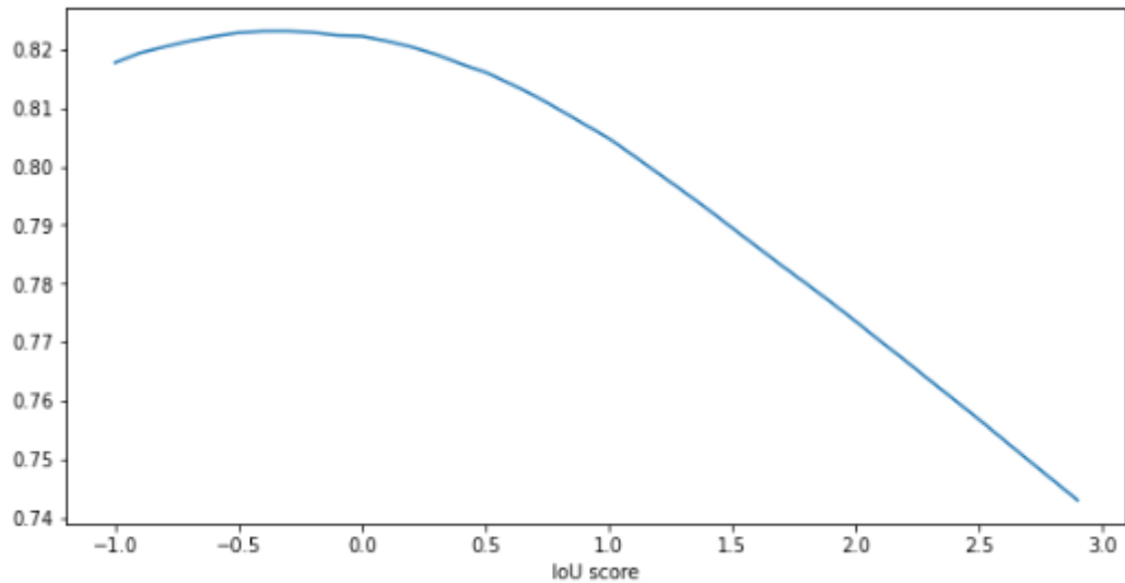
Рисунок 91 – График зависимости IoU от порога PSPNet
