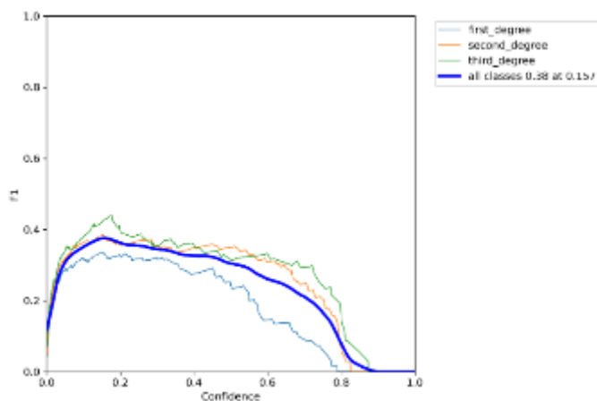
Рисунок 127 – Зависимость F1 score от уверенности модели Yolov5x(640x640)
