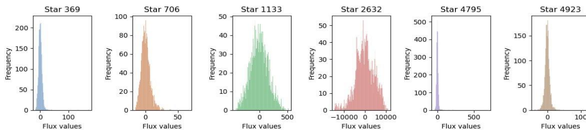
Рисунок 2 – графики распределения интенсивности светового потока
