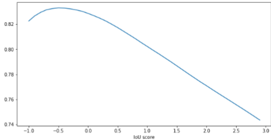
Рисунок 104 – График зависимости IoU от порога дистиллированной модели
