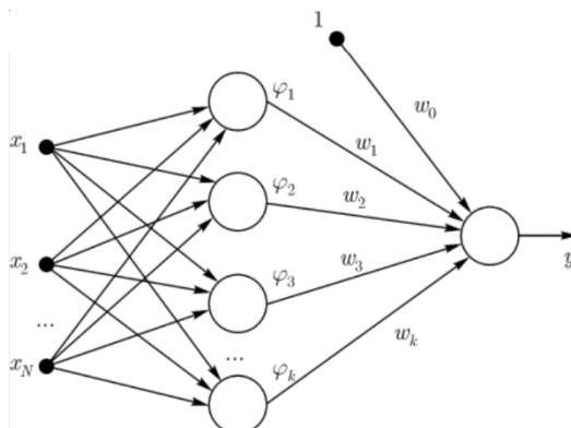
Рисунок 1 – радиально-базисная сеть [1]
