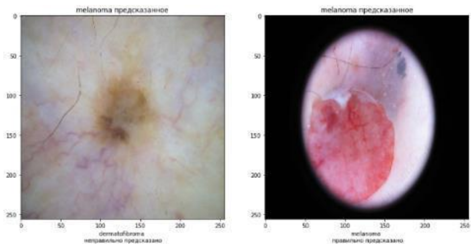
Рисунок 58 – Результаты MOBILENET
