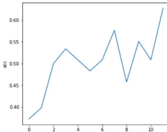
Рисунок 55 – Точность MOBILENET
