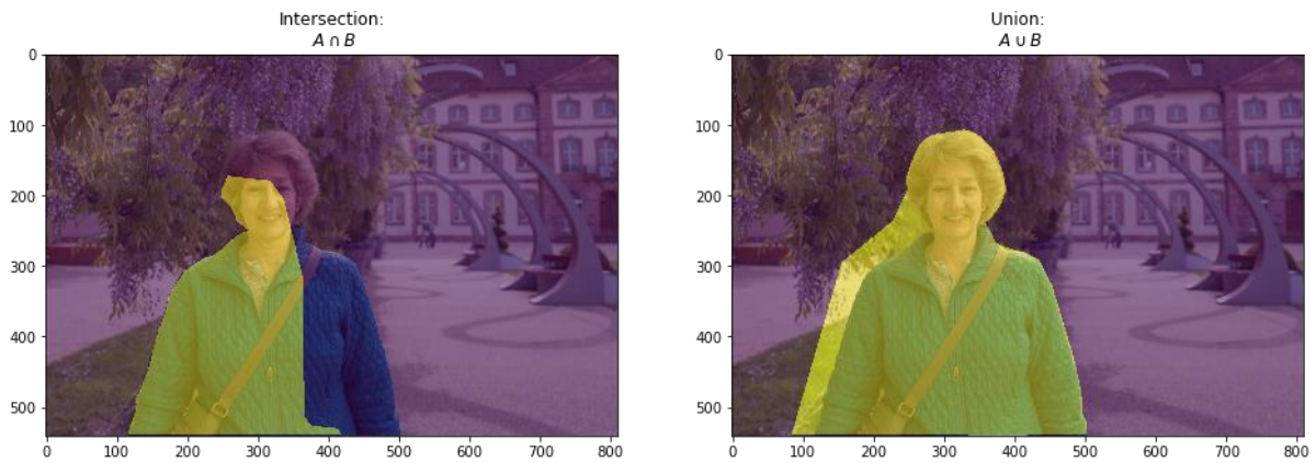
Рисунок 68 – Операции над множествами
