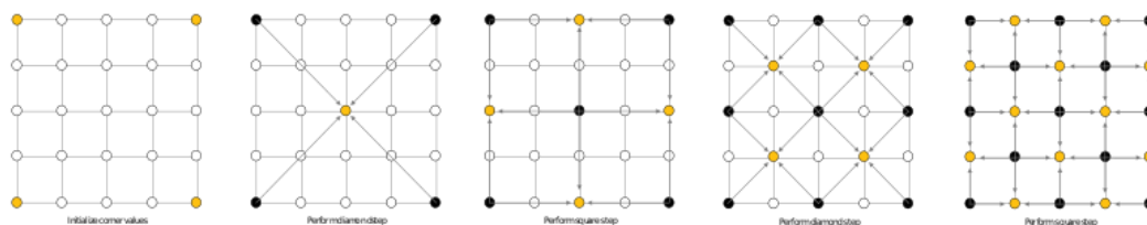
Рисунок 1 – алгоритм Diamond-Square[2]
