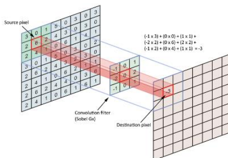
Рисунок 1 – Свертка изображения
