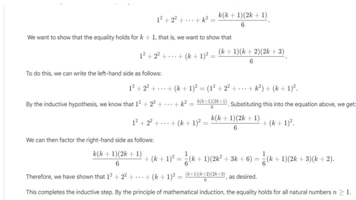
Рисунок 1 – Ответ ChatGPT
