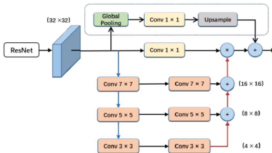
Рисунок 95 – Архитектура FPA
