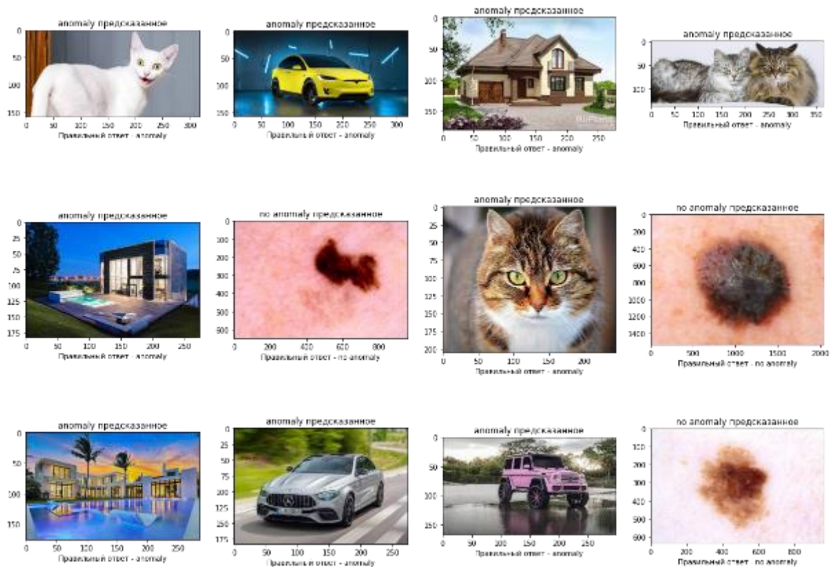
Рисунок 13 – Результаты autoencoder
