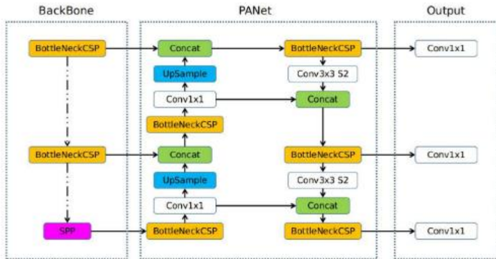
Рисунок 109 – Архитектура YOLOv5
