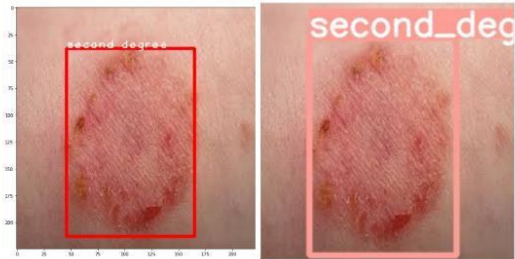
Рисунок 123 – Результаты Yolov5x(256x256)
