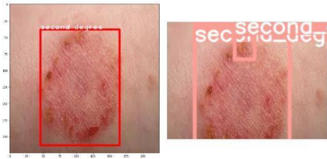
Рисунок 129 – Результаты Yolov5x(640x640)
