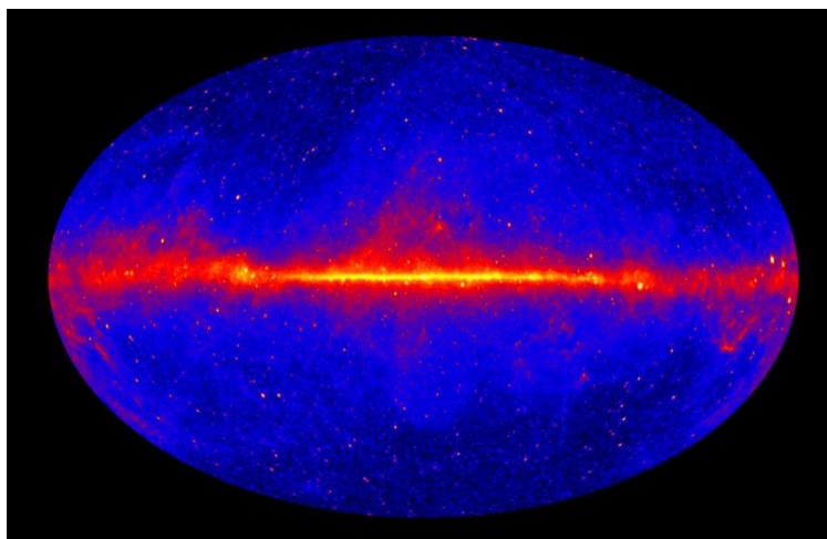
Рисунок 1 – Изображение, полученное FGST
