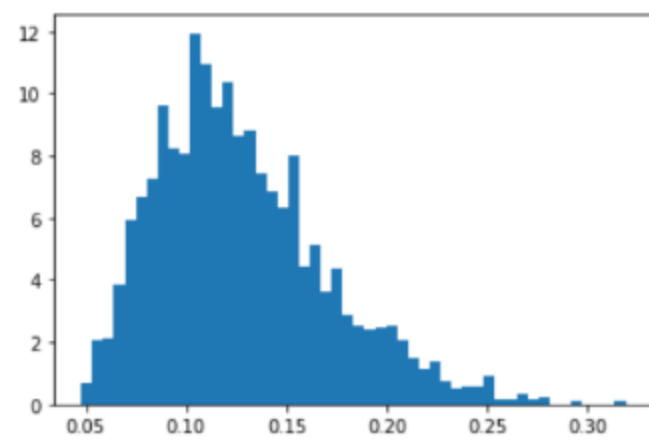
Рисунок 6 – Гистограмма разностей
