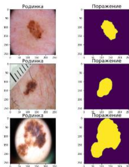
Рисунок 65 – Данные
