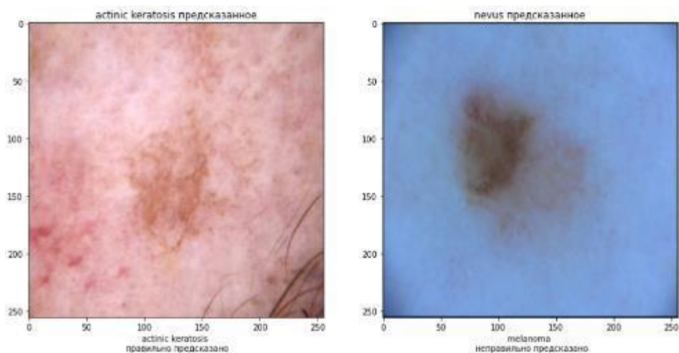
Рисунок 35 – Результаты WIDE_RESNET50_2
