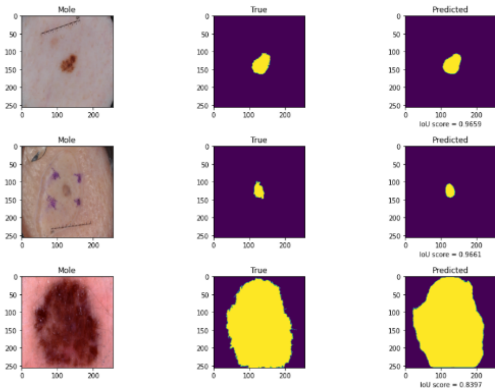
Рисунок 87 – Результаты LinkNet
