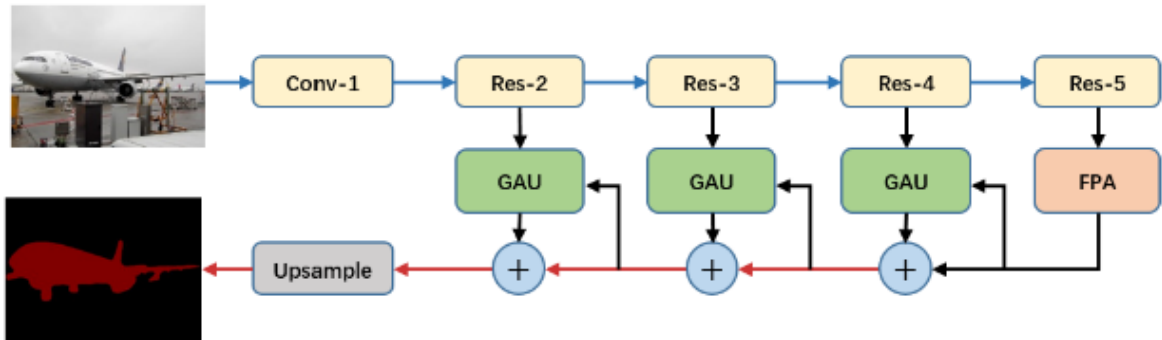
Рисунок 94 – Архитектура PAN
