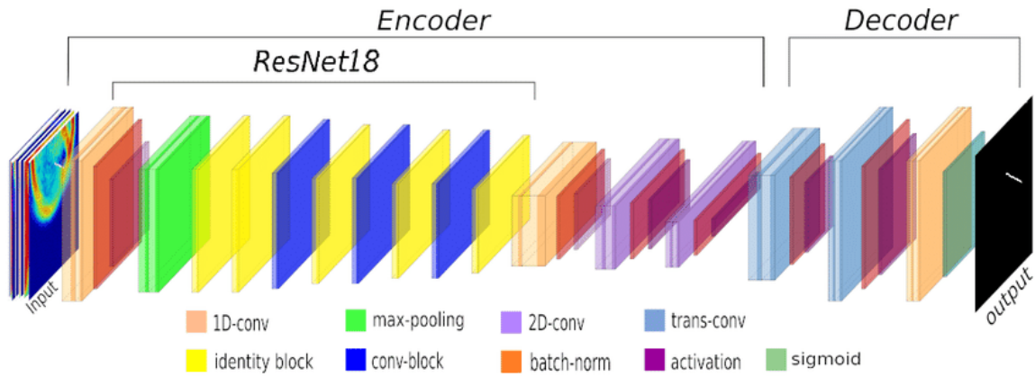
Рисунок 4 – Архитектура resnet18
