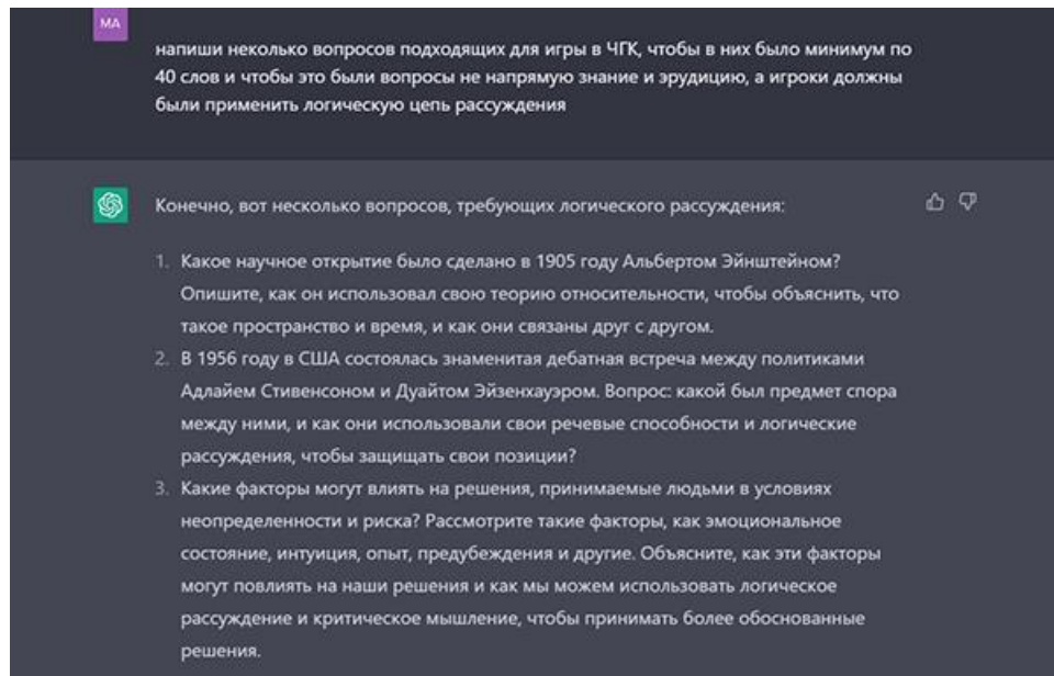
Рисунок 1 – Генерация вопросов
