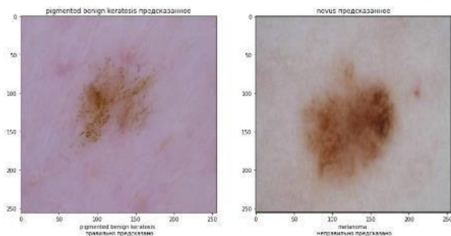
Рисунок 36 – Результаты WIDE_RESNET50_2
