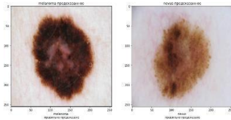
Рисунок 48 – Результаты EfficientNet_V2_L
