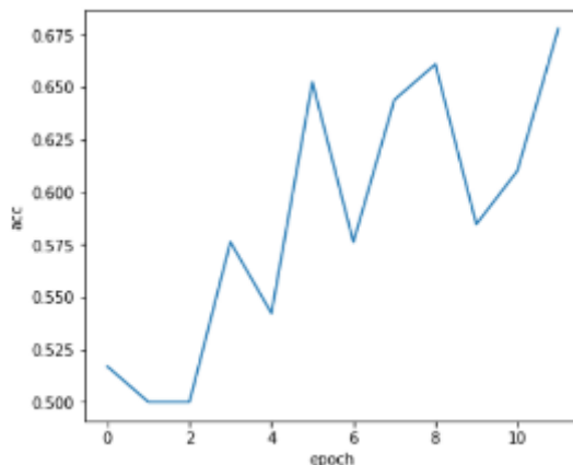
Рисунок 45 – Точность EfficientNet_V2_L
