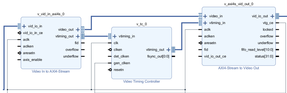
Рисунок 3 – Каскад конвертирования сигнала
