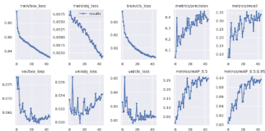
Рисунок 132 – Ошибки и точности модели Yolov5m(640x640)
