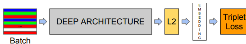
Рисунок 2 – Архитектура встроенной сети FaceNet
