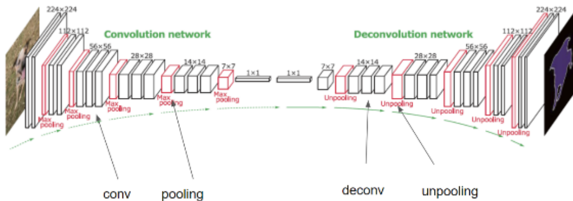
Рисунок 66 – Общая архитектура сегментационных моделей
