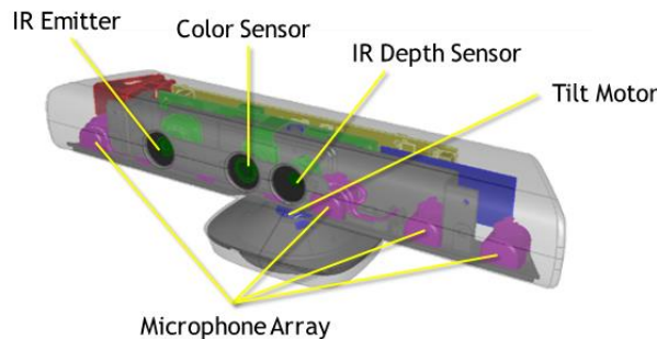
Рисунок 1 – Устройство Microsoft Kinect v1.0
