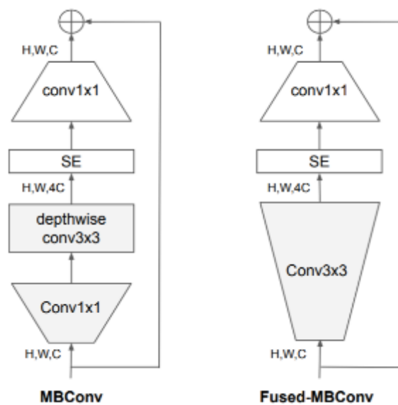
Рисунок 43 – Блоки MBConv и Fused-MBConv
