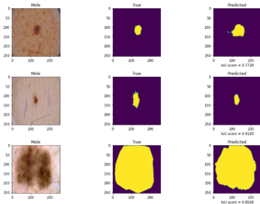
Рисунок 106 – Результаты дистиллированной модели
