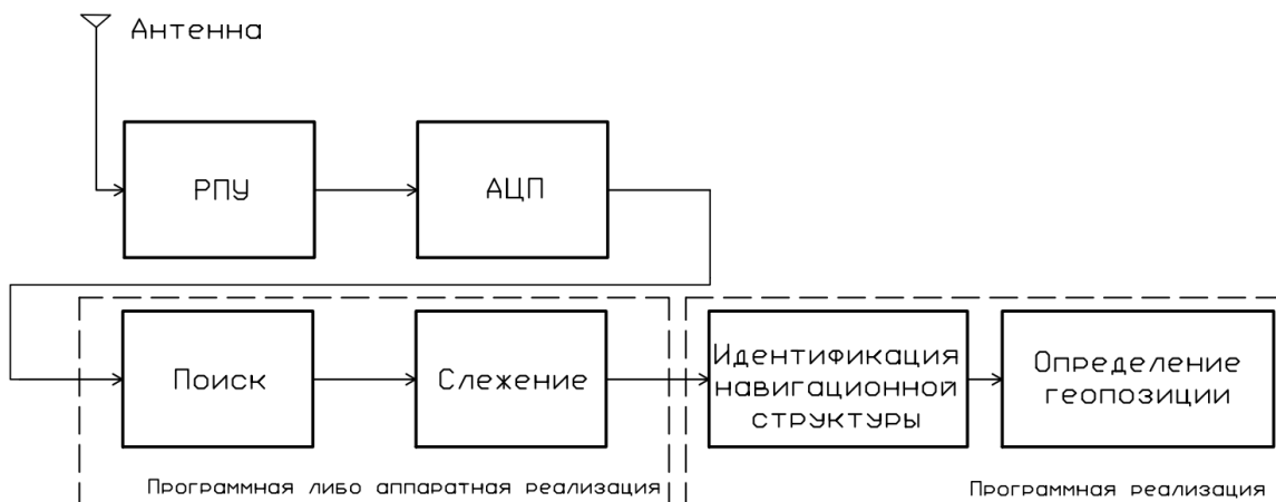
Рисунок 1 – Структура навигационного приемного устройства
