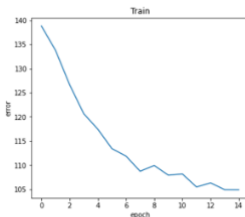
Рисунок 26 – Ошибка VGG-16 без заморозки промежуточных слоев на тренировочных данных
