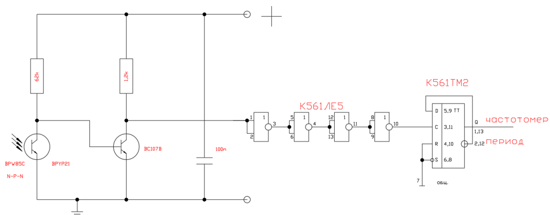
Рисунок 2 – Электрическая схема установки
