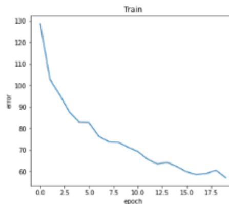
Рисунок 21 – Ошибка VGG-16 на тренировочных данных
