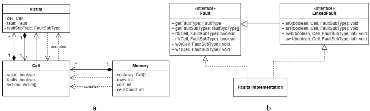
Рисунок 2 – Диаграмма классов программного средства
