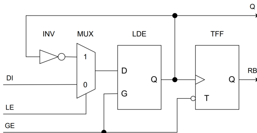
Рисунок 1 – Схема базового элемента комбинированного генератора
