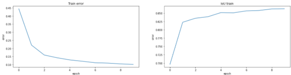
Рисунок 83 – Ошибка LinkNet на тренировочных данных и IoU
