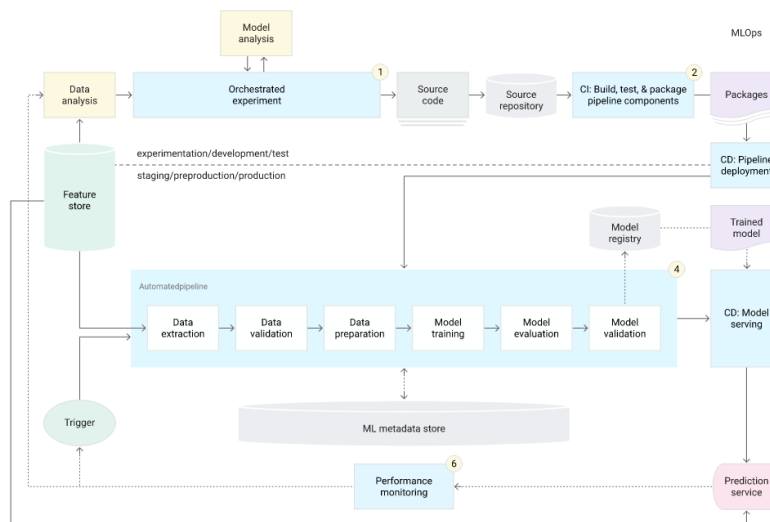
Рисунок 1 – автоматизация всего ML пайплайна с использованием continuous integration и continuous delivery.
