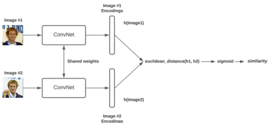
Рисунок 1 – Архитектура нейронной сети
