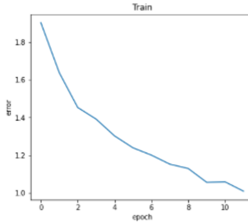
Рисунок 37 – Ошибка WIDE_RESNET50_2 с длинный fc
