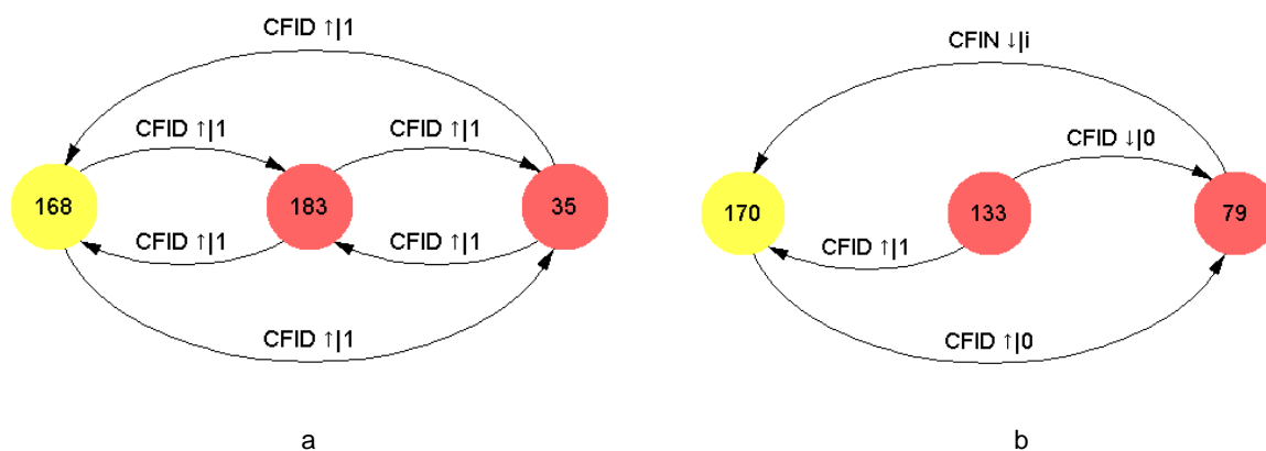
Рисунок 1 – Графы неисправностей взаимного влияния для трёх ячеек
