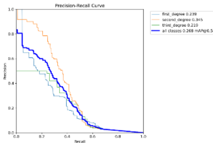
Рисунок 134 – Зависимость Precision от Recall модели Yolov5m(640x640)
