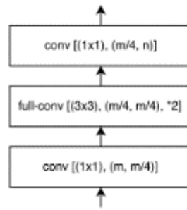
Рисунок 82 – Архитектура decoder блока
