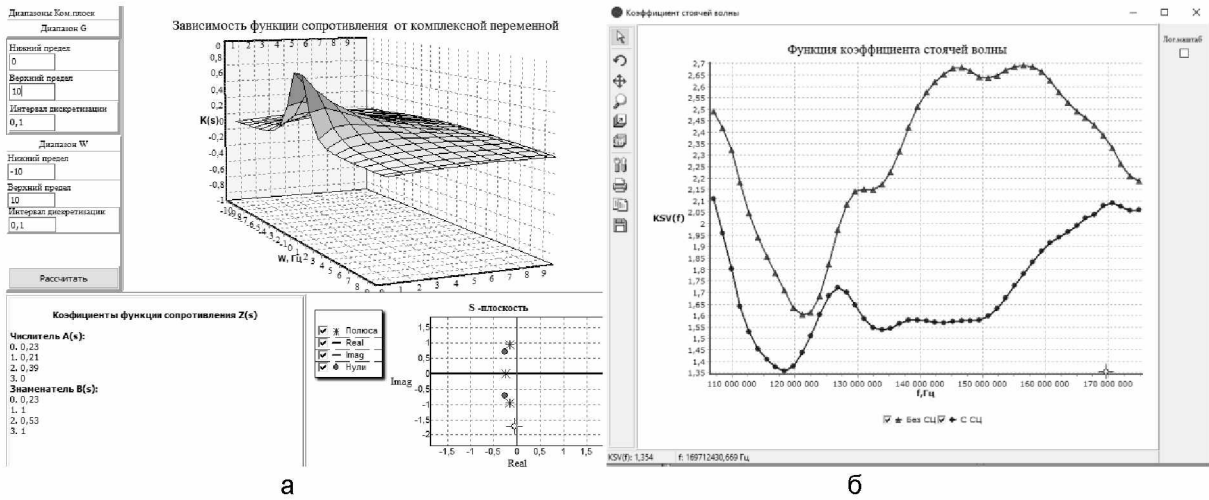
Рисунок 4 – Подпрограмма отображения функции сопротивления ШСУ на комплексной плоскости (а) и зависимость КСВ от частоты с синтезированным ШСУ и без его (б)
