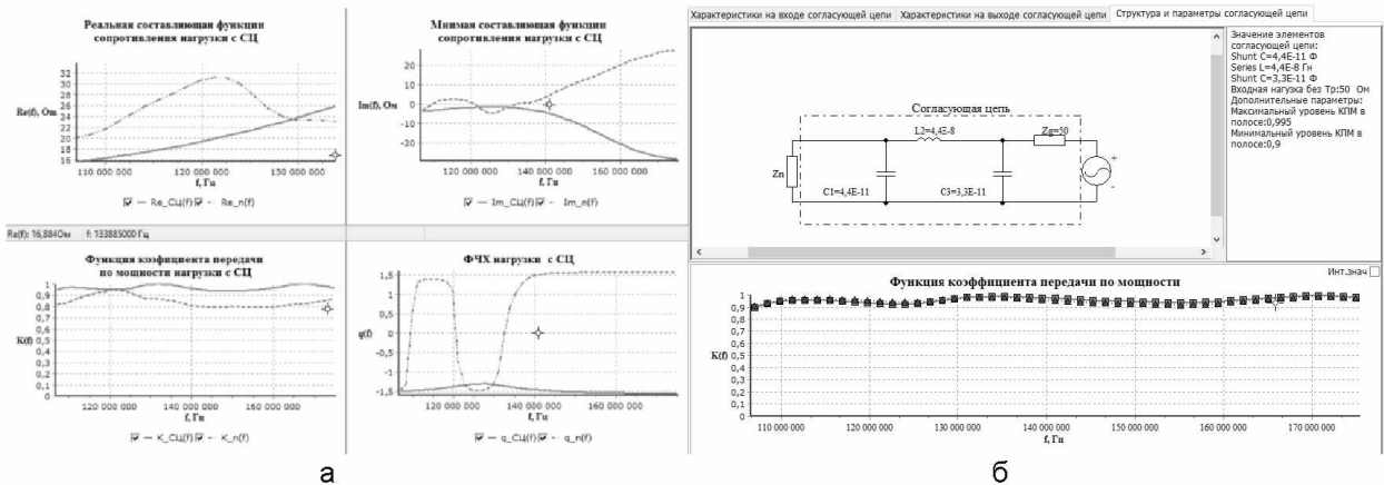
Рисунок 3 – Результаты математического моделирования (а) и синтеза ШСУ с элементами СЦ приведенные под ряд номиналов (б)
