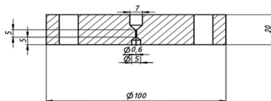
Рис. 2. Геометрия рабочего канала Fig. 2. Geometry of the working channel
