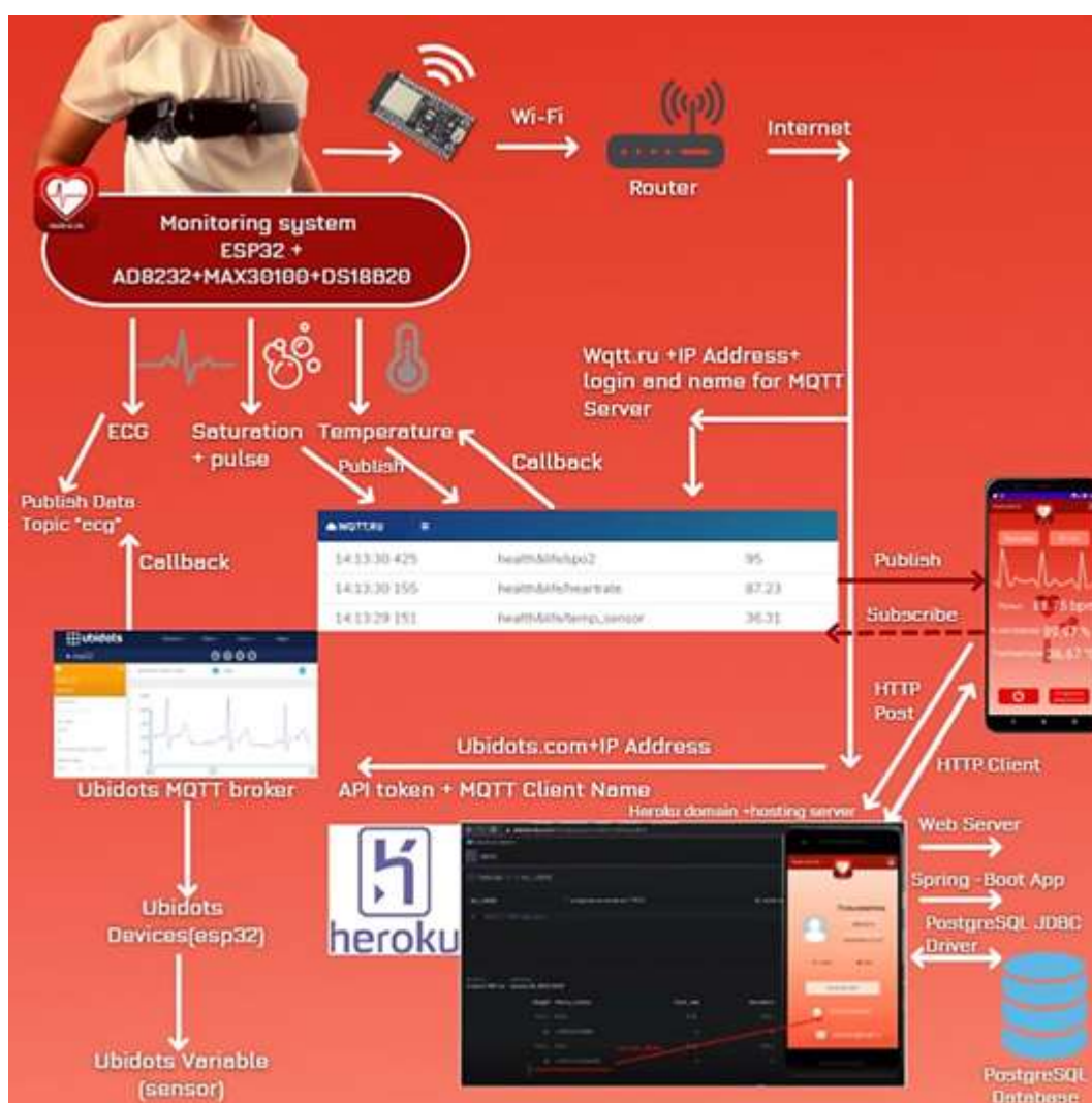
Рисунок 8 – Схема работы с данными
