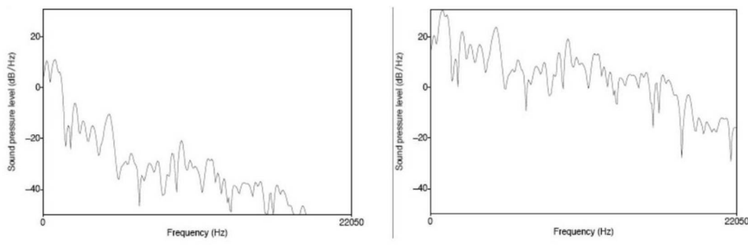
Рисунок 3 – Предварительное усиление высоких частот (Pre-emphasis) в обработке речи
