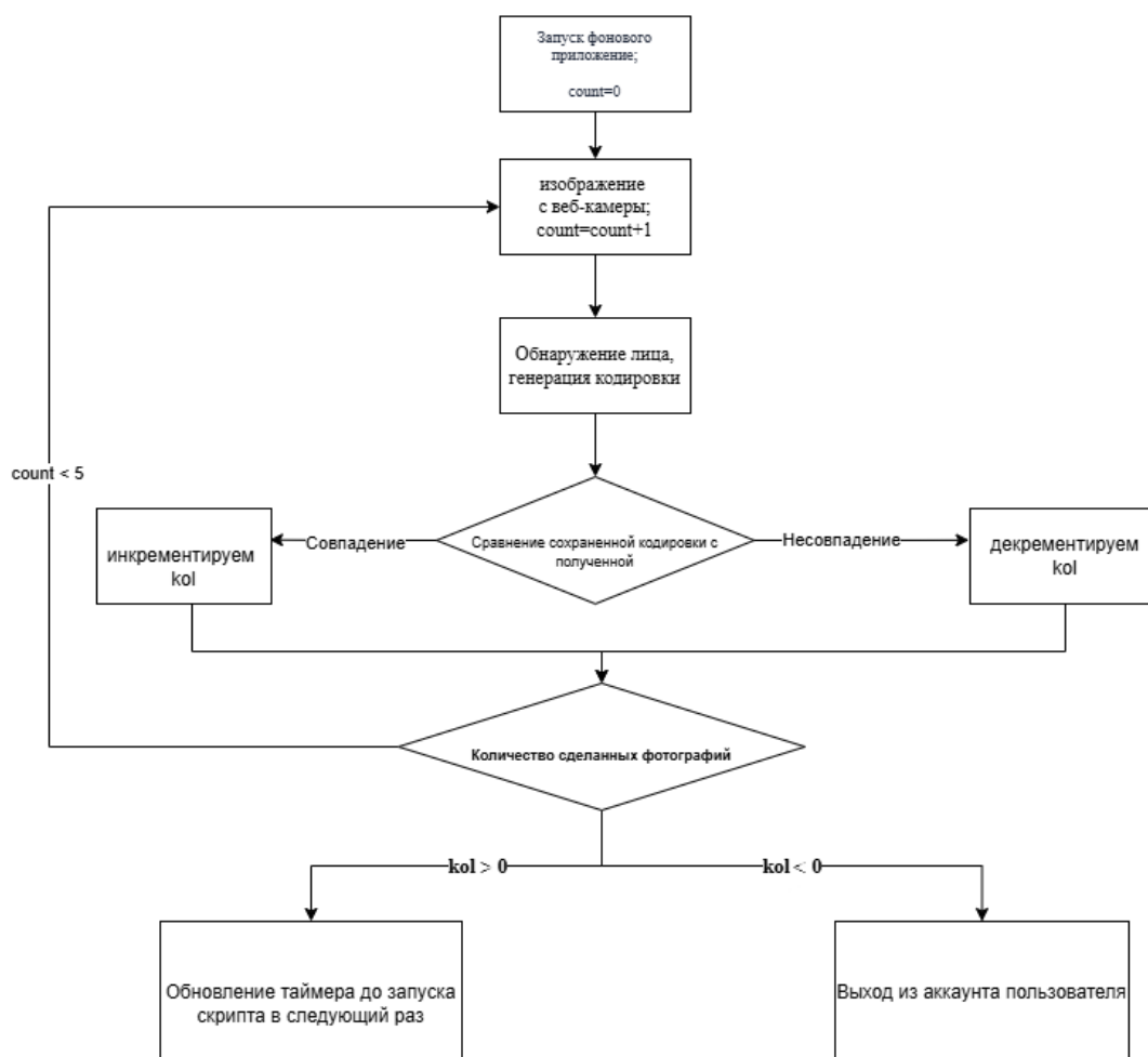
Рисунок 1. Алгоритм работы фоновой службы автоматического сканирования пользователей
