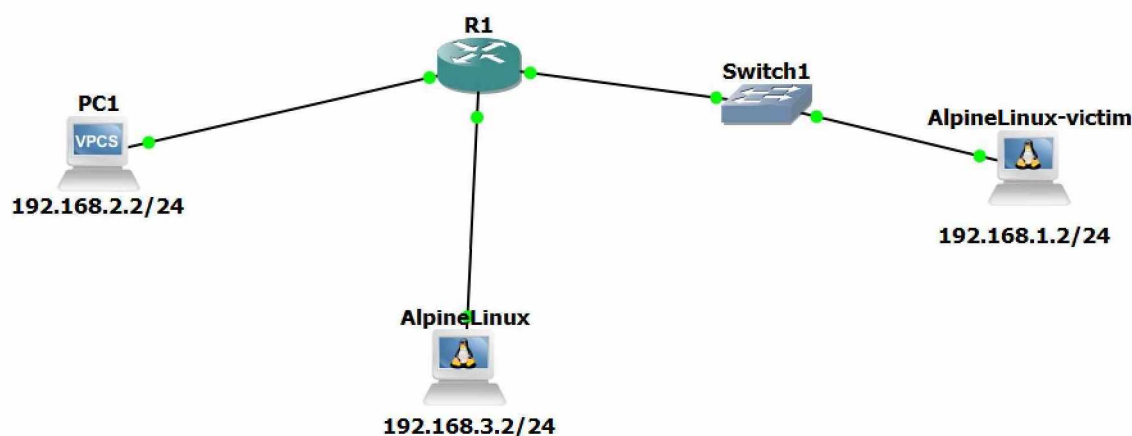
Рисунок 2 – Схема виртуальной лаборатории, построенной с использованием симулятора GNS3
