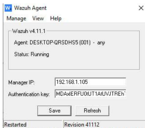
Рисунок 1 – Главное меню программы Wazuh Agent
