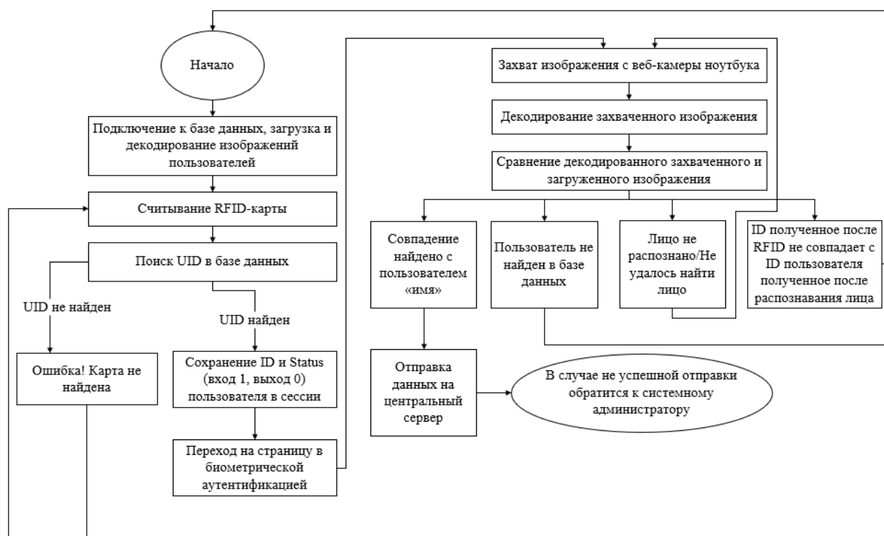
Рисунок 1 – Блок-схема функционирования СКУД
