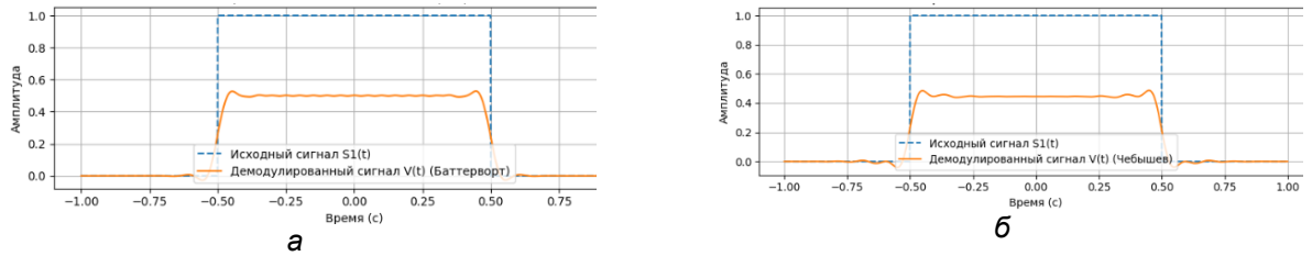
а – вид демодулированного сигнала с фильтром Баттерворта; б – вид демодулированного сигнала с фильтром Чебышева;
