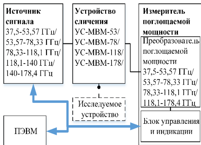
Рисунок 1 – Обобщенная структурная схема эталона
