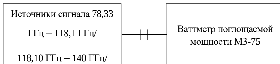
Рисунок 2 – Структурная схема измерений уровня мощности источников сигнала
