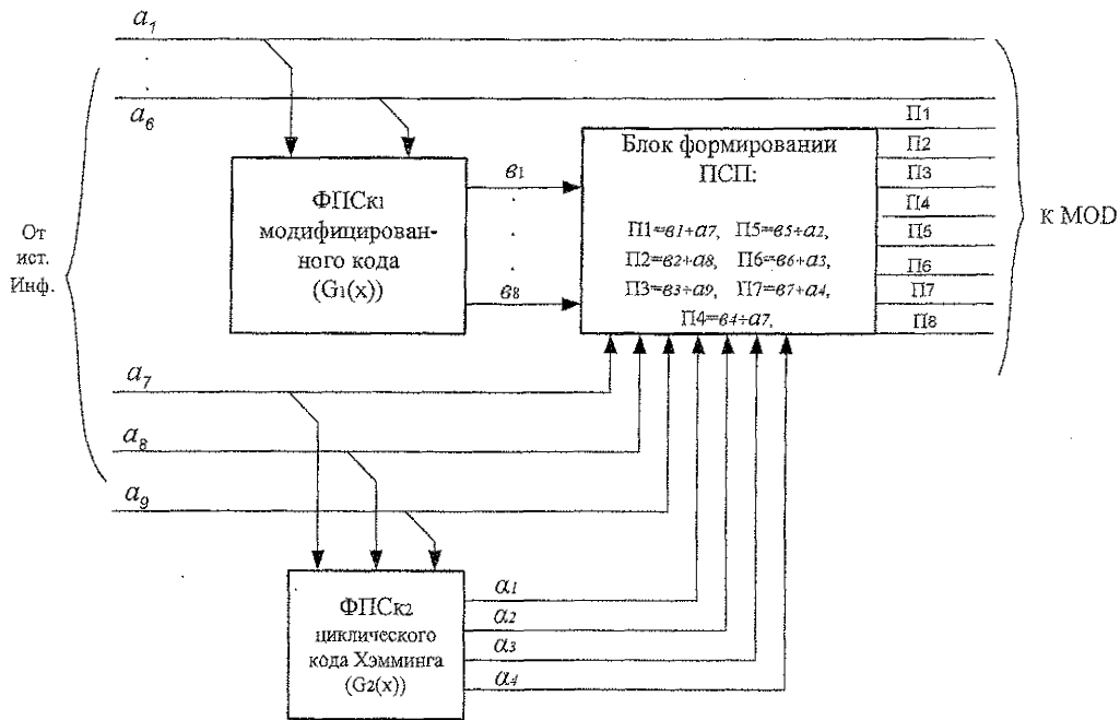
Рис. 2. Кодировующие устройство модифицированного ЦК: ФПСк 1 и ФПСк 2 – формирователи проверочных символов соответственно первого и второго каналов кодирования; ПСП – псевдослучайная последовательность
