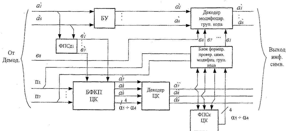
Рис. 3. Декодировующие устройство модифицированного ЦК: БУ – буферное устройство, БФКП – блок формирования кодовых последовательностей, ФПСд 1 – формирователь проверочных символов декодера модифицированного группового кода
