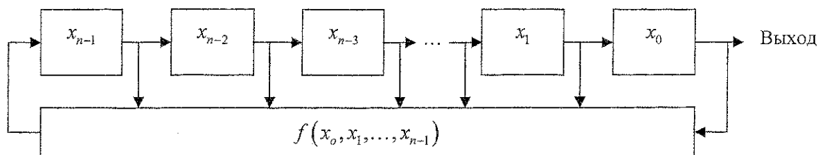
Рис. 1. Блок-схема n -уровневого регистра сдвига с обратной связью конфигурации Фибоначчи
