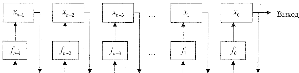
Рис. 2. Блок-схема n -уровневого регистра сдвига с обратной связью конфигурации Галуа
