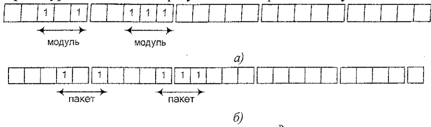
Рис. 1. Образующие вектора ошибок, t=5 : a - e^P_{обр} модульной ошибки; b - e^M_{обр} пакетной ошибки
