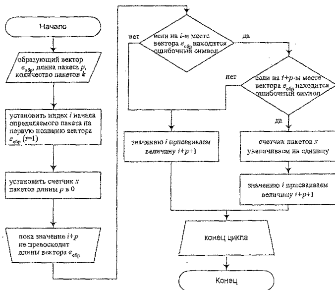
Рис. 4. Алгоритм реализации шага 2 метода генерации пакетов
