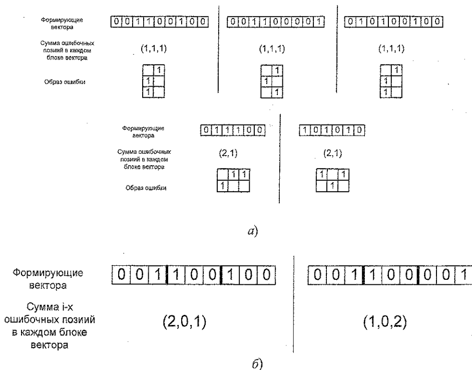
Рис. 7. Образы классов: а – совпадающие по строкам; б – совпадающие по столбцам
