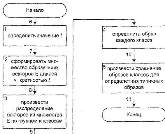
Рис. 9. Алгоритм формирования библиотеки образов ошибок кратности t
