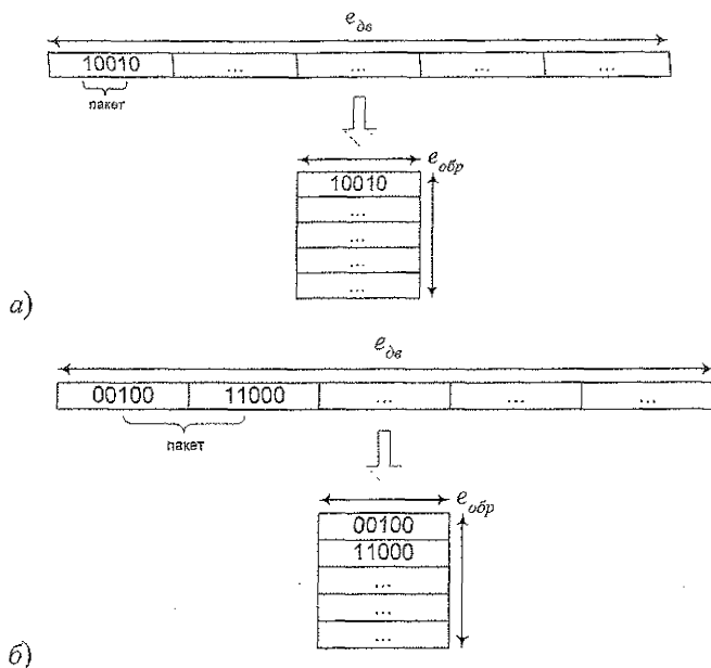
Рис. 5. Размещение пакета в образующем векторе ошибки:
