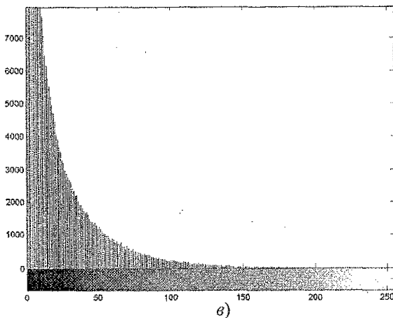
Рис. 1. Формирование контурной маски при T_L(n) = 80 и T_H(n) = 160 : а – полутоновое изображение I(n) ; б – контурное изображение I_C(n) ; в – гистограмма контурного изображения I_C(n) ; г – контурная маска M_C(n)
