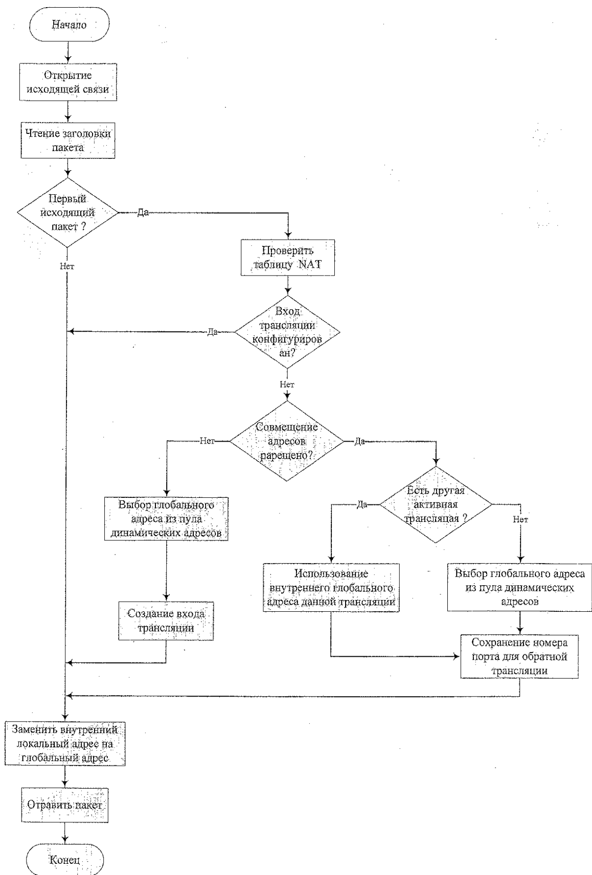
Рис. 6. Алгоритм совмещения внутренних глобальных адресов
