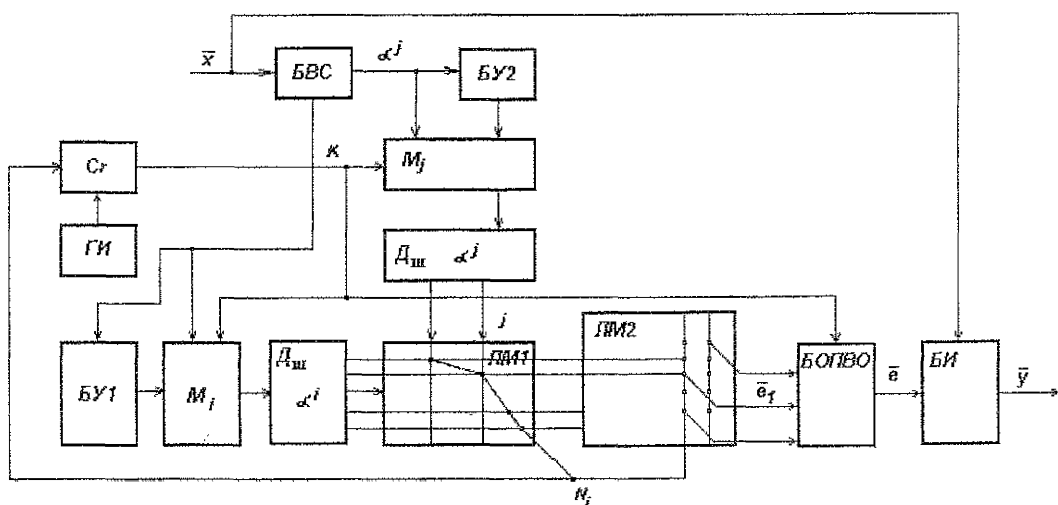
Рис. 2. Структурная схема декодера, реализующего метод циклотомического сдвига для t=3
