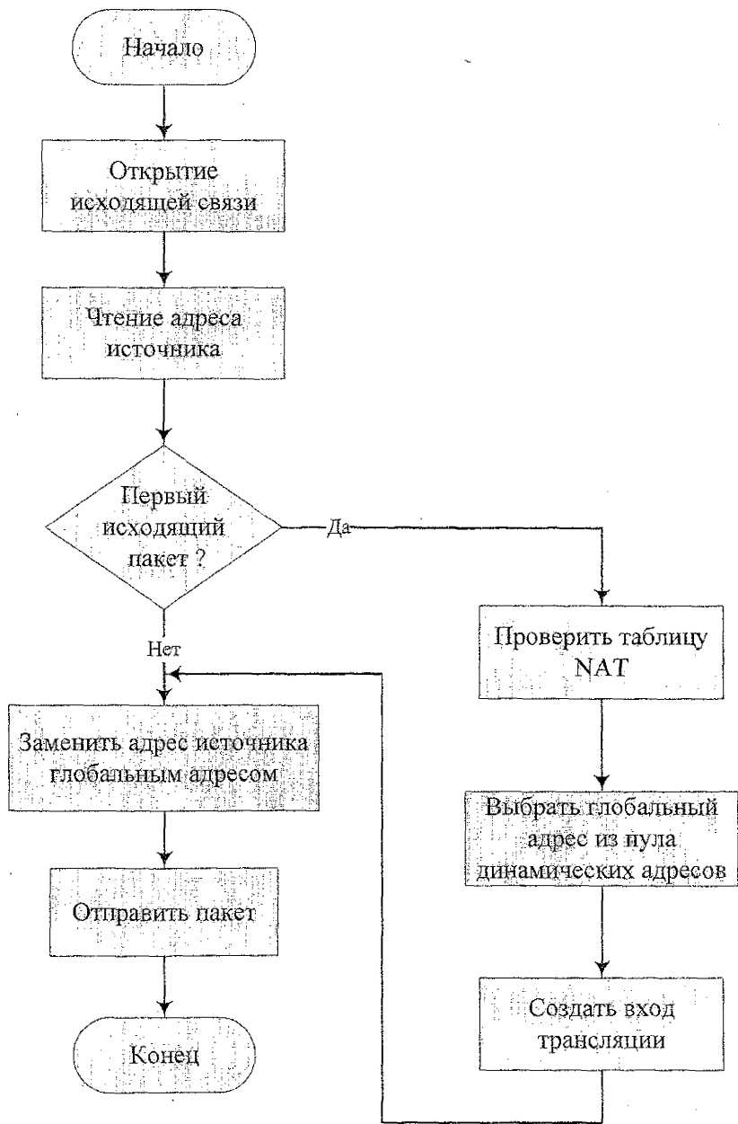
Рис. 3. Алгоритм трансляции внутреннего адреса источника динамическим методом
