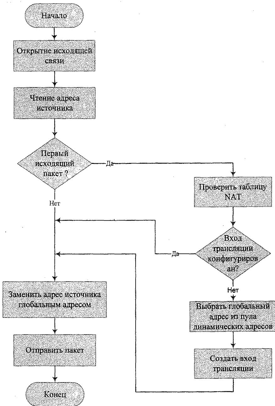
Рис. 4. Алгоритм трансляции внутреннего адреса источника смешанным методом
