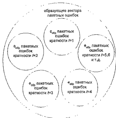
Рис. 2. Множество образующих векторов пакетных ошибок
