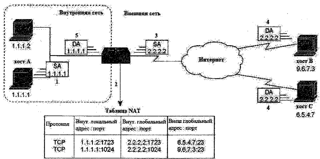
Рис. 5. Перегрузка глобальных адресов в NAT
