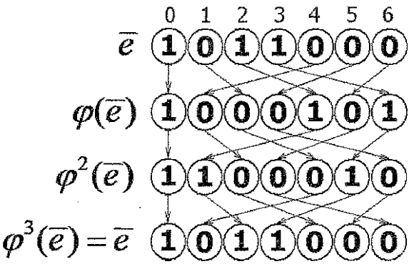
Рис. 1. Действие циклотомической подстановки \varphi и ее степеней в пространстве E_7 на вектор \overline{e} = (1011000)
