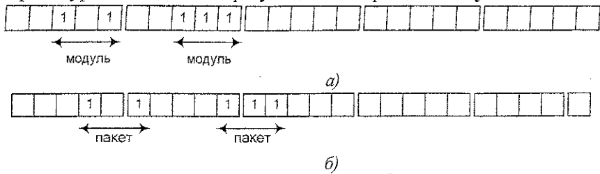
Рис. 1. Образующие вектора ошибок, t=5 : a - e^P_{обр} модульной ошибки; б - e^M_{обр} пакетной ошибки
