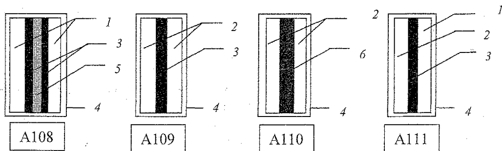
Рис. 1. Состав исследованных образцов: 1 – поролок, пропитанный водой; 2 – поролок сухой; 3 – шунгит; 4 – полиэтиленовая пленка; 5 – алюминиевая фольга, 6 – порошкообразный шунгит с добавлением воды, герметизированный полиэтиленовой пленкой
