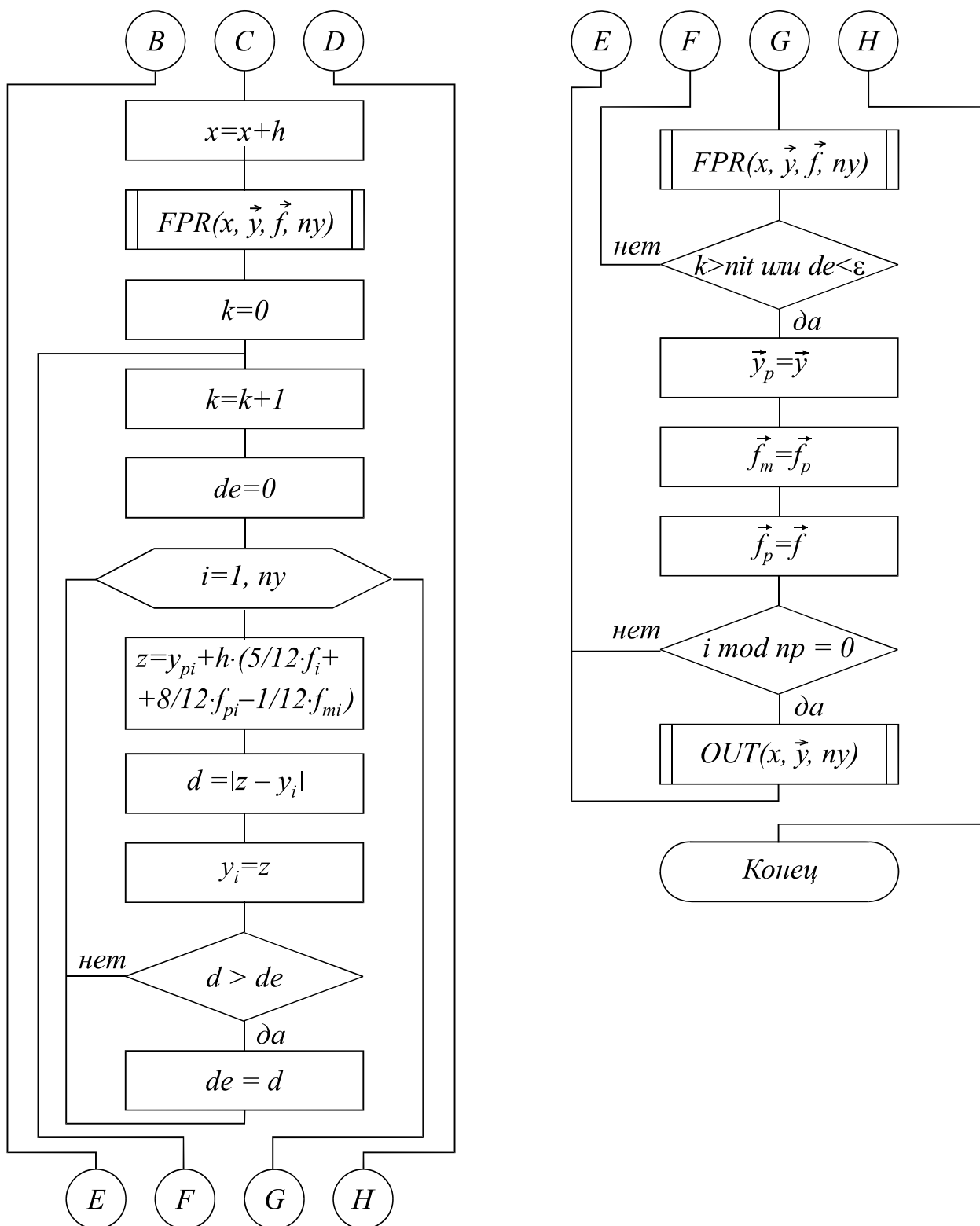
Рис. 19.4. (окончание) Схема Адамса 3-го порядка
