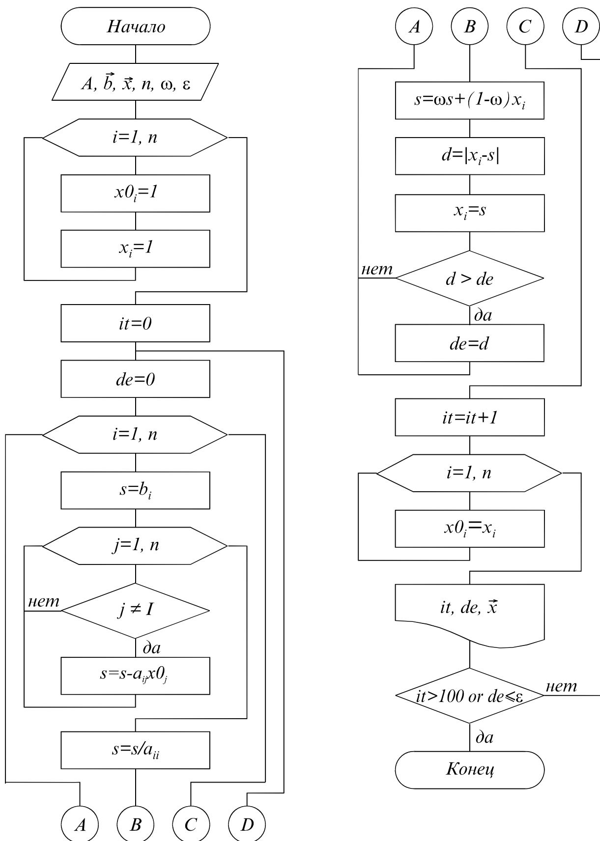
Рис. 15.3 Схема алгоритма метода простой итерации
