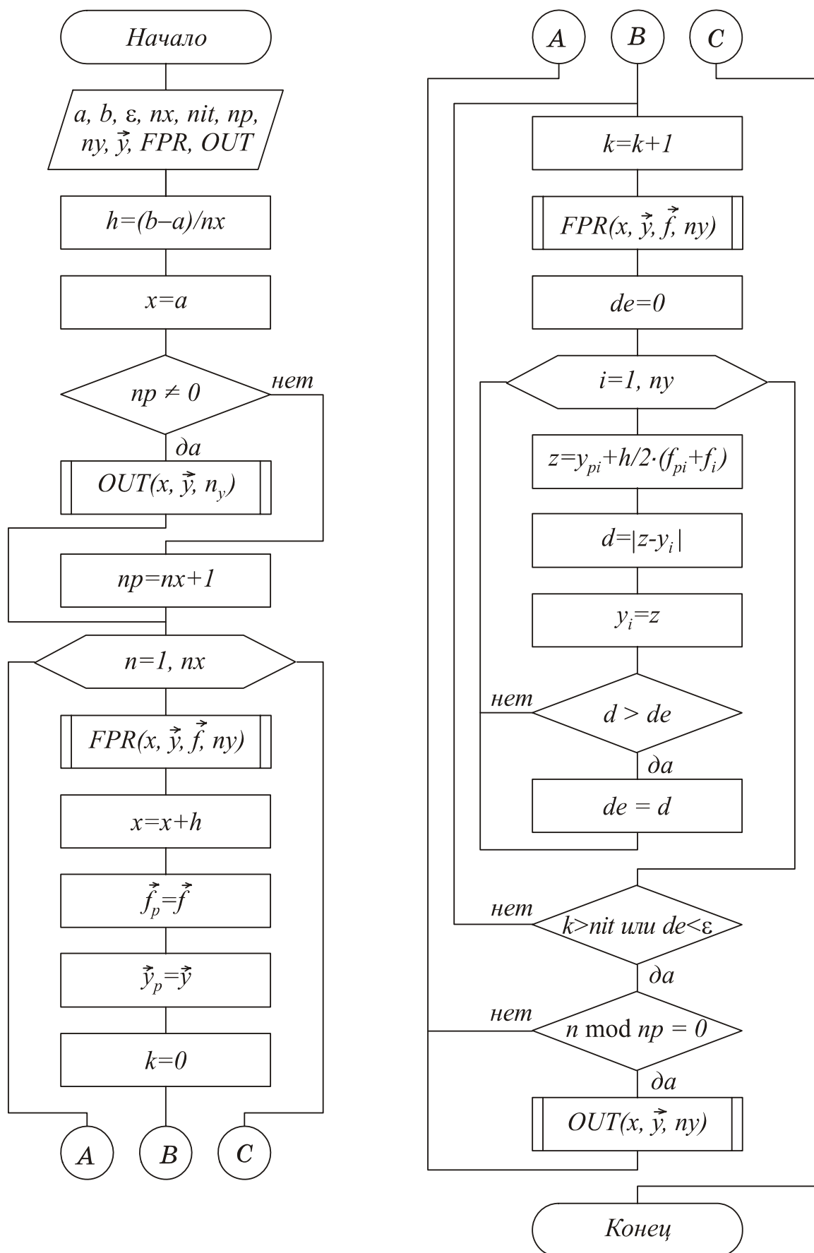
Рис. 19.2. Неявная схема 2-го порядка
