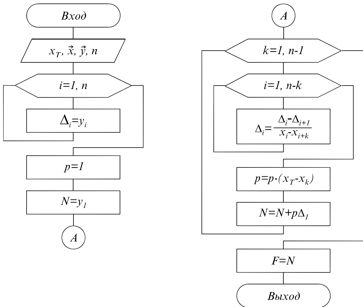
Рис. 16.1 Схема алгоритма расчета многочлена Ньютона
