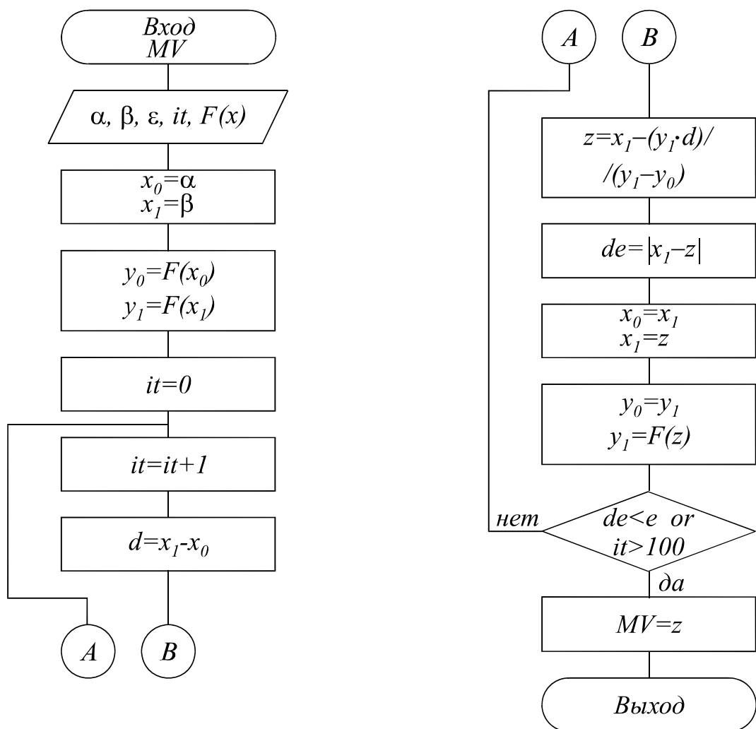
Рис. 17.2 Схема алгоритма метода Вегстейна
