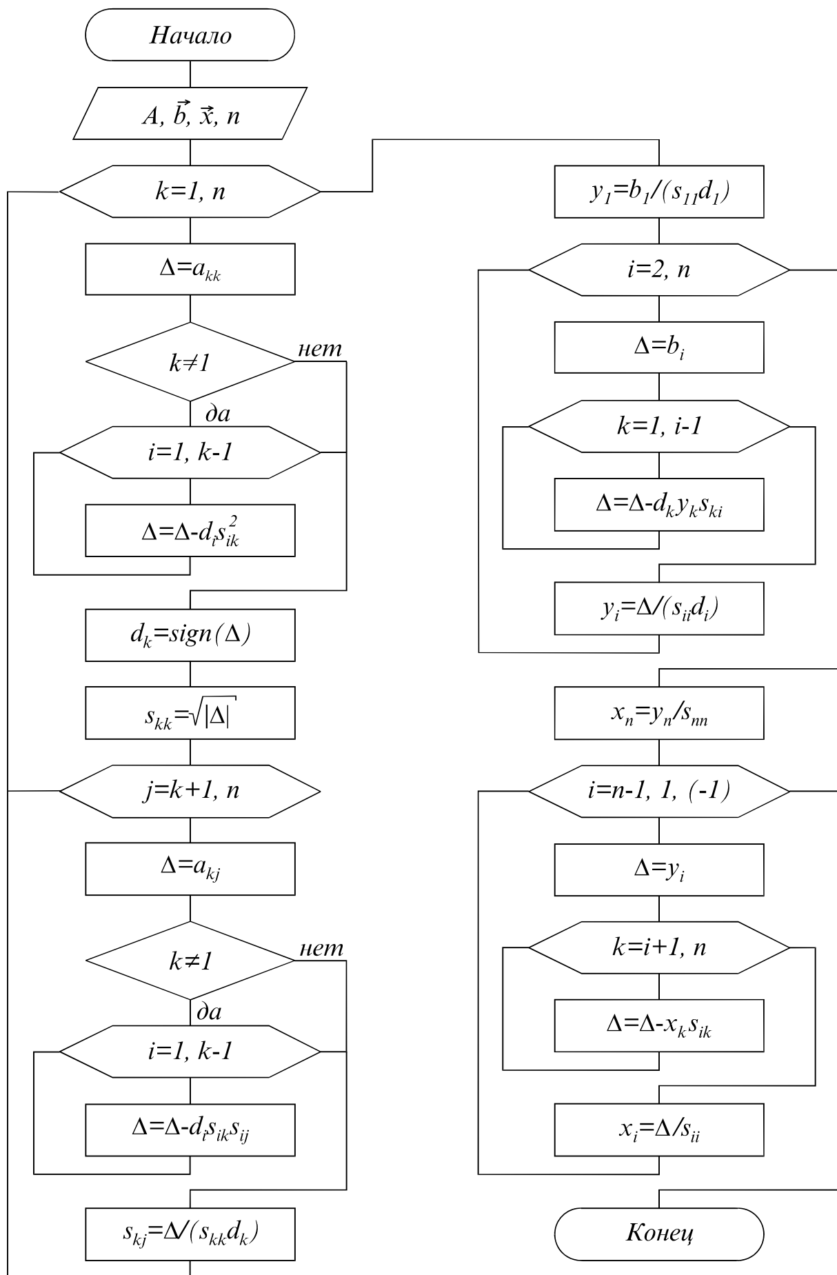
Рис. 15.2 Схема алгоритма метода квадратного корня
