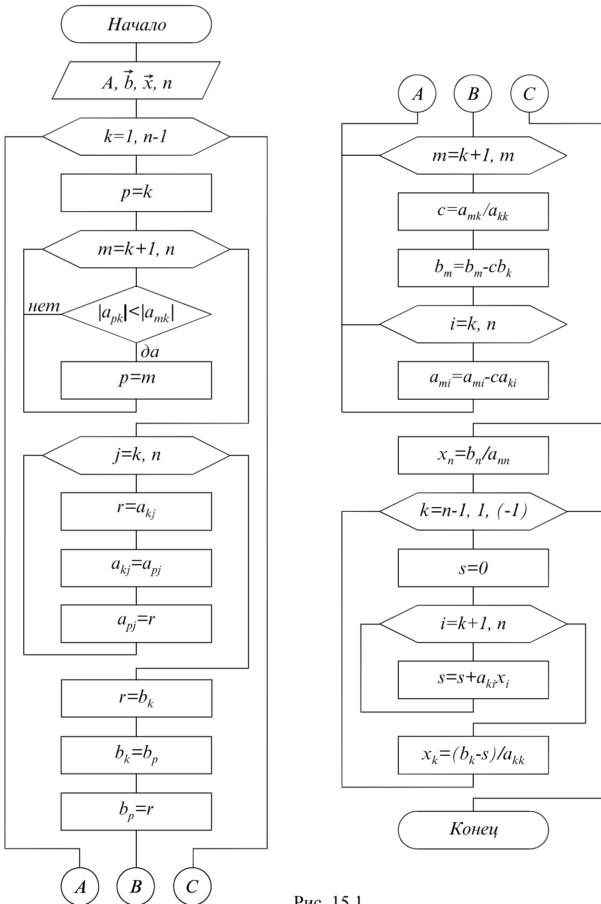
Рис. 15.1 Схема алгоритма метода Гаусса
