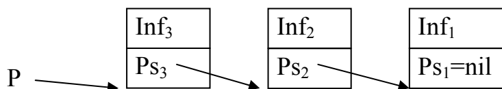
Рис.16.1. Структура стека
