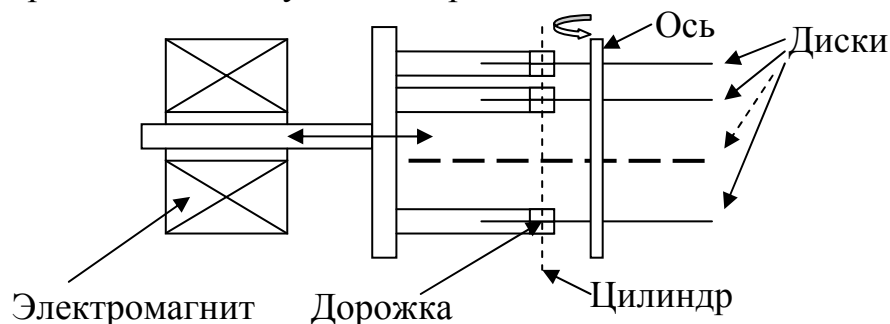
Рис.2.2. Схема дисководов
