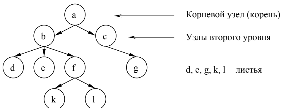
Рис.16.3. Структура дерева
