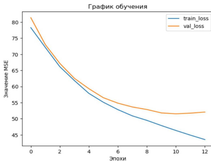
Рисунок 2. Динамика MSE предсказания длительности для DurationPredictor.
