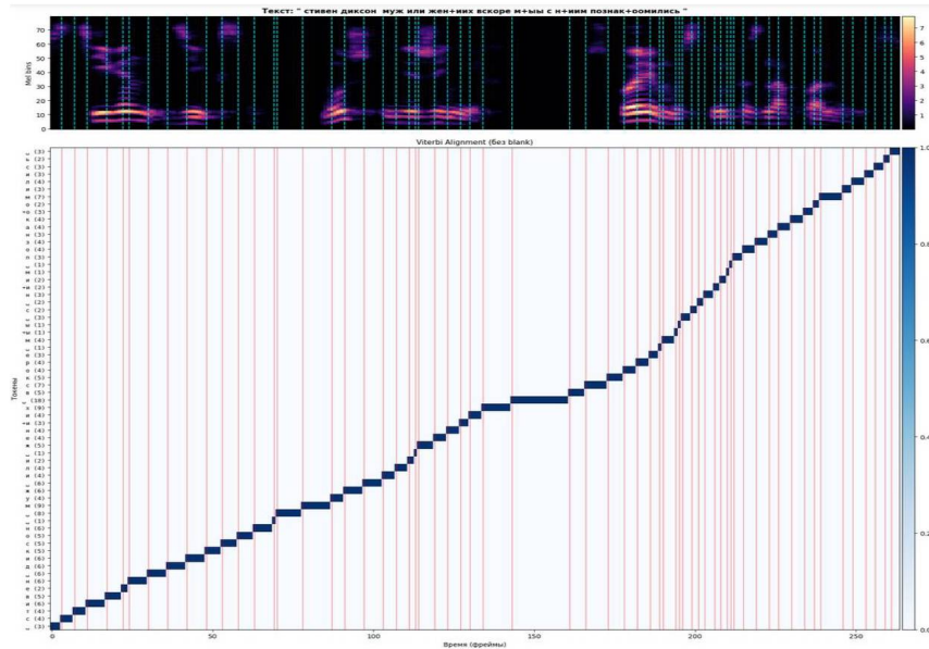
Рисунок 1. Alignment текста, полученный с помощью алгоритма Витерби.
