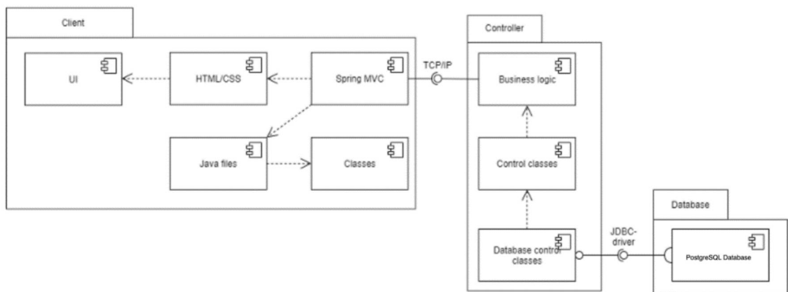
Рисунок 4. Диаграмма компонентов
