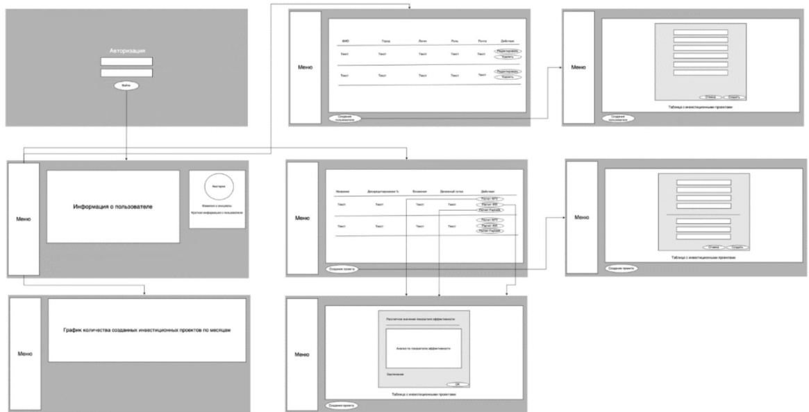
Рисунок 2. Карта экранов
