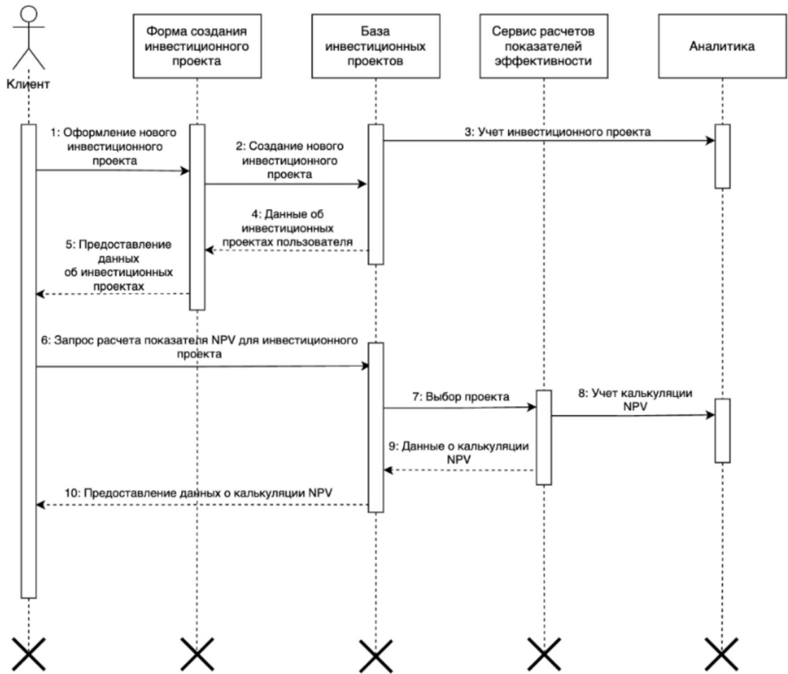
Рисунок 7. Диаграмма последовательности для вариантов использования «Создать инвестиционный проект» и «Расчитать показатель эффективности NPV»
