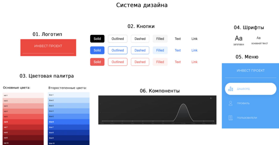
Рисунок 1. Система дизайна
