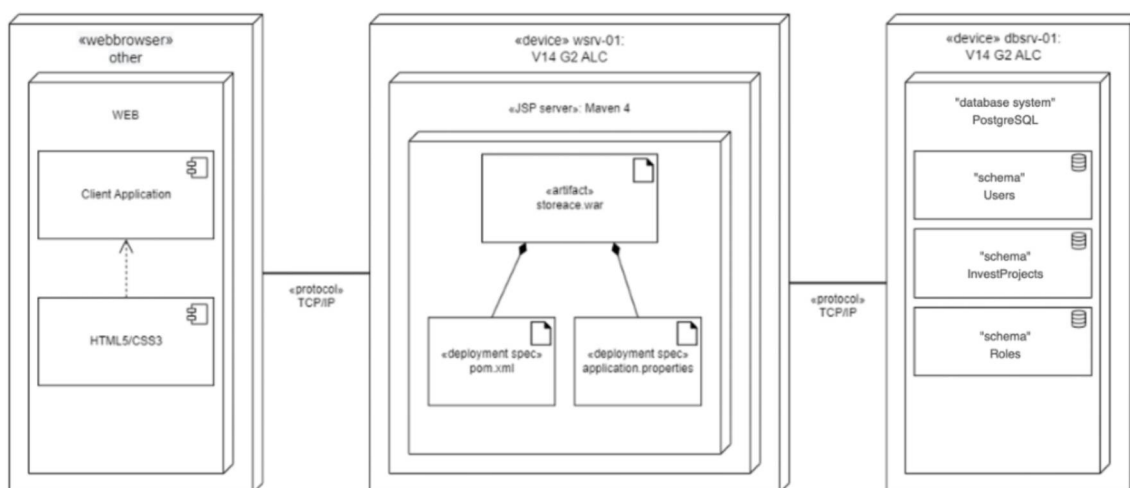
Рисунок 5. Диаграмма размещения
