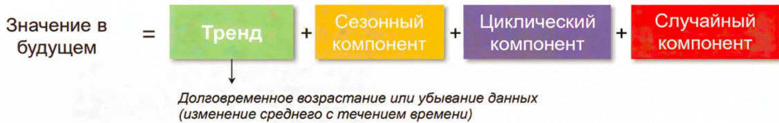
Рисунок 1. Классическая аддитивная модель временного ряда [13]
