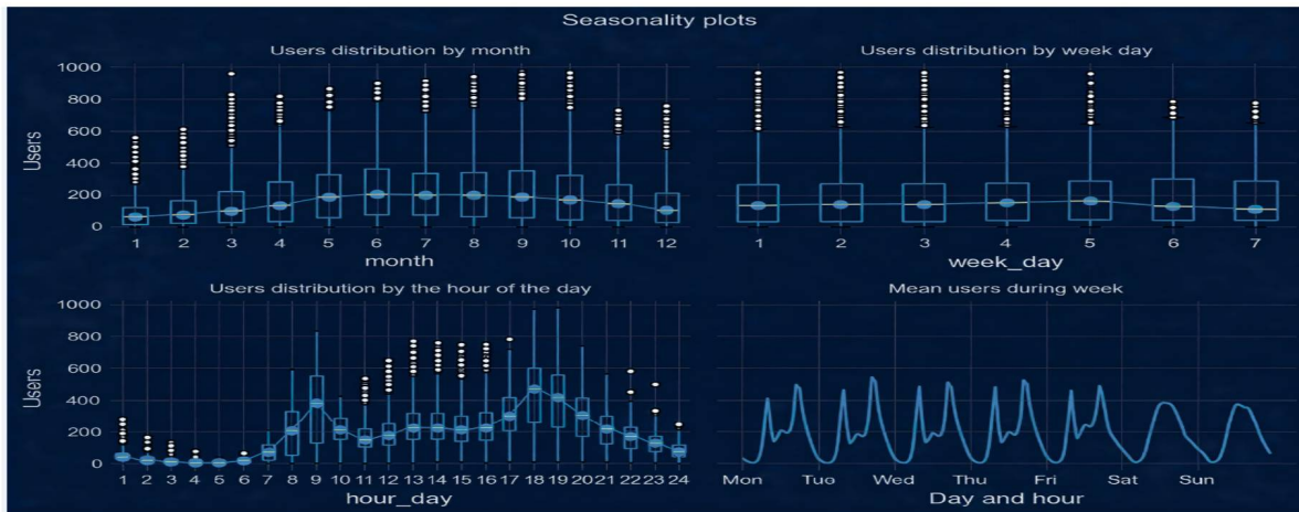
Рисунок 2. Пример сезонных графиков с данными для выявления сезонных закономерностей и трендов во временных рядах [7]
