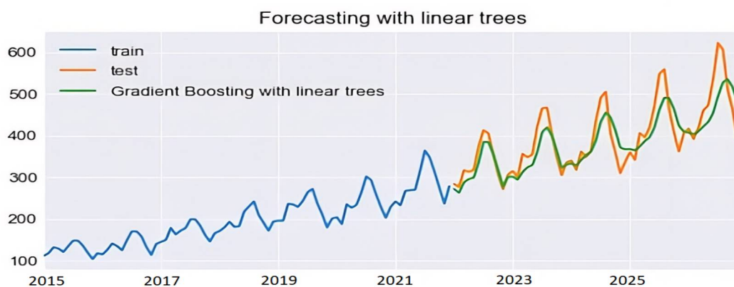
Рисунок 3. График, иллюстрирующий применение градиентного бустинга с линейными деревьями [7]
