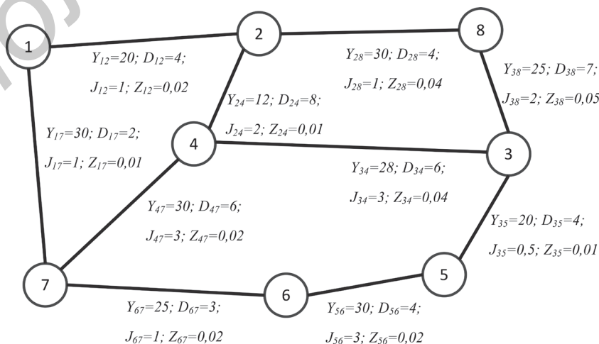
Рис. 1. Схема сети
